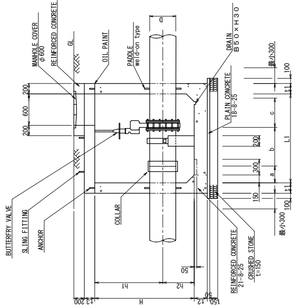
Longitudinal Section
