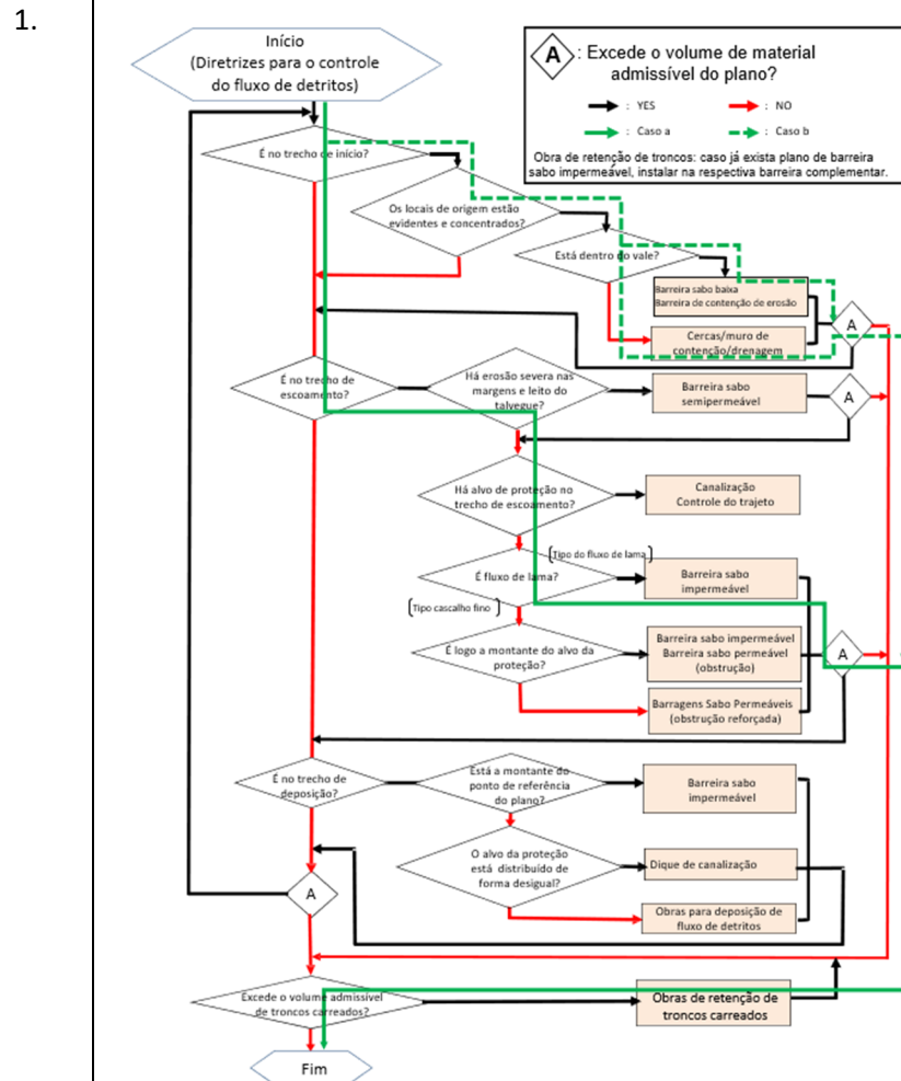
Figura 7.1 Seleção do tipo de solução de engenharia seguindo o fluxo grama
