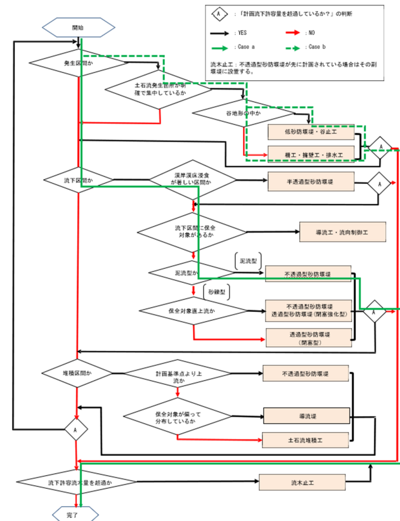
図 7.1 フローチャートによる工法選定
