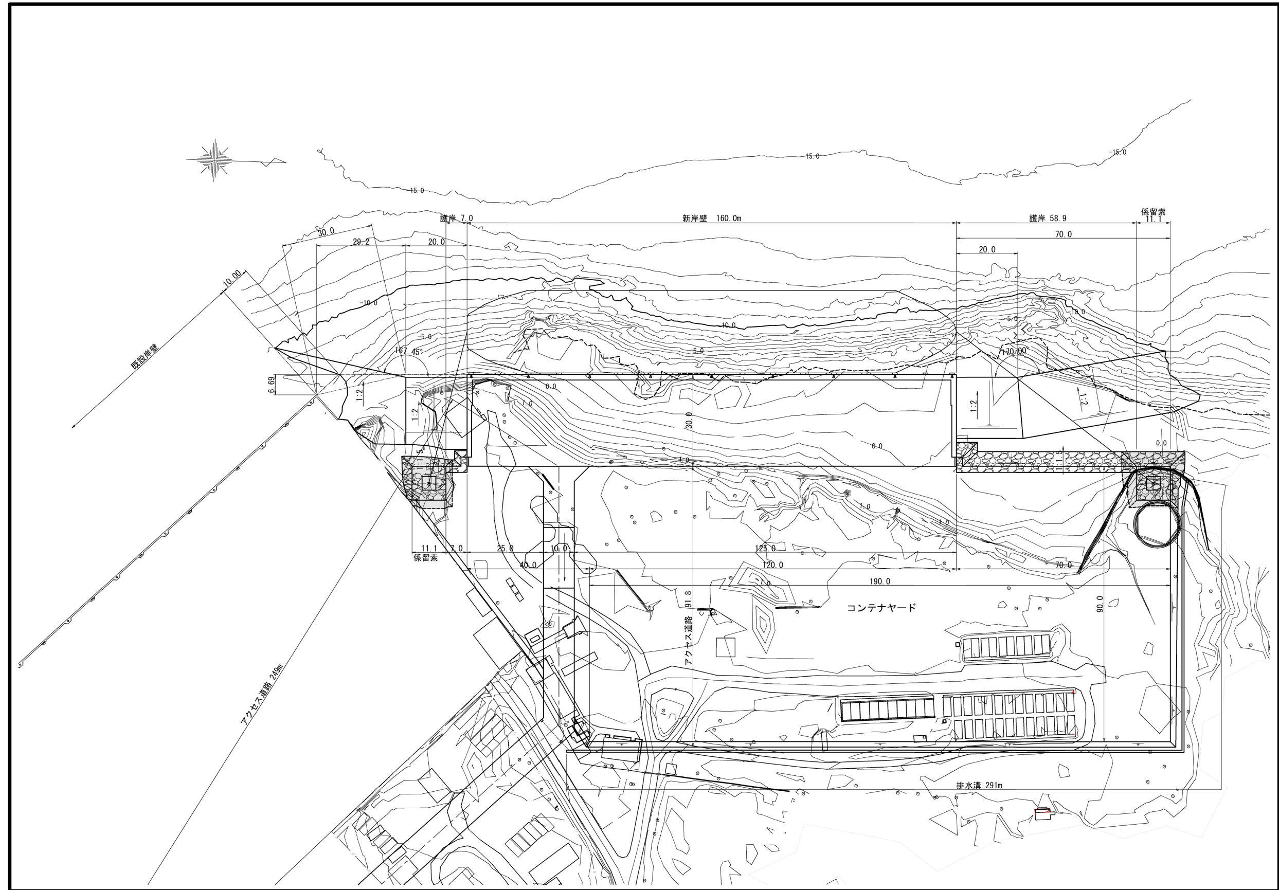
図 3-2-8 係留索工平面図
