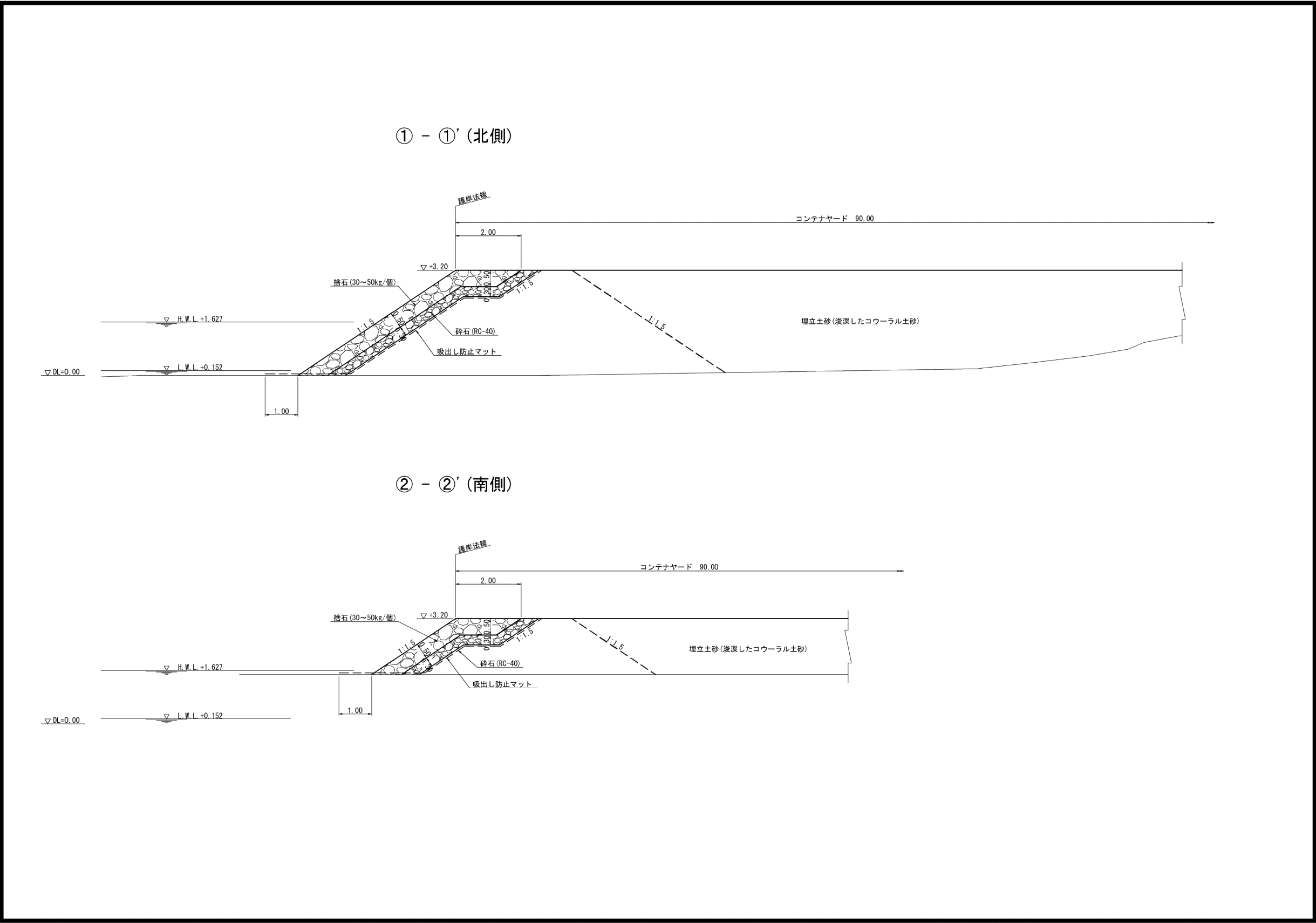
図 3-2-12 コンテナヤード護岸標準断面図
