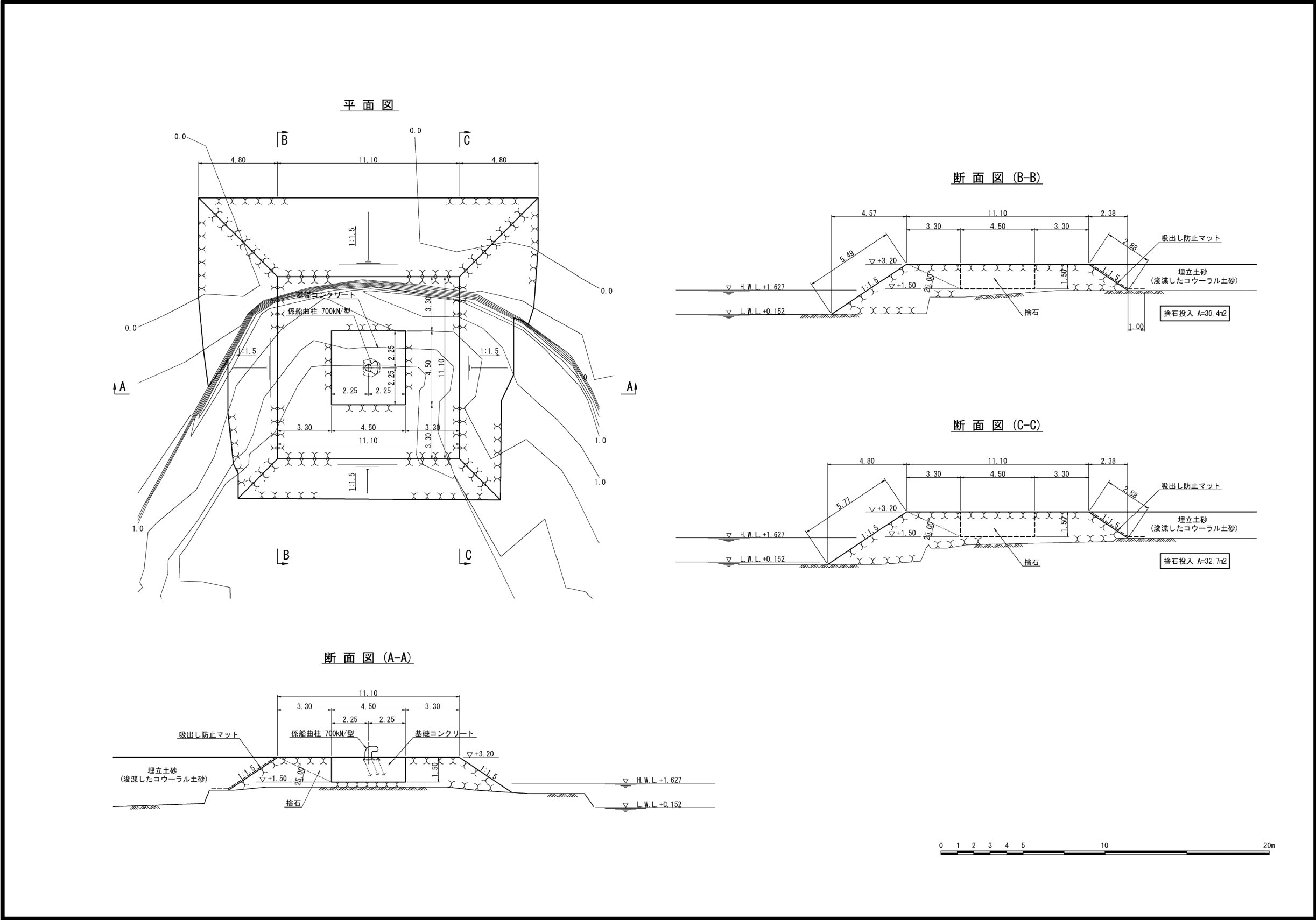
図 3-2-9 係留索工図（北側）
