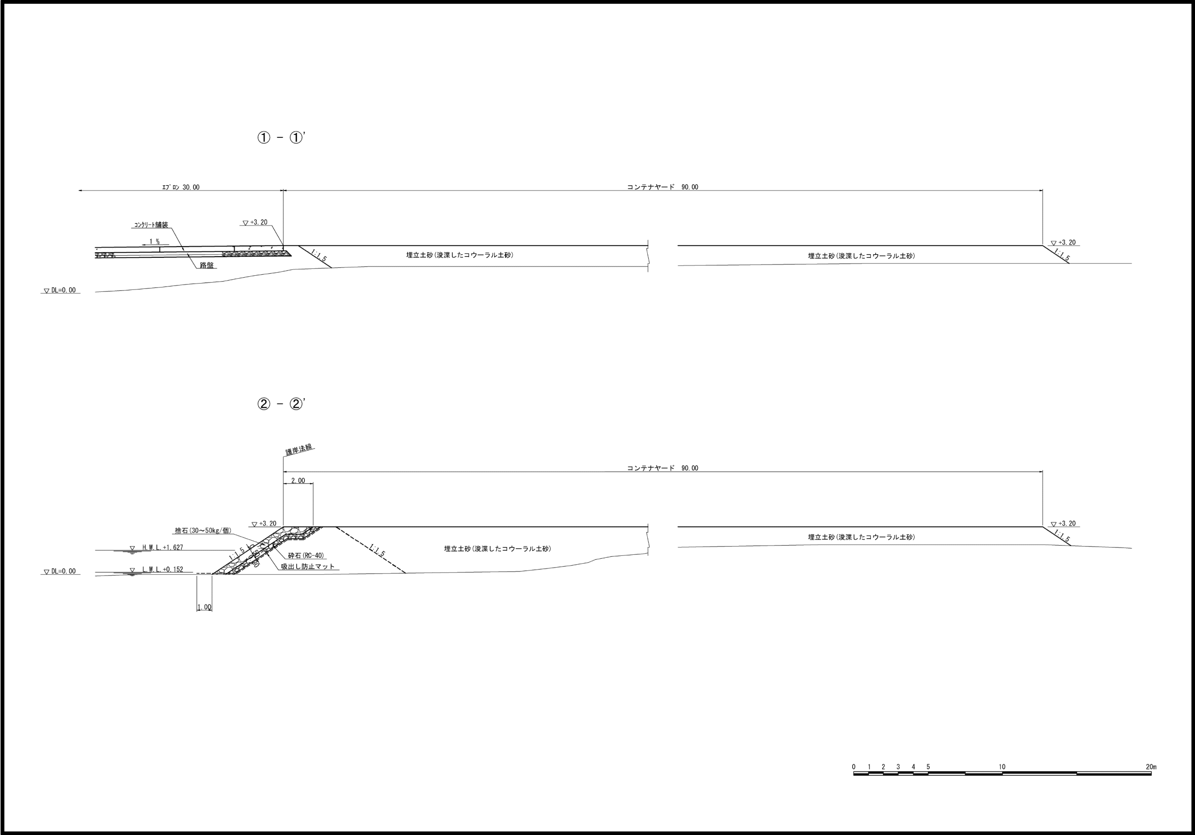
図 3-2-14 コンテナヤード標準断面図
