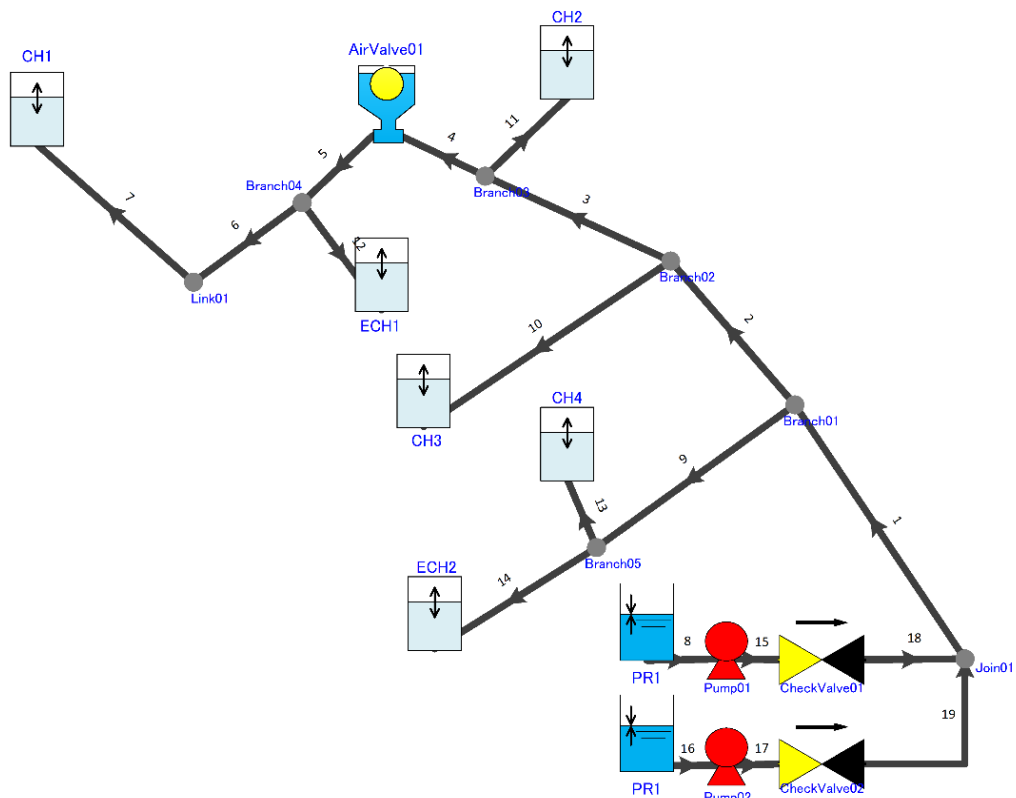
図 2 : 計算モデル
