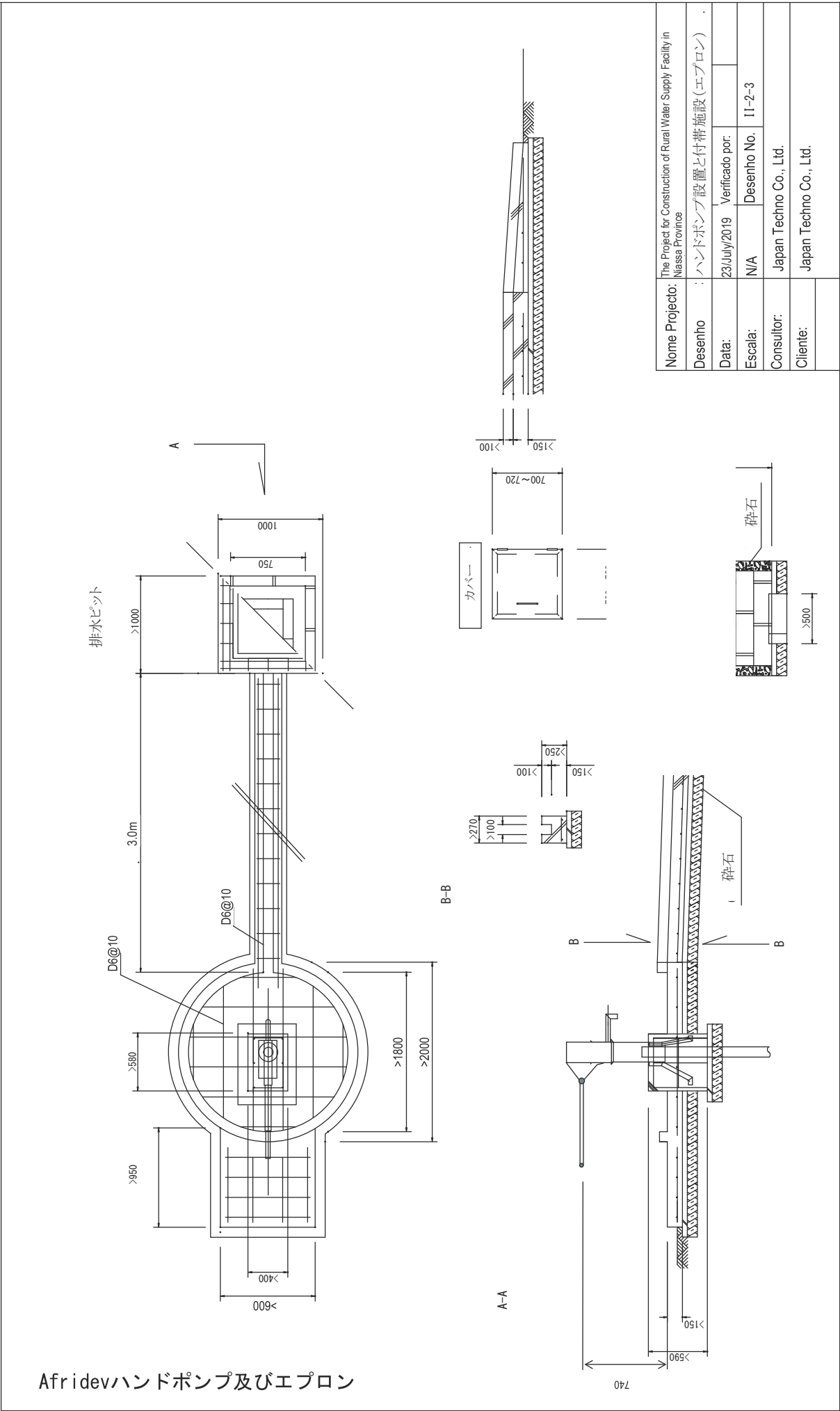
図-5.b ハンドポンプ付き深井戸給水施設 (付帯施設-エプロン) (標準図)
