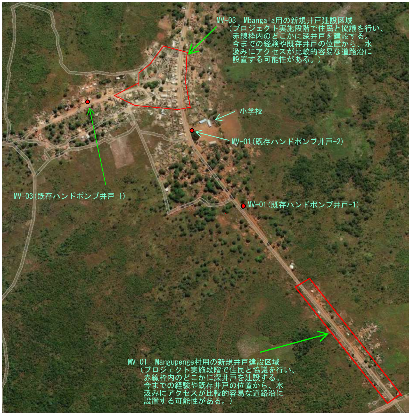
図-1 既存ハンドポンプ付深井戸位置および新規ハンドポンプ付深井戸建設予定区域 (対象サイト： MV-01 Mangupenge、およびMV-03 Mbangala)
