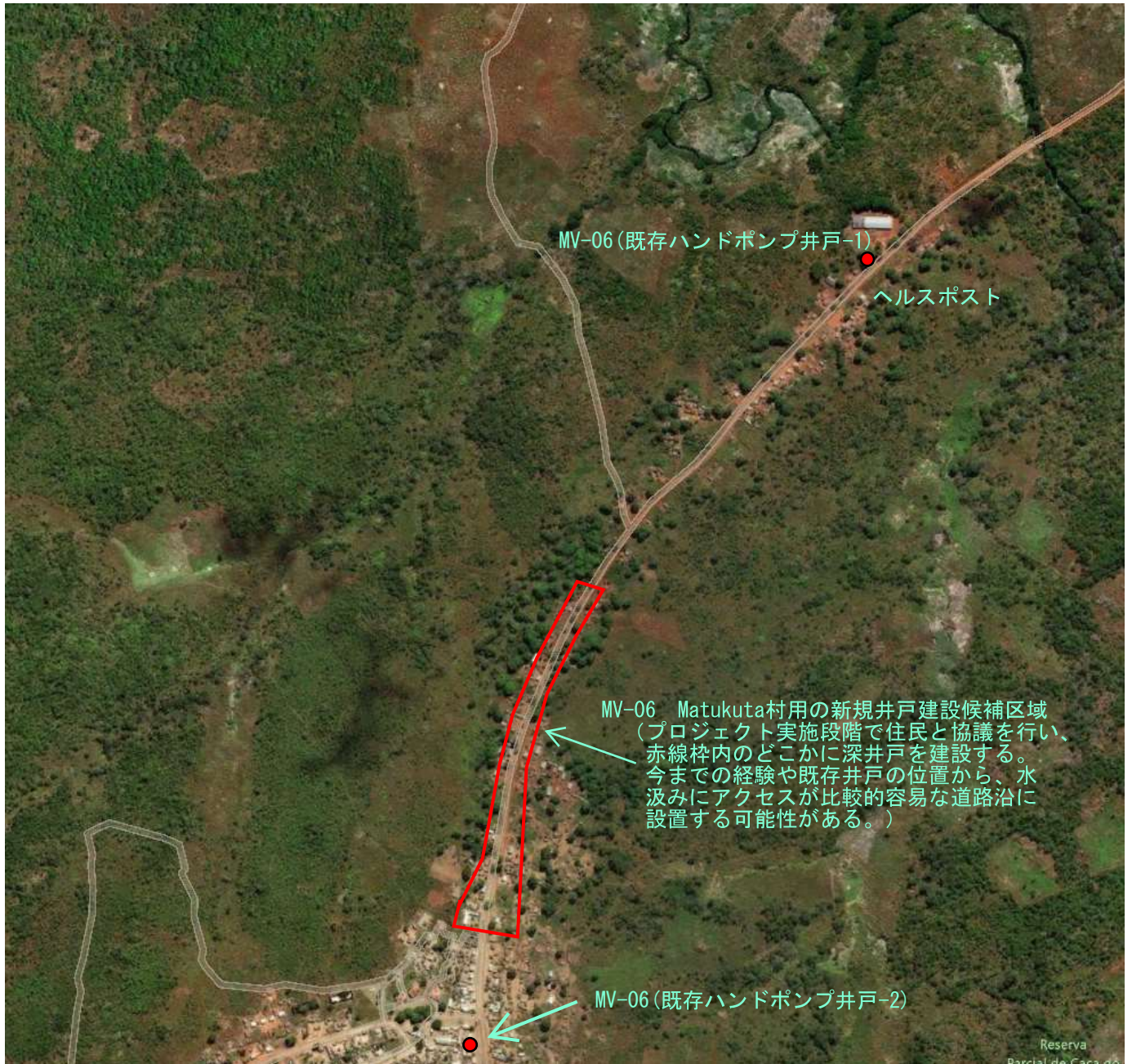
図-2 既存ハンドポンプ付深井戸位置および新規ハンドポンプ付深井戸建設予定区域 (対象サイト: MV-06 Matukuta)
