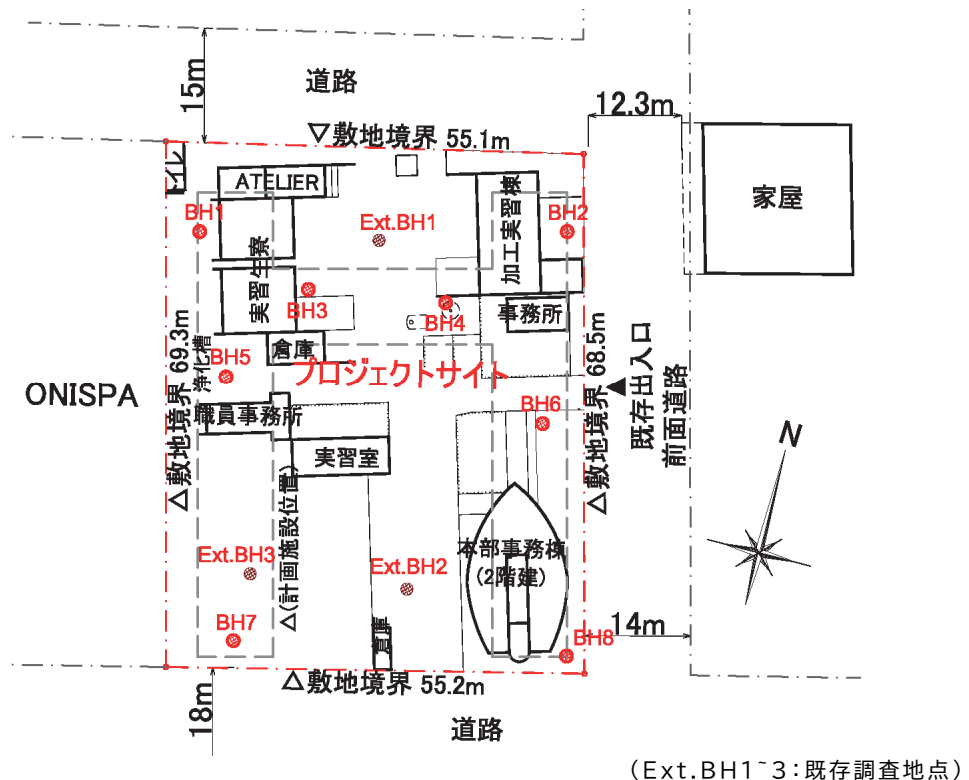
図 3-34:実施設計時の地盤調査計画位置
