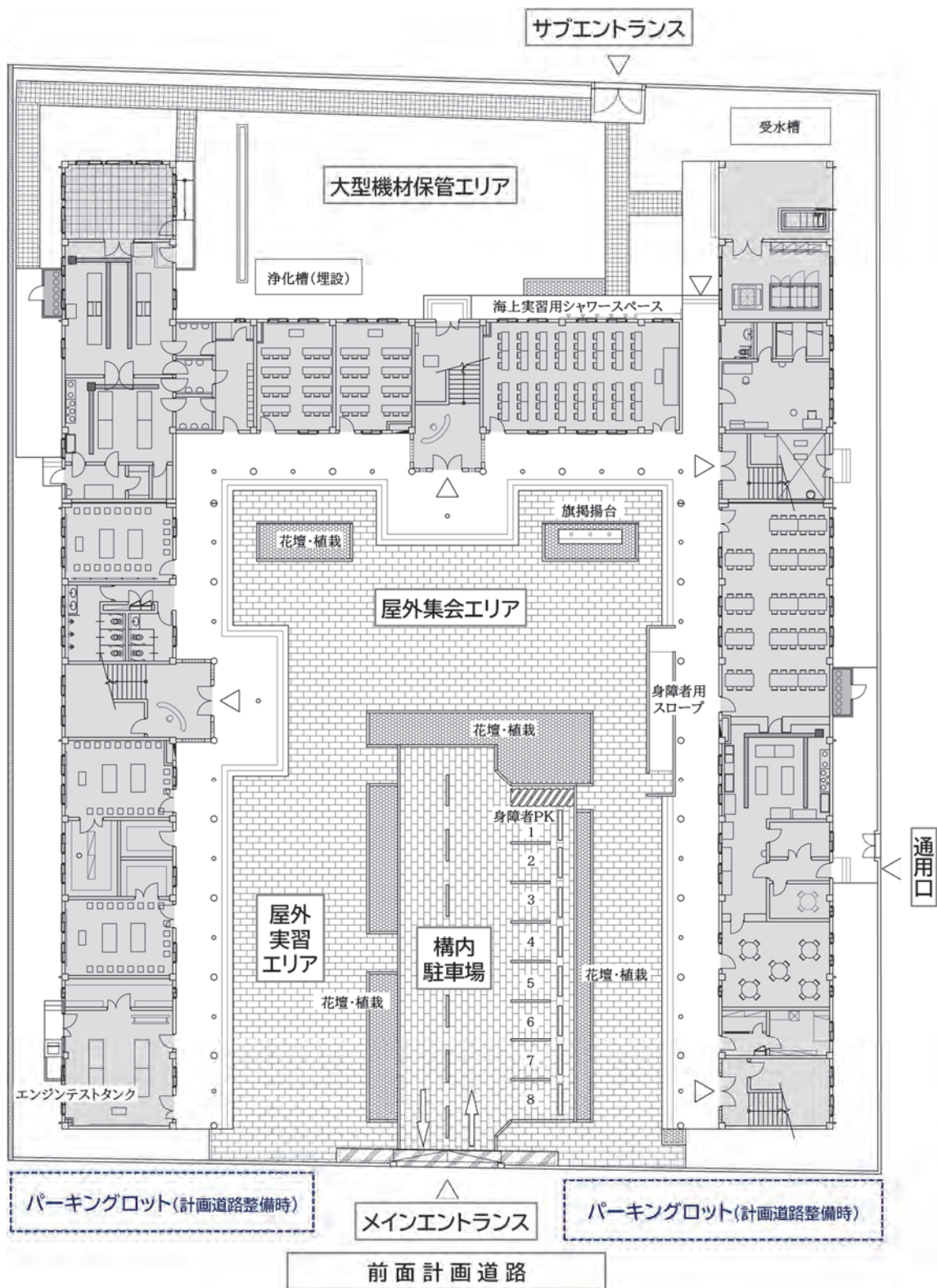
図 3-8: CQFMP 施設の配置計画案
