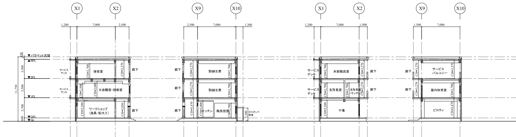
A-A' 断面図
