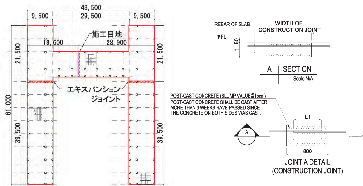
図 3-33:エキスパンションジョイント・施工目地
