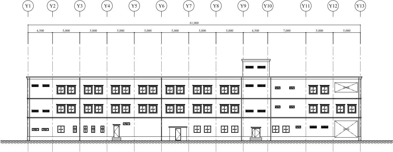
東側立面图
