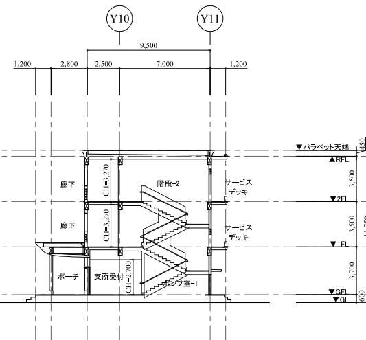
G-G' 断面図
