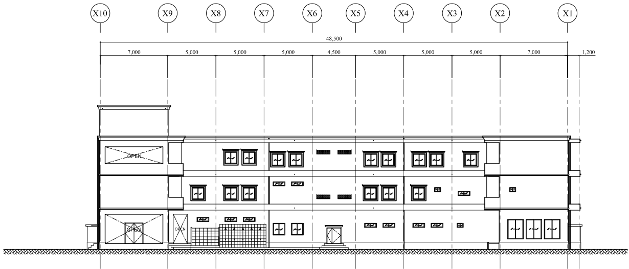
北側立面图
