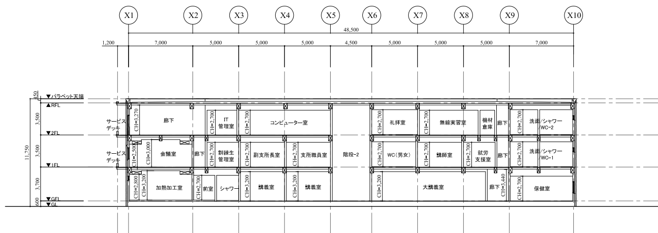
B-B' 断面図
