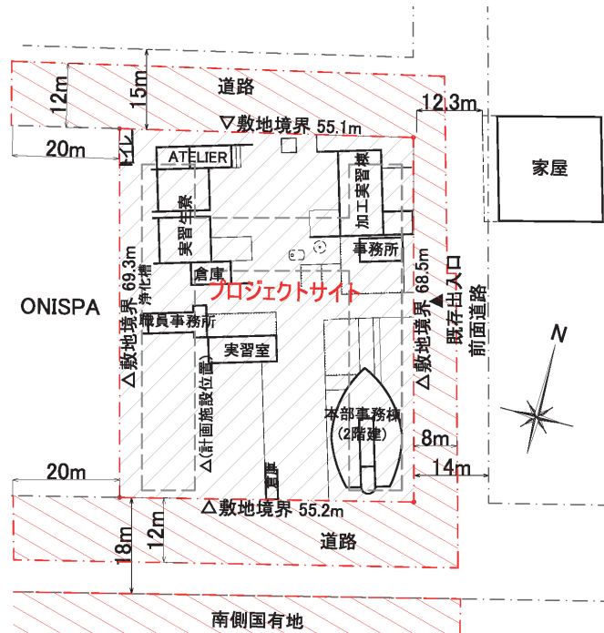
図 3-35 : CQFMP ノアクショット敷地(プロジェクトサイト)及び仮設ヤード
