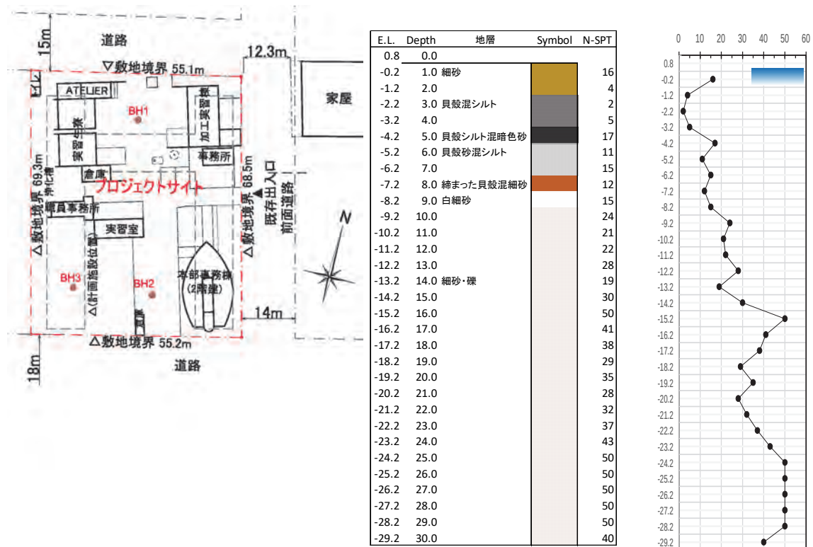
図 3-32:地盤調査結果(BH3 標準貫入試験結果)
