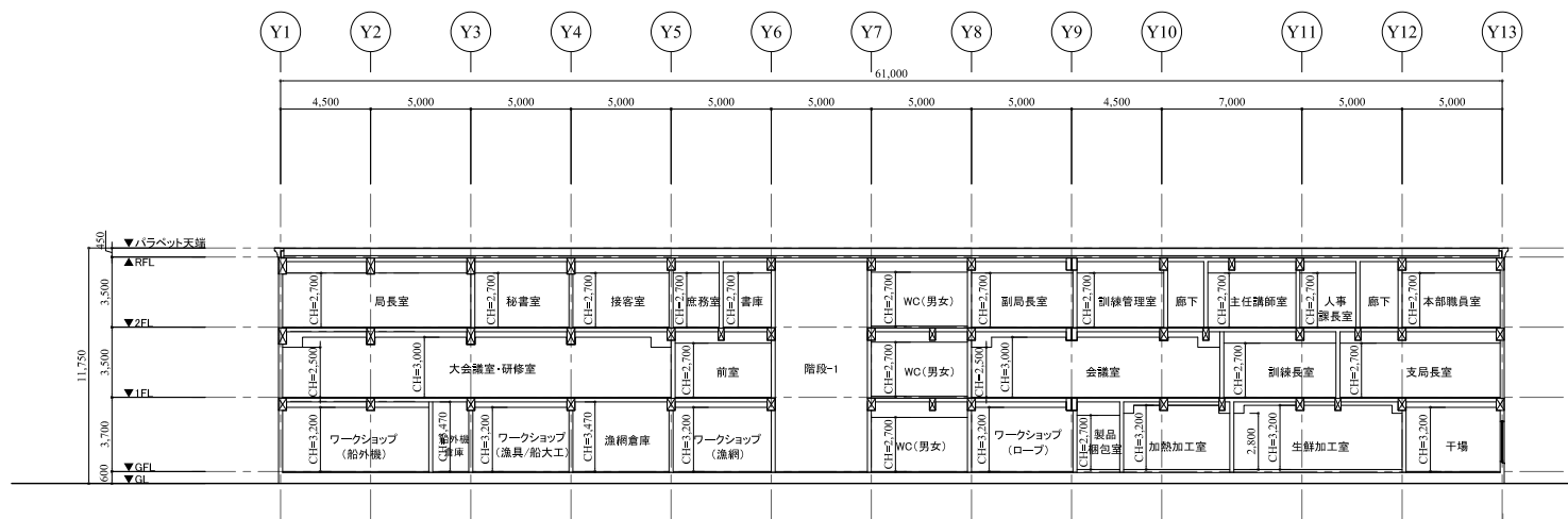
D-D' 断面図
