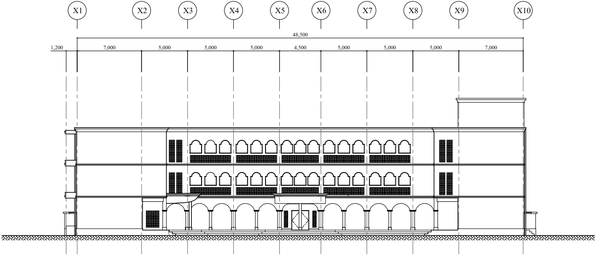
南側立面图
