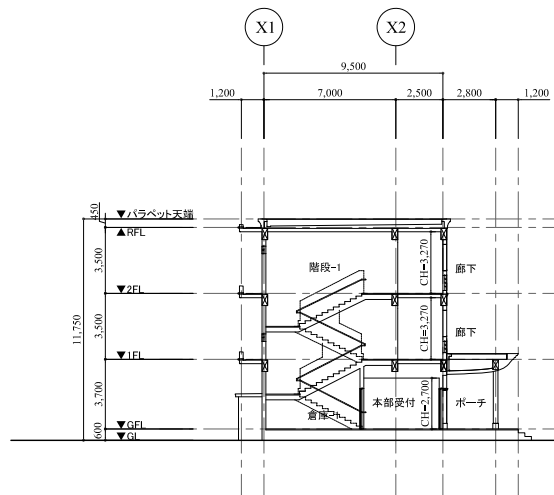
E-E' 断面図
