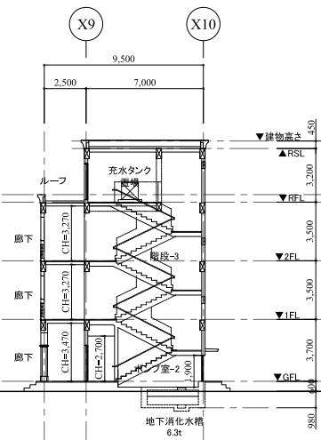
F-F' 断面図
