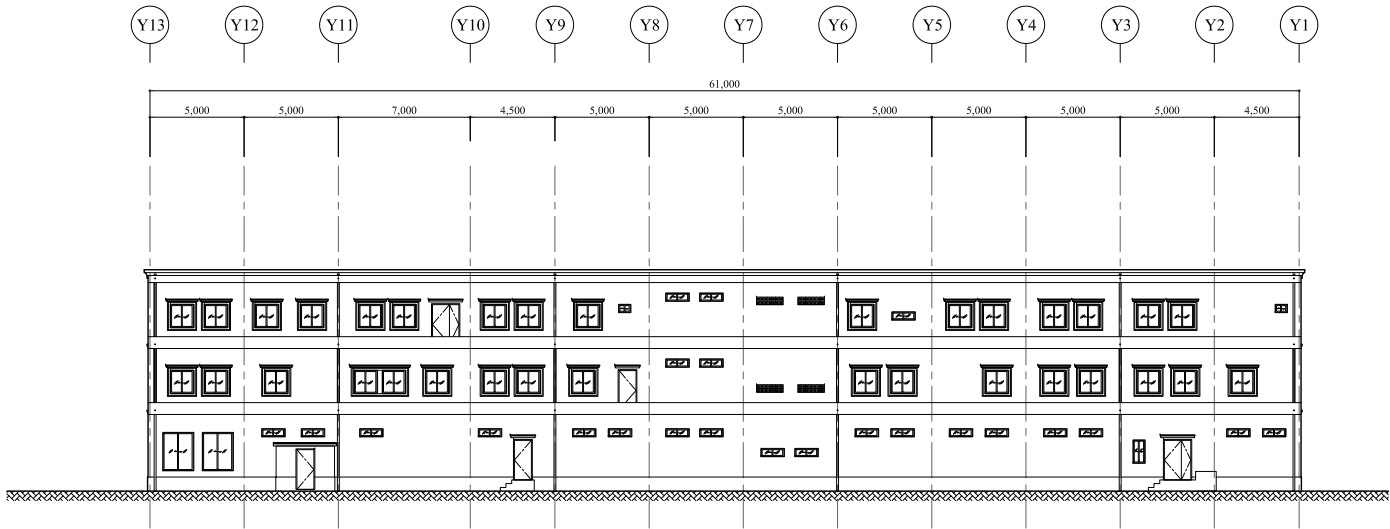
西側立面图
