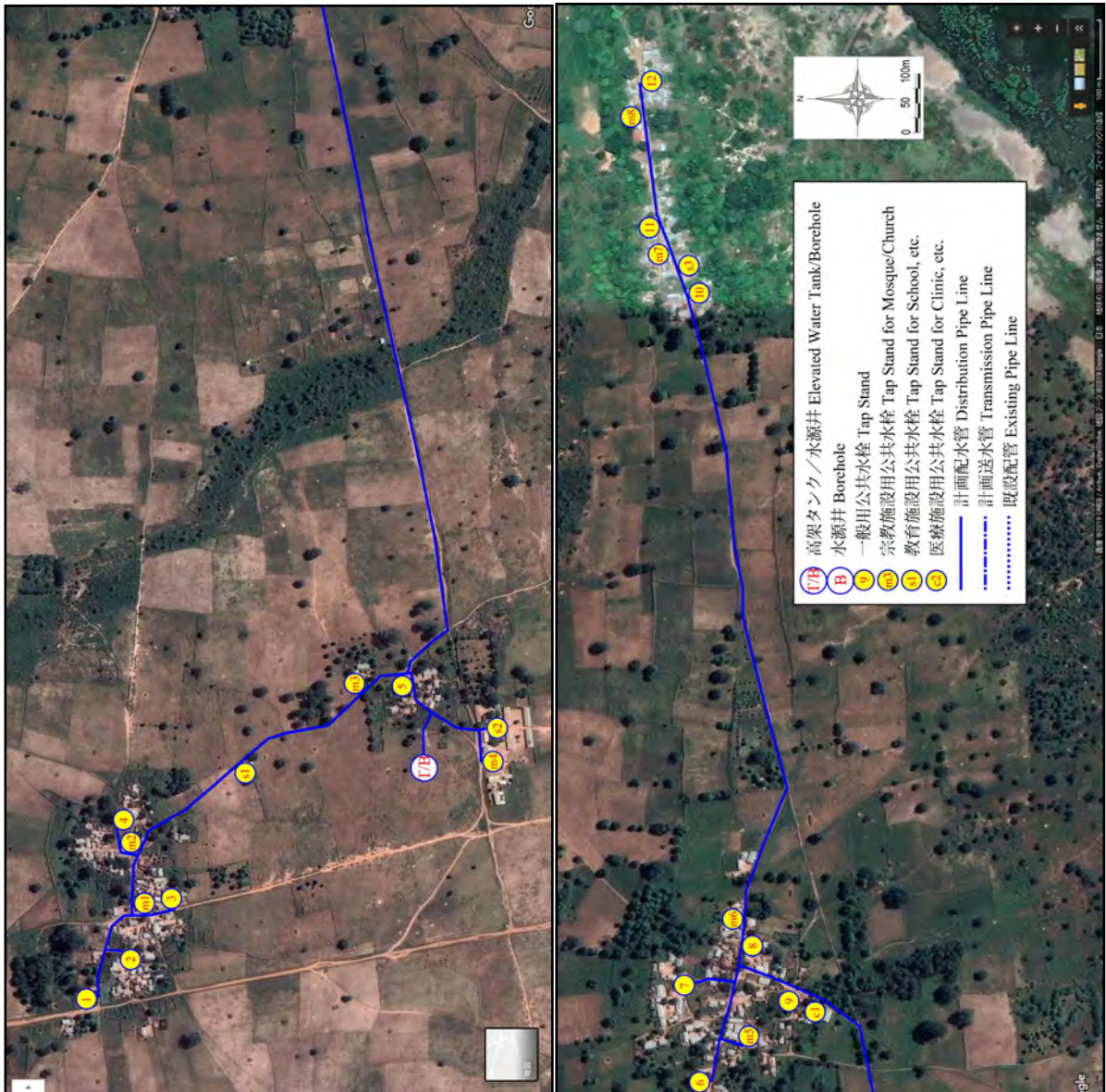
サイト平面図：N-07
