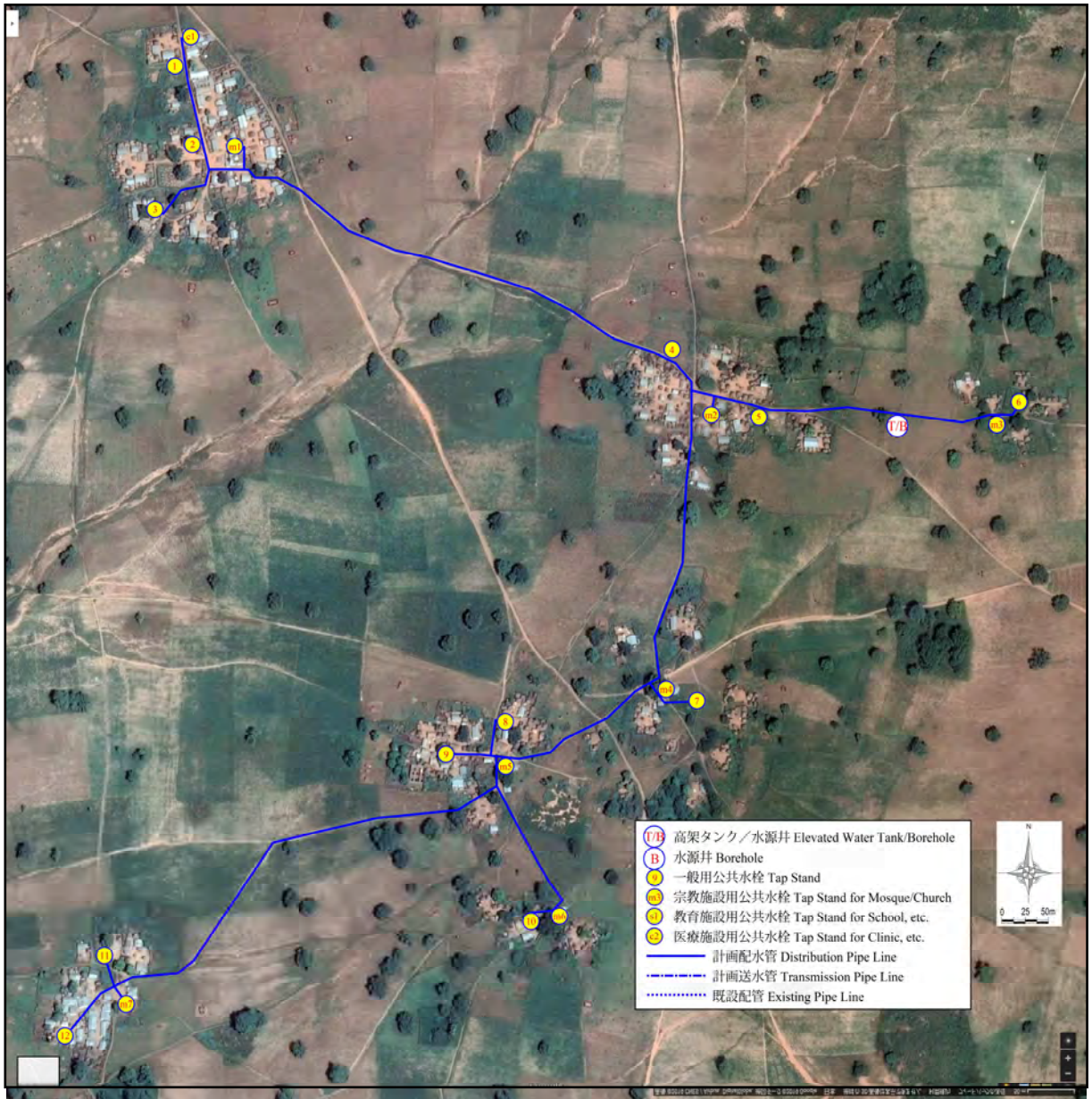
サイト平面図：N-22
