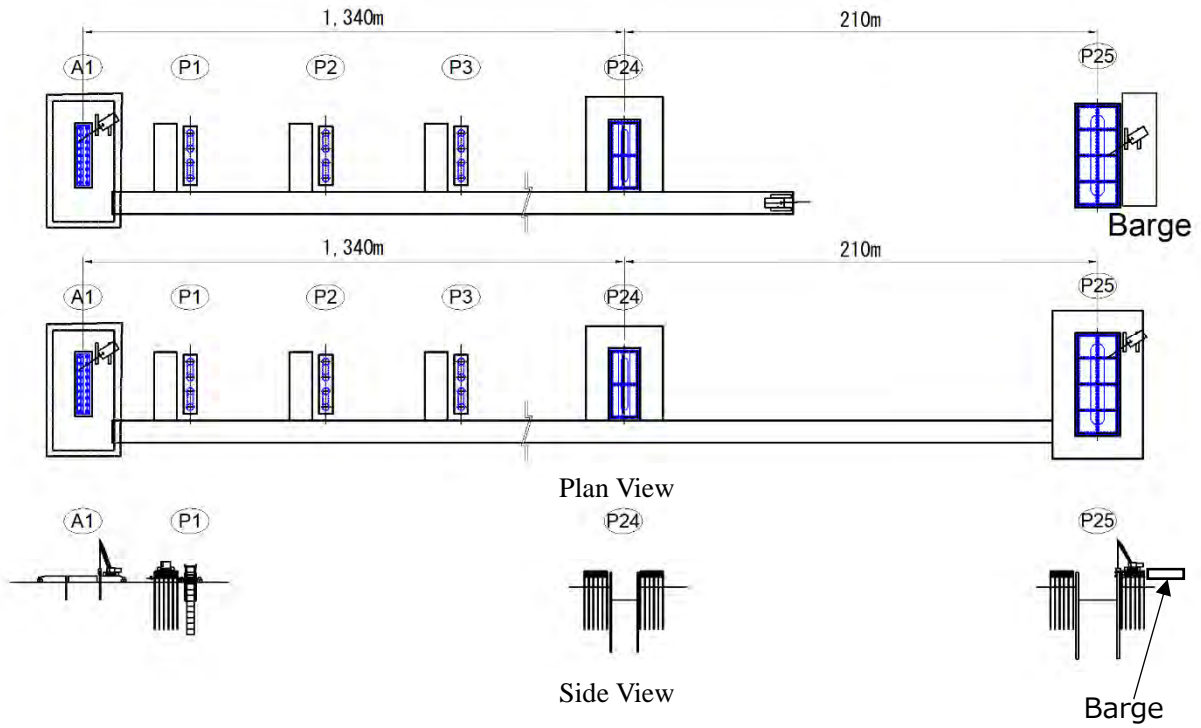
図11-3-1. 左岸側仮橋
