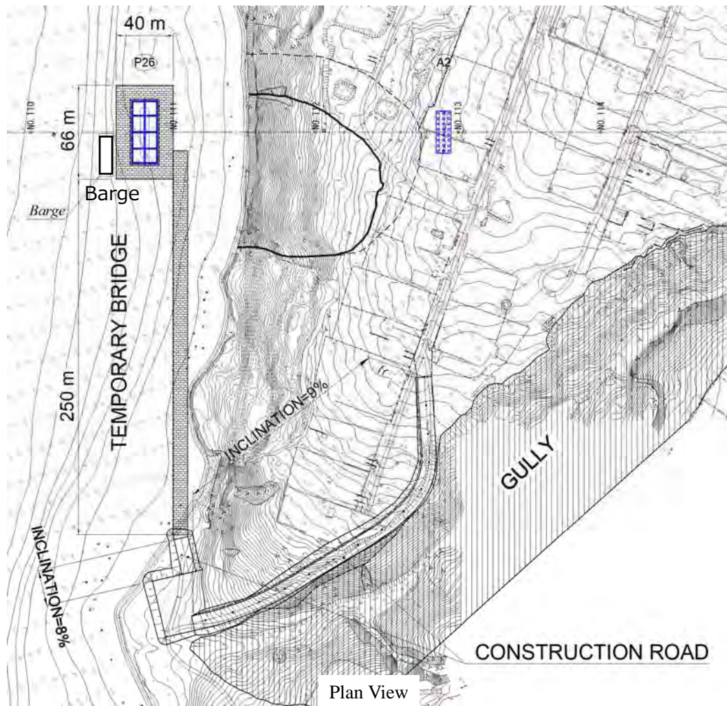
図 11-3-2. 右岸側仮橋および仮設道路
