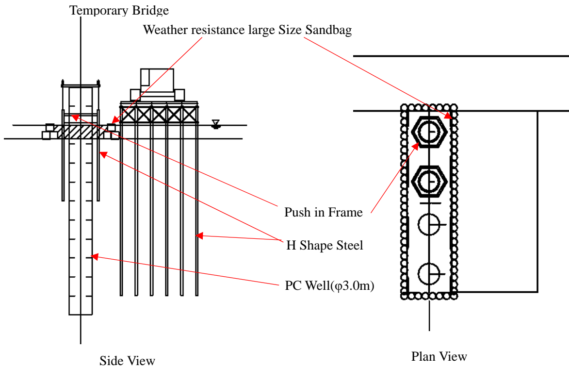
図 11-2-29.P1-P20 仮設参考図
