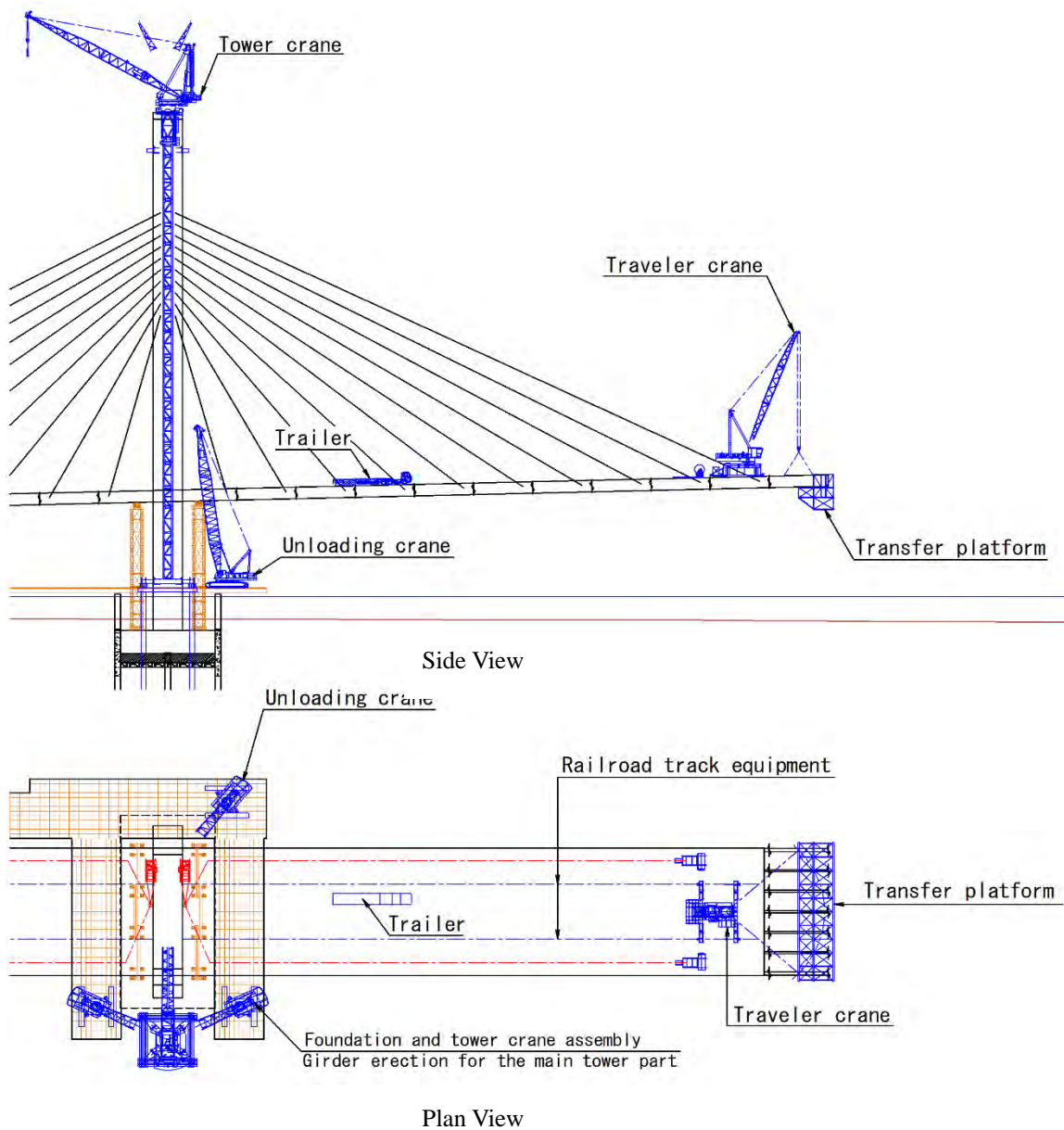
図12-2-12-2-1. トラバークレーン及び運搬台車設備のイメージ
