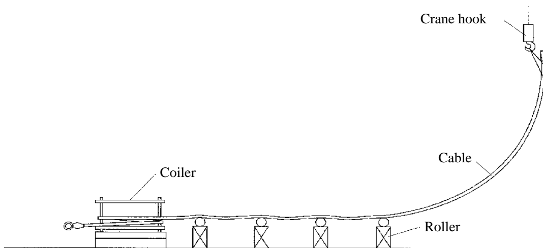
図 12-2-2. ケーブル展開作業のイメージ
