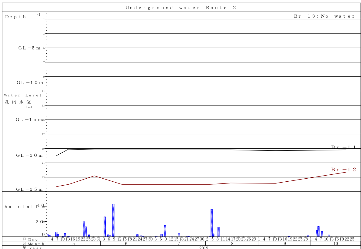
図9-8-8. 観測グラフ (ルート2: 伸縮計, 地下水位)
