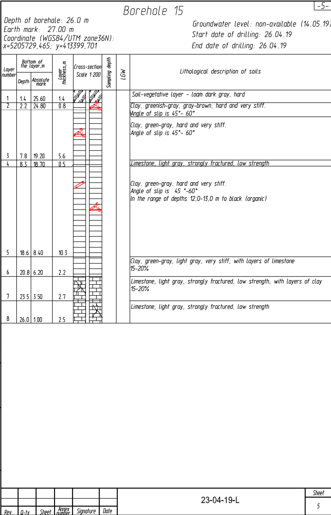
図9-8-18. ボーリング柱状図 (Br-15)
