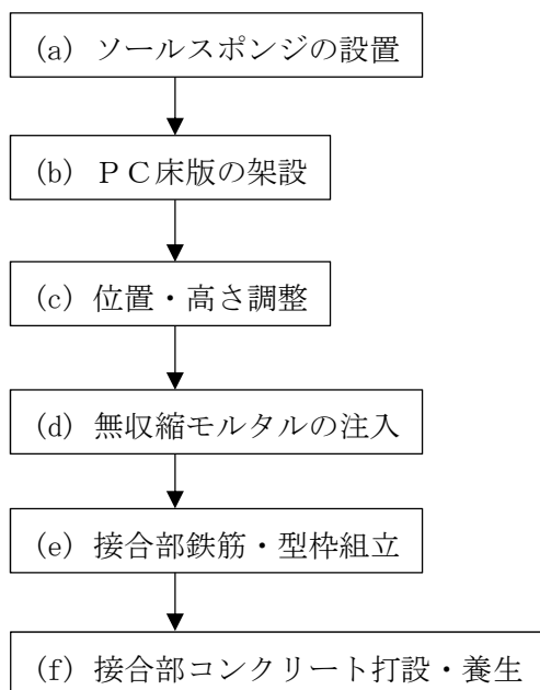
図 11-2-20. PC 床版施工フロー
