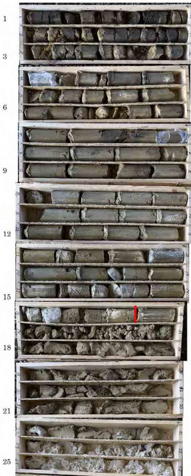
図 9-8-2. コア写真 (Br-11)
