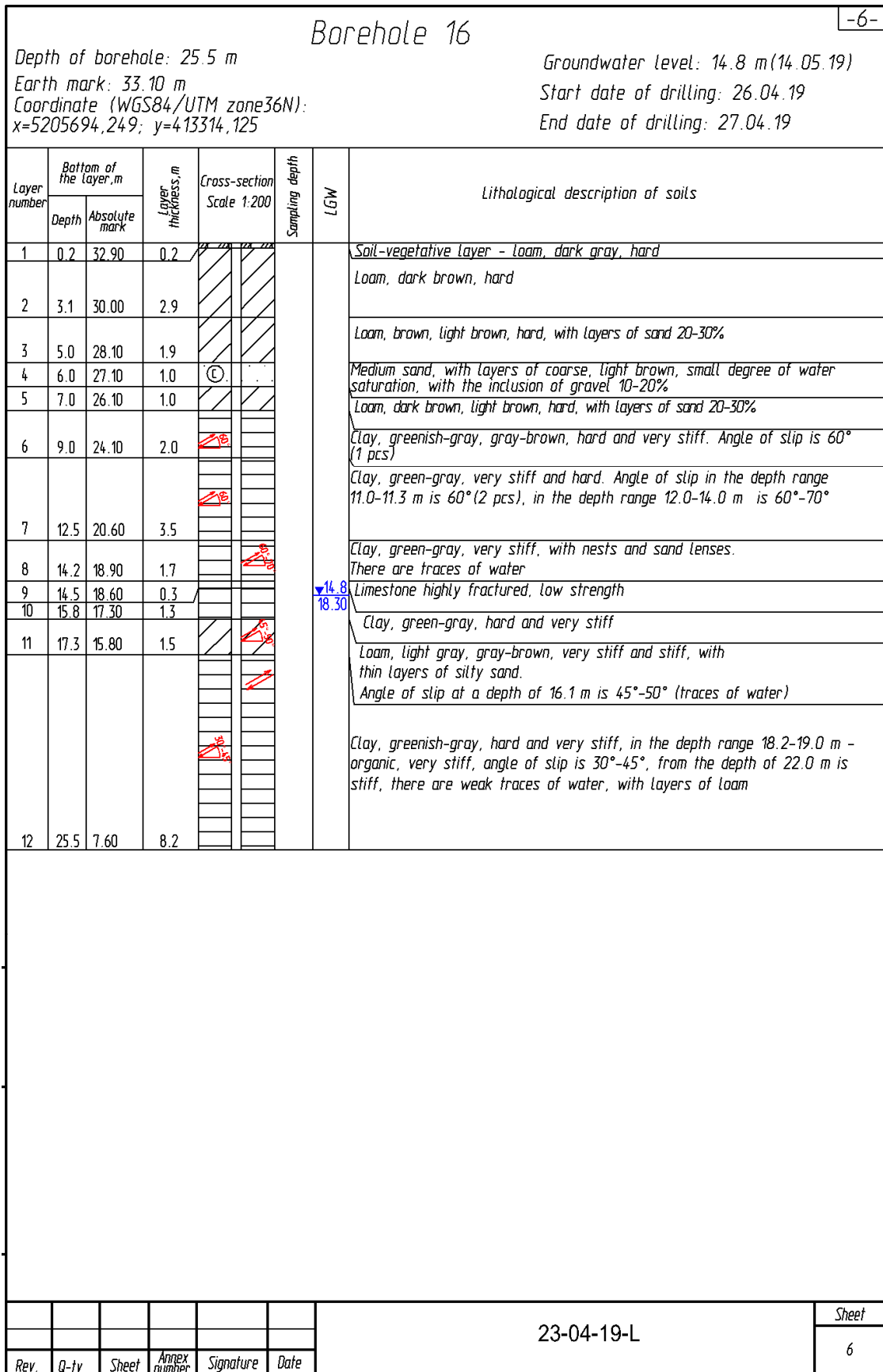
図9-8-20. ボーリング柱状図 (Br-16)
