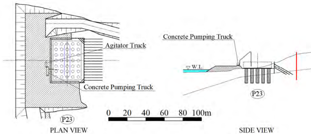
図11-2-16.フーチングの施工（コンクリート打設）参考図
