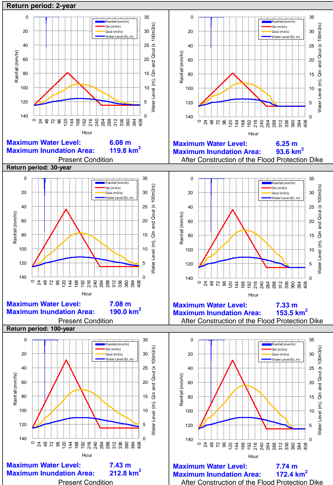
図 3.3.2 単純貯留モデルを用いた洪水シミュレーション結果
