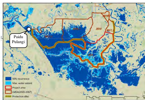
図 3.1.3 湛水範囲と年再帰の傾向 (1984-2014)
