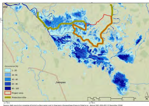
図 3.1.2 Liguasan 湿地水域の長期的変動 (1984-2014)
