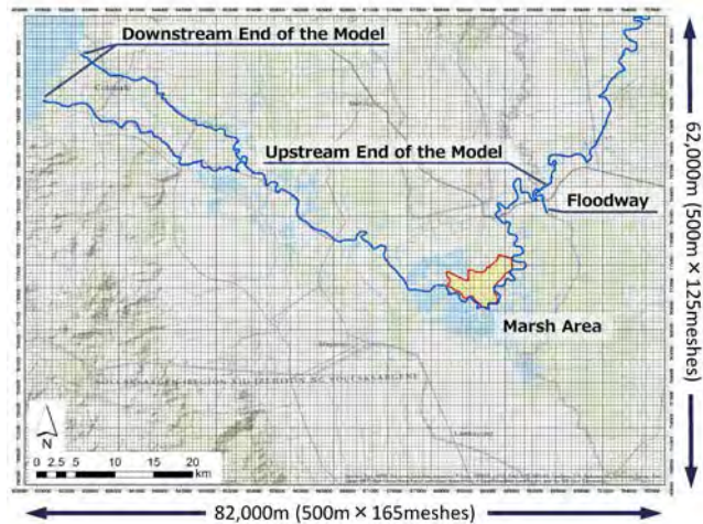
図 3.4.1 洪水氾濫範囲把握モデル
