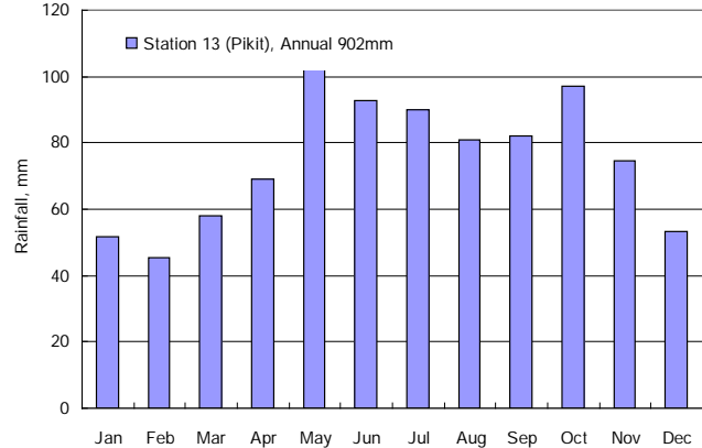
図 2.1.4 月別降水量 (Pikit)
