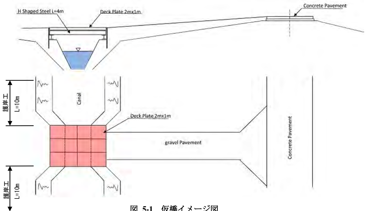
図 5-1 仮橋イメージ図
