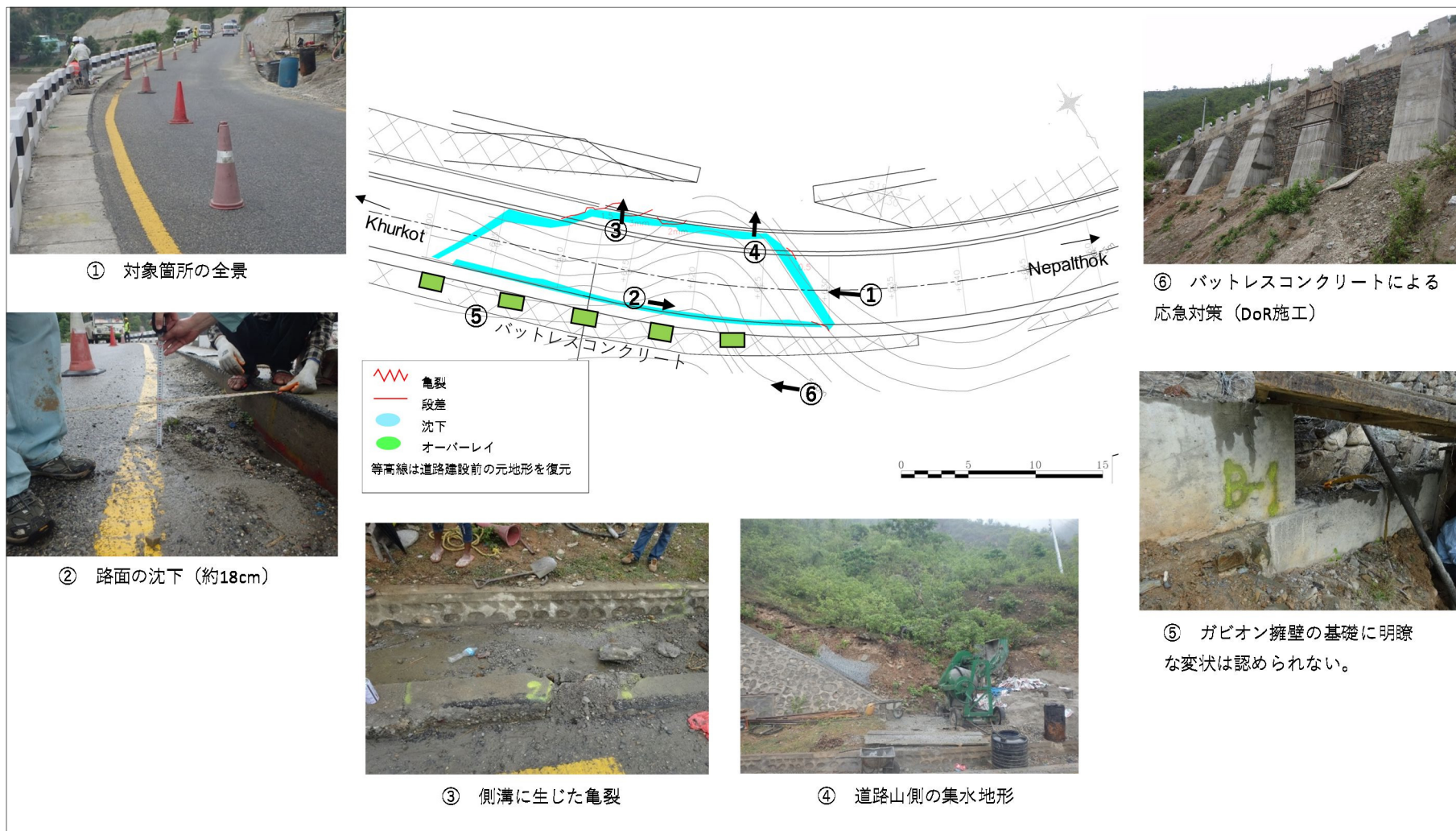
図 2.1.7 第三工区 Sta. 11+620 の周辺状況（Non-Scale）
