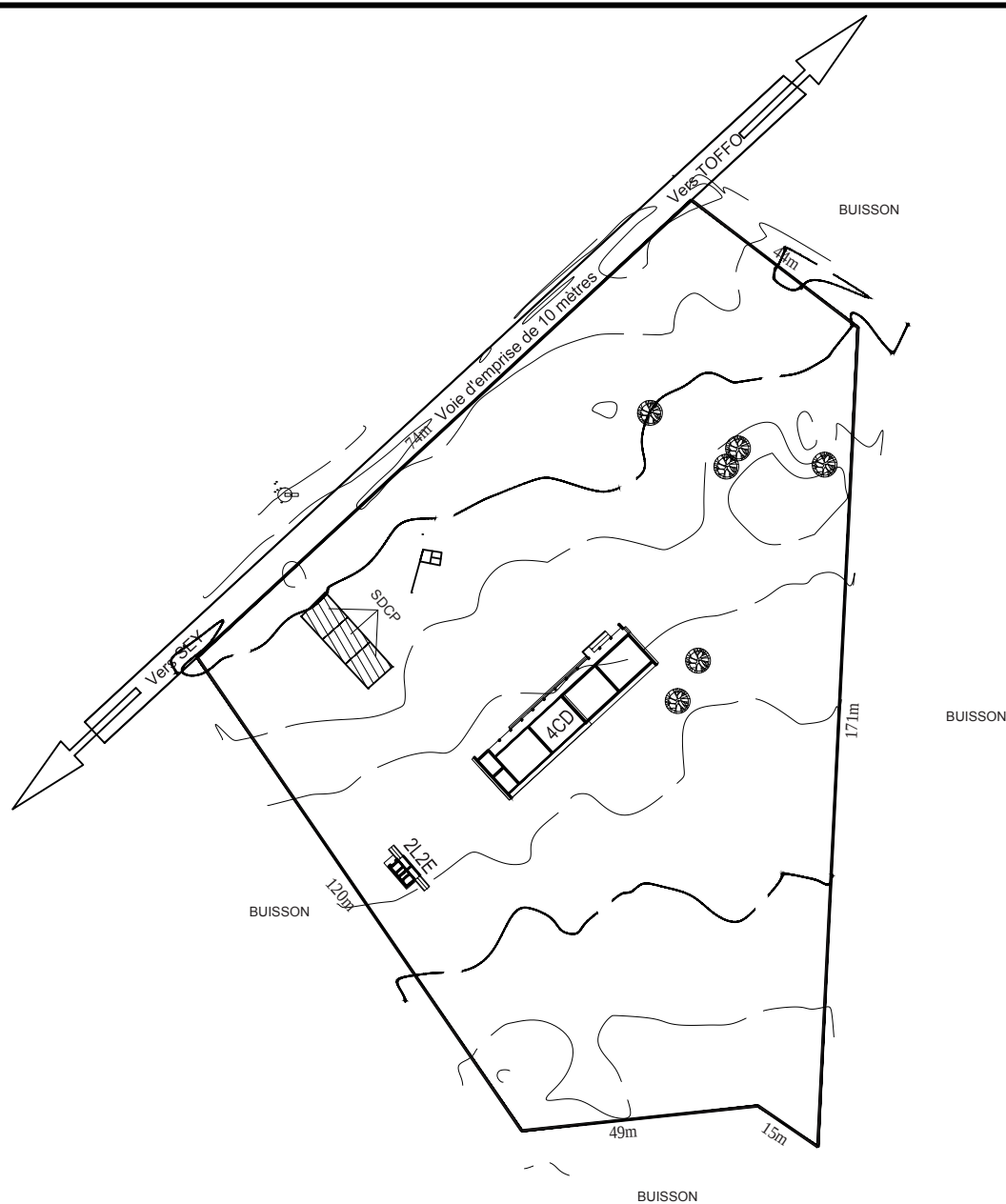
配置図 PLAN DE SITE
