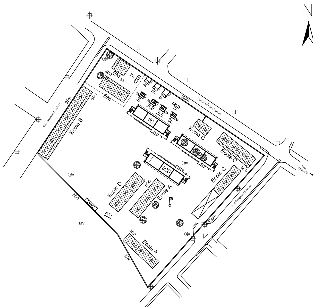
配置図 PLAN DE SITE
