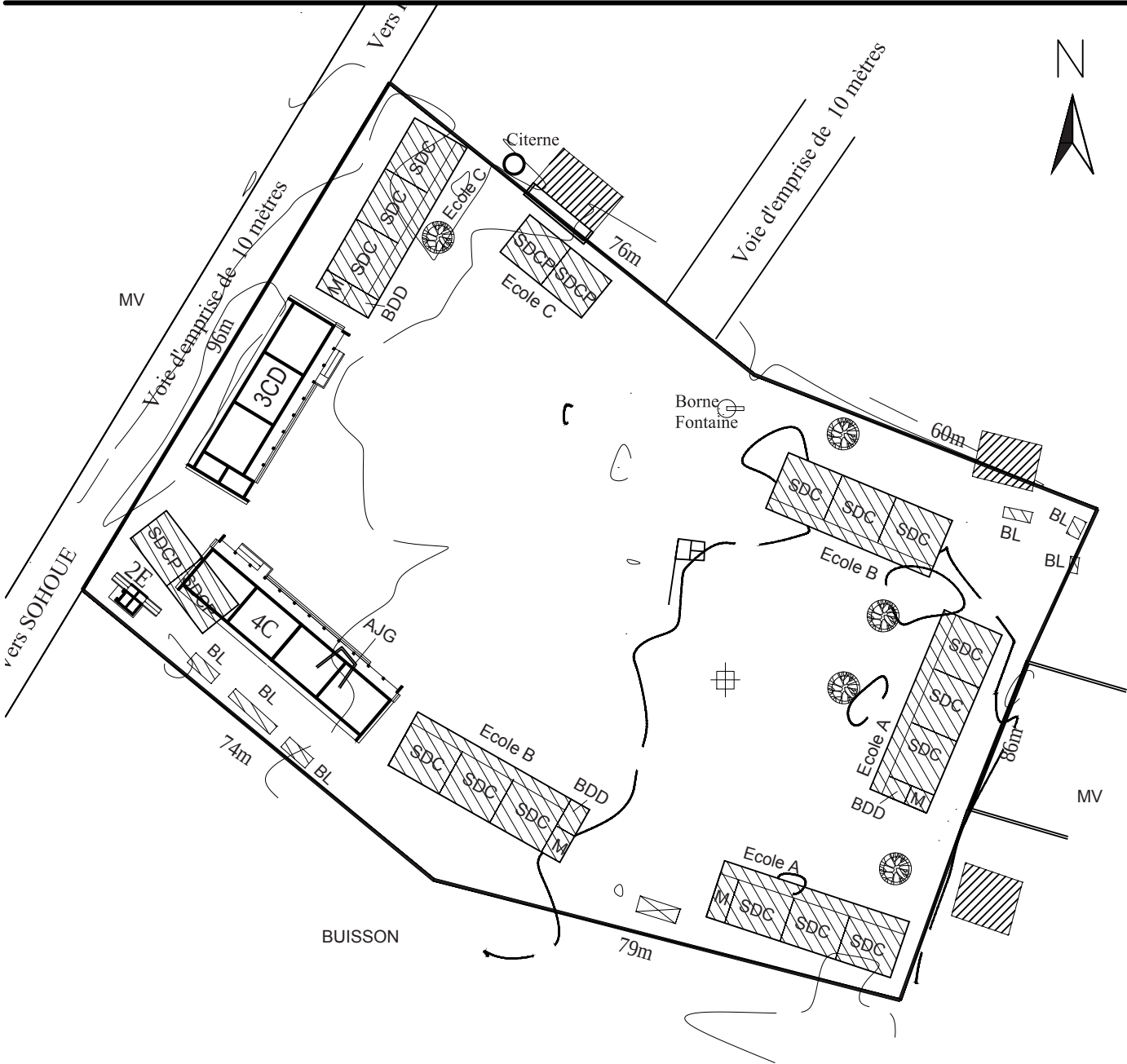
配置図 PLAN DE SITE 1 : 1000
