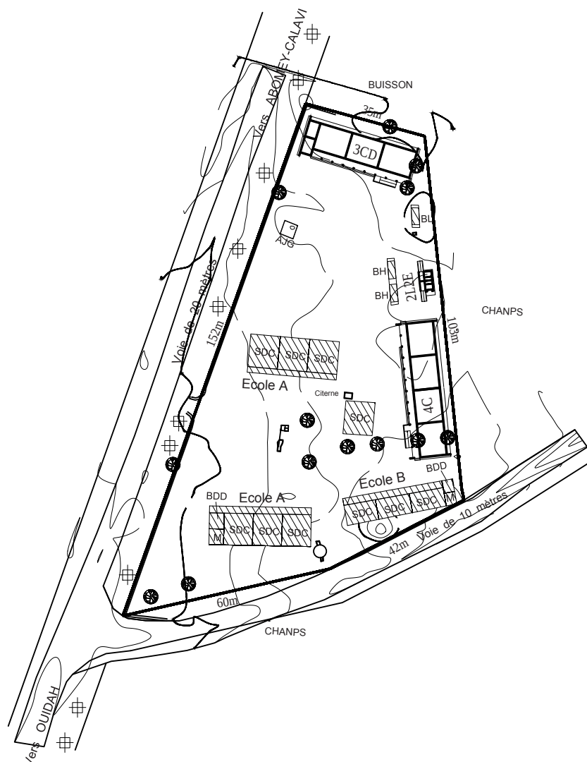
配置図 PLAN DE SITE
