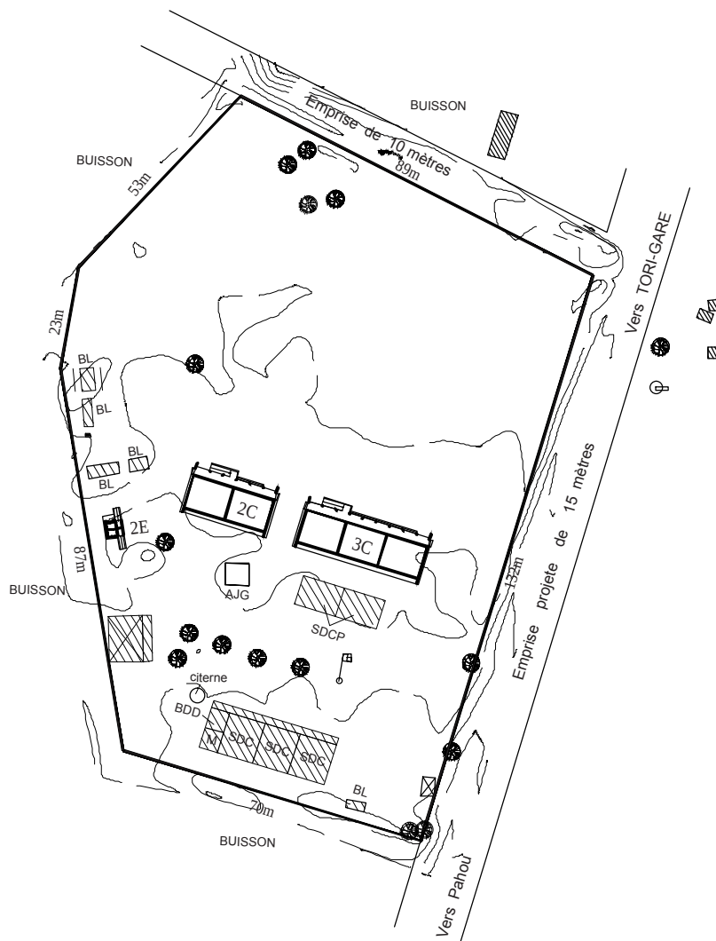
配置図 PLAN DE SITE
