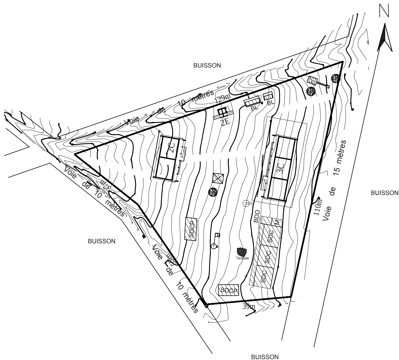
配置図 PLAN DE SITE
