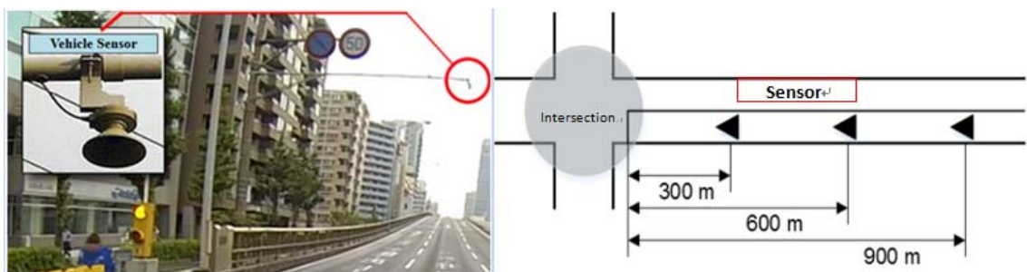
図 3.8 路側車両感知器設置イメージ(渋滞長計測システム)
