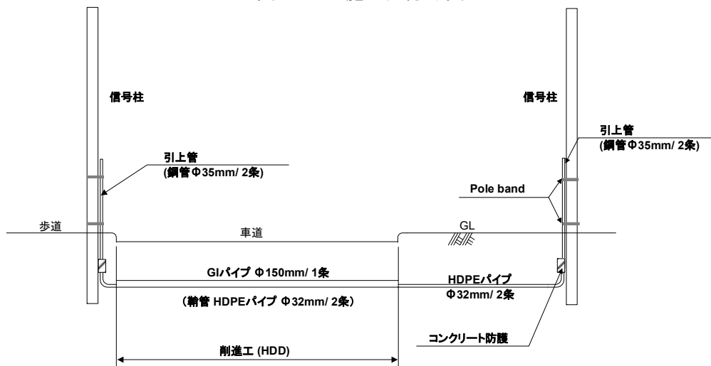
図 3.22 施工区分け図
