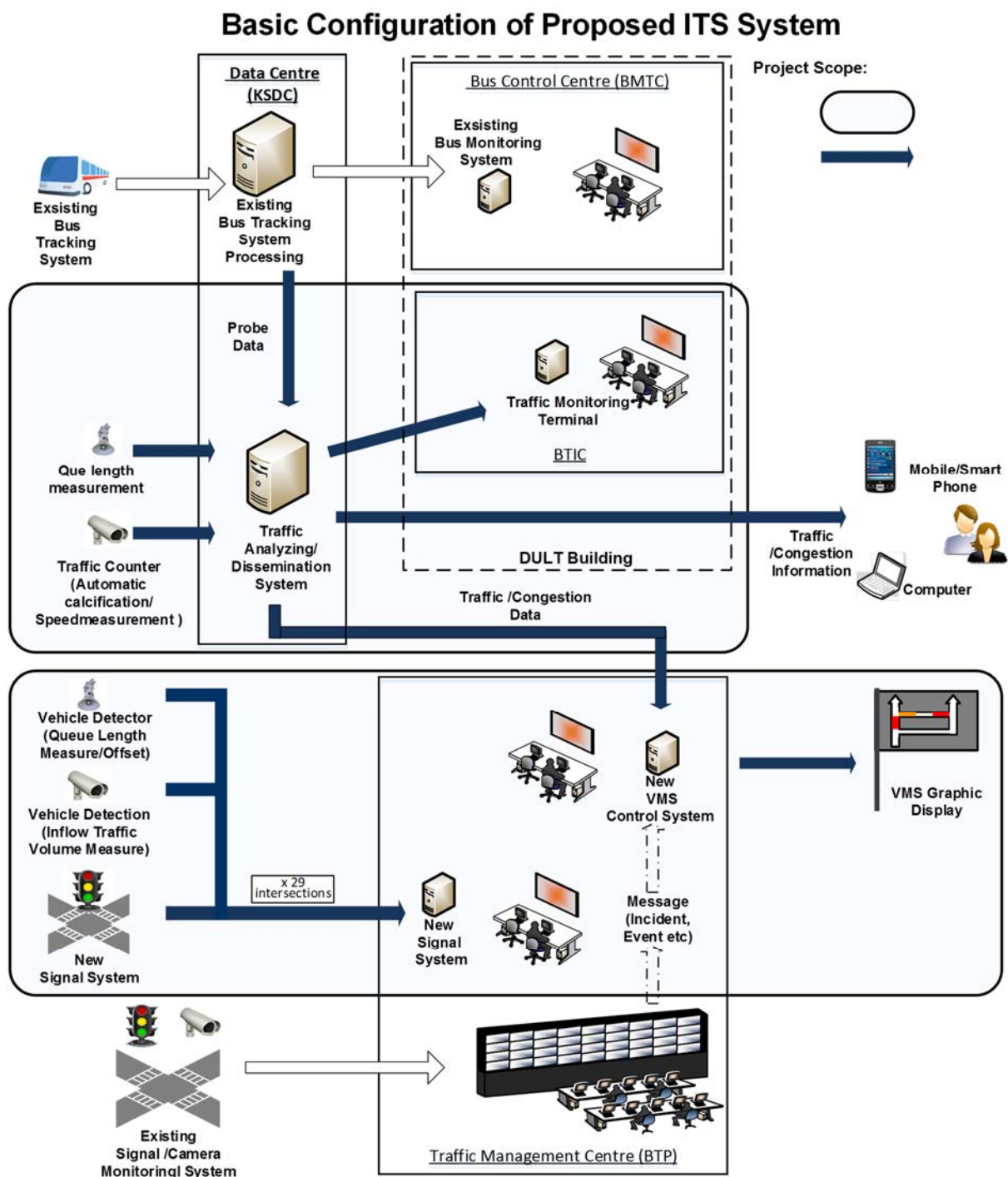
図 3.1 全体システム構成図
