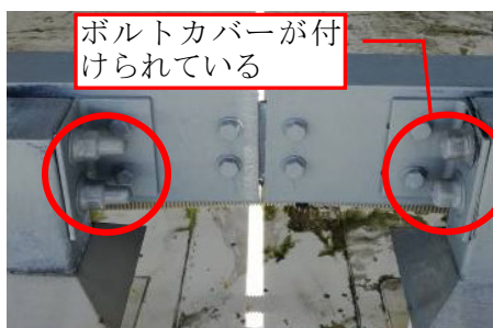
写真 3-3 架台部分ボルトへのカバー
