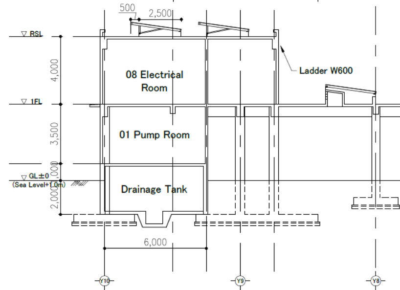
A-A' SECTION
