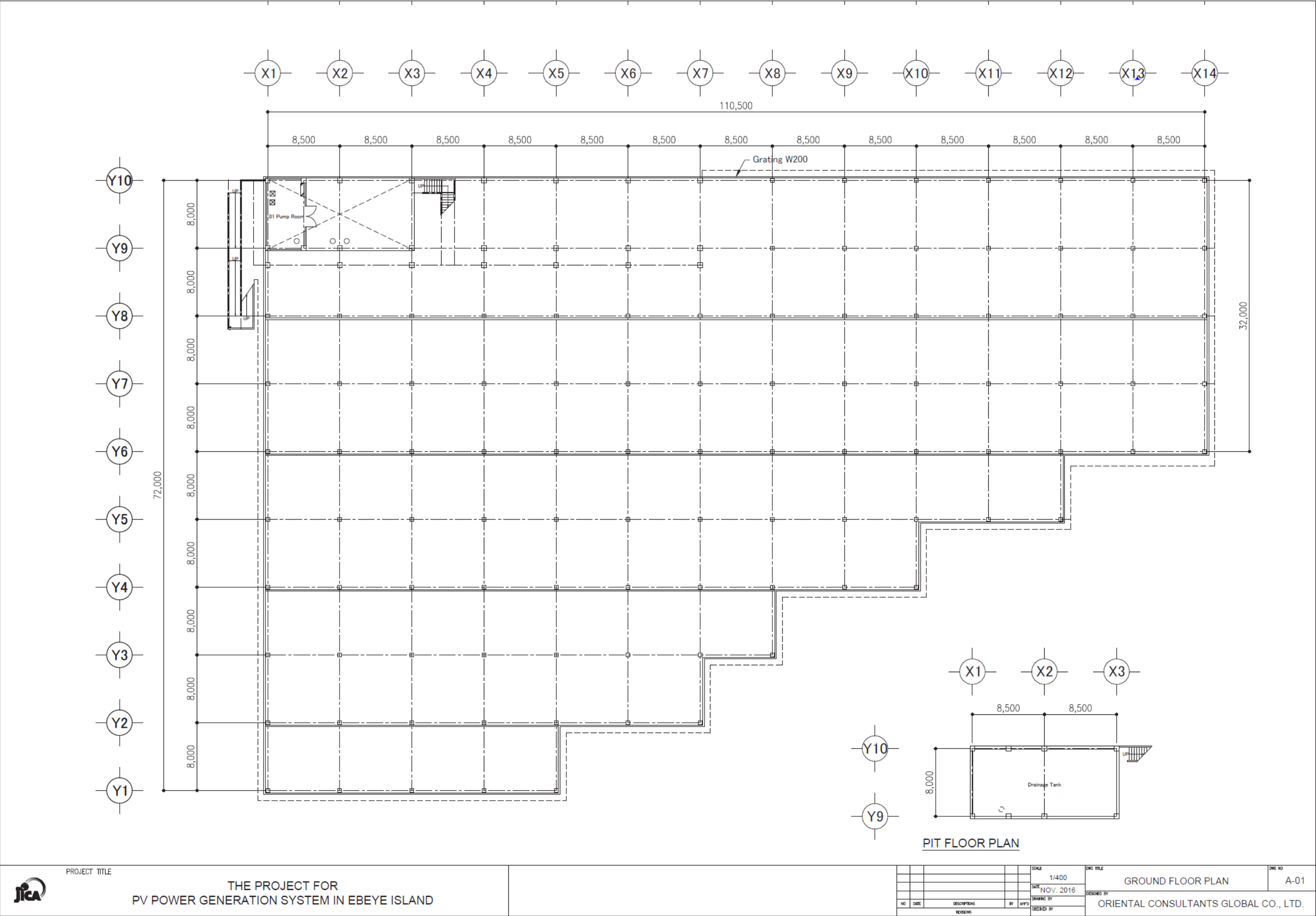
A-001(1) 平面図
