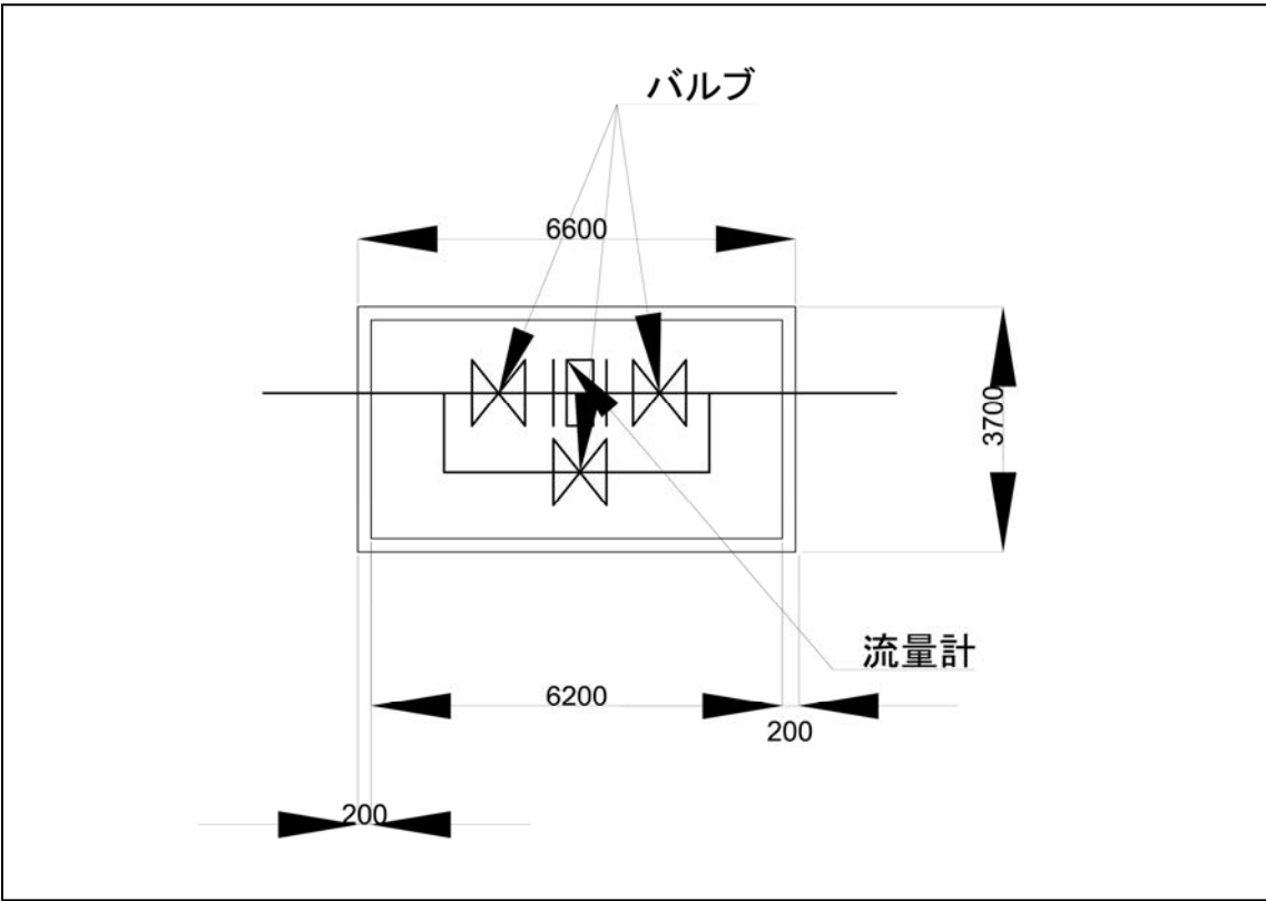
図 3-15 流量計室モデル図
