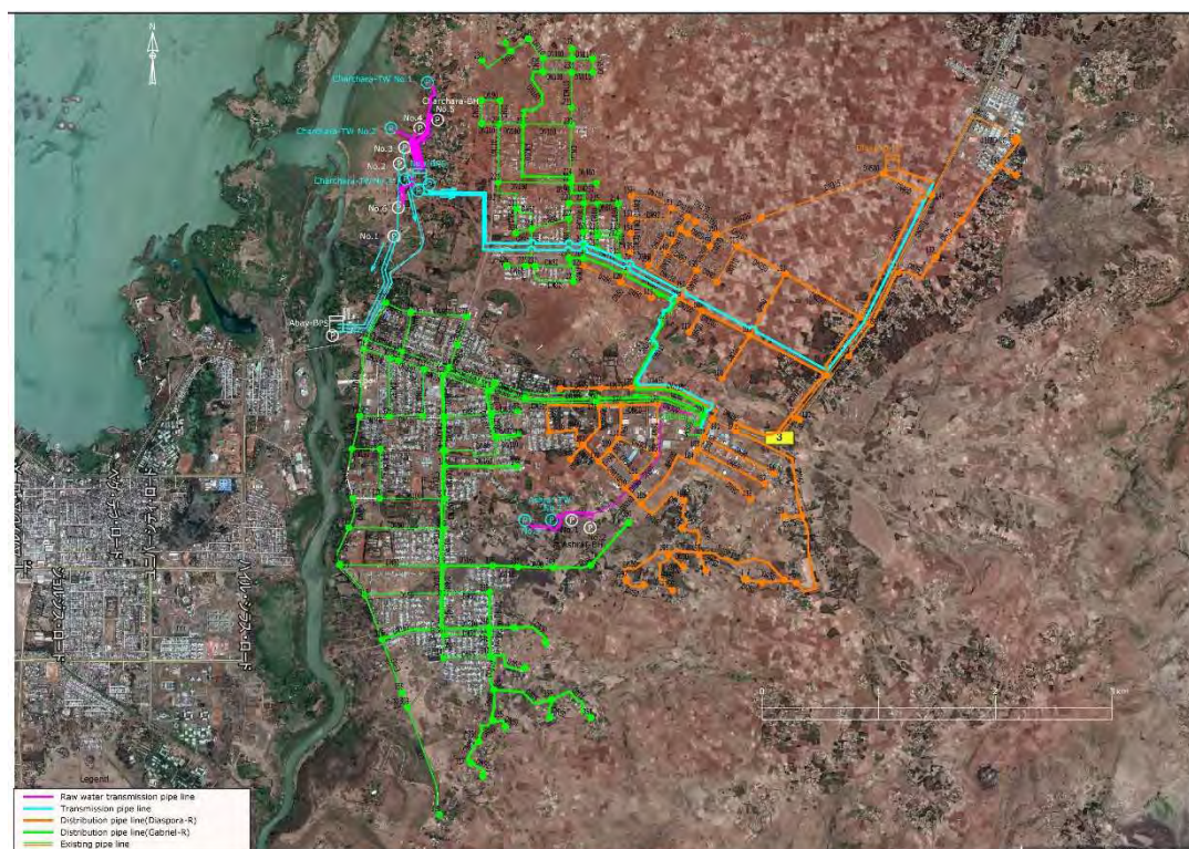
図 3-16 配管網図
