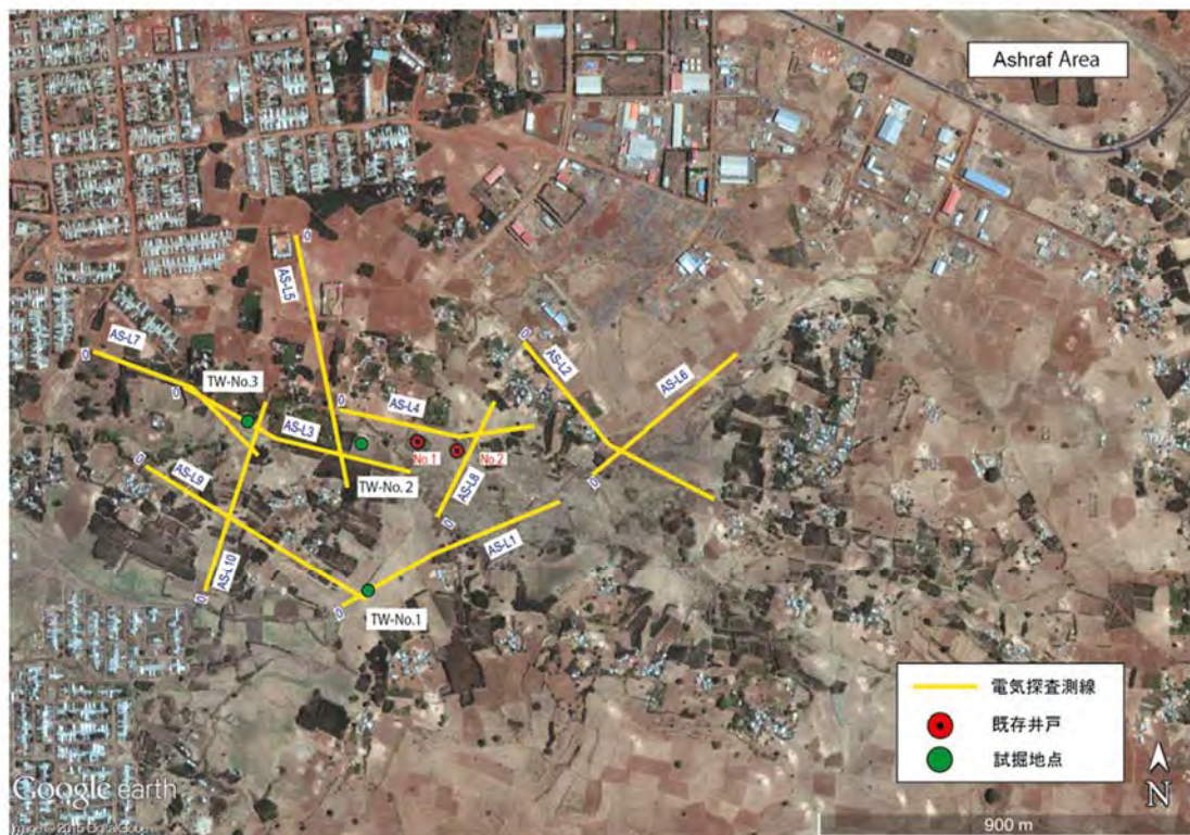
図 3-3 Ashraf 地区の電気探査実施位置および試掘位置図
