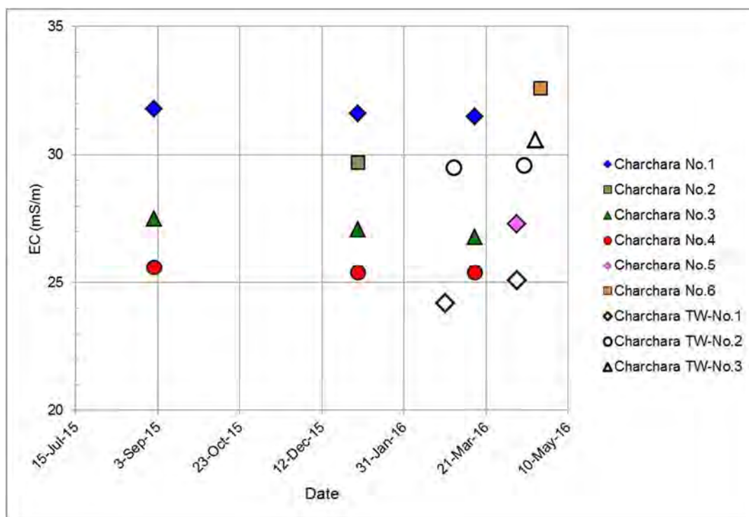
図 3-5 電気伝導度の測定結果
