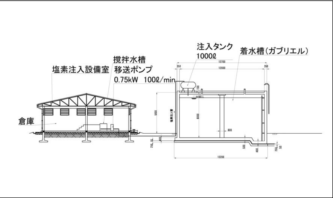
図 3-14 塩素注入設備モデル図
