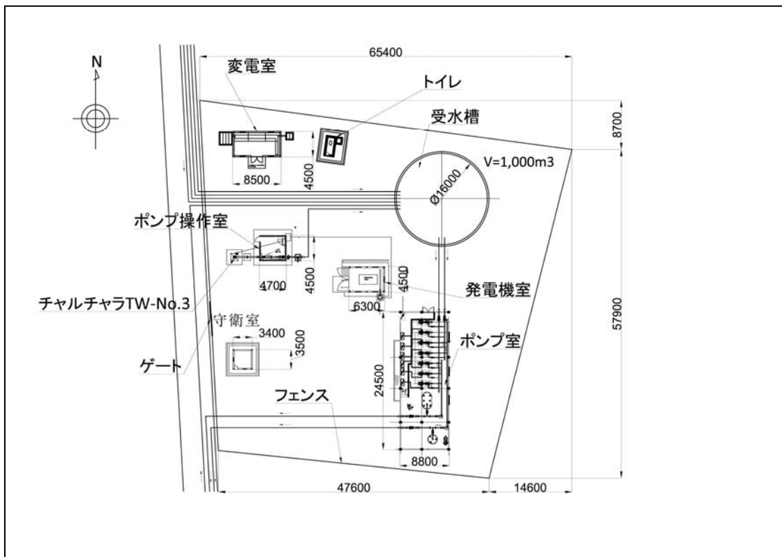
図 3-9 加圧ポンプ場 レイアウト図
