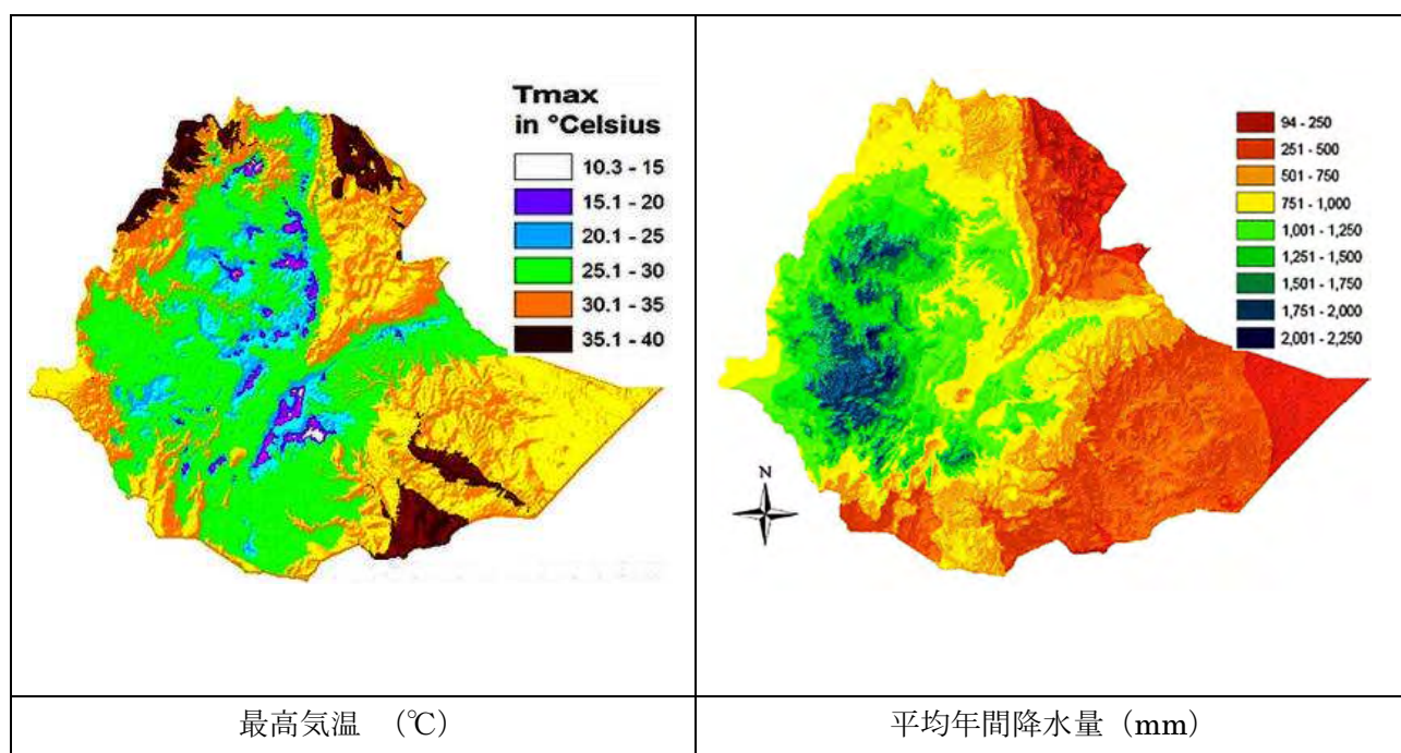
図 2-6 エチオピア最高気温、平均年間降水量図
