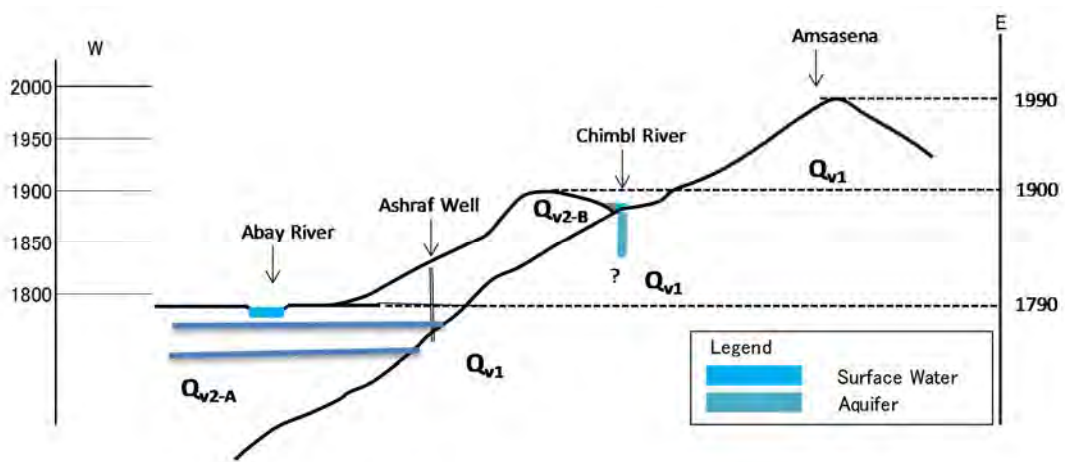
図 2-10 Ashraf 地区模式水理地質断面図 (Ashraf-Amsasena)
