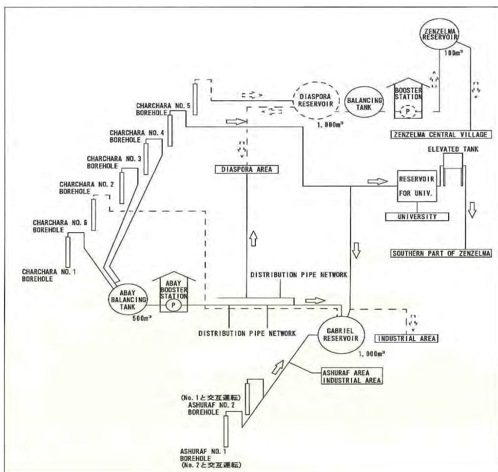
図 2-3 Zone 2 配水系模式図（点線は計画）
