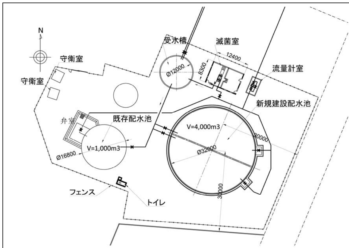
図 3-12 ガブリエル配水場 レイアウト図
