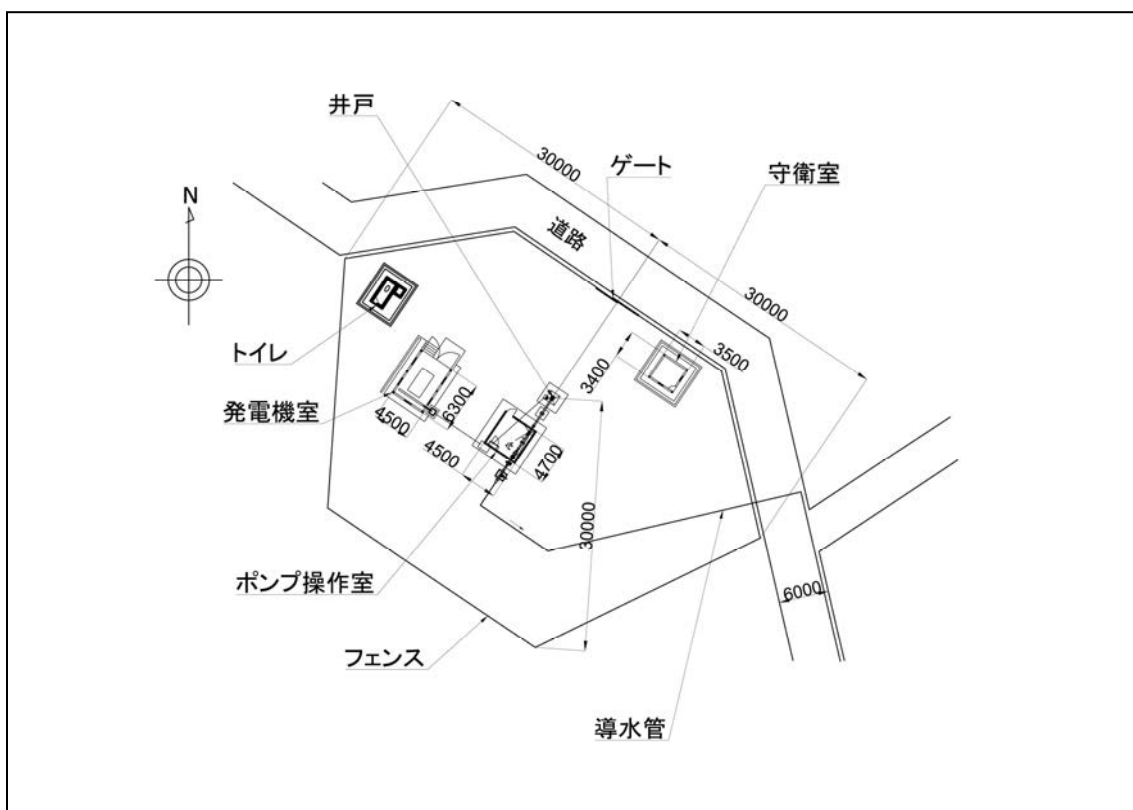
図 3-8 Charchara TW No. 1 レイアウト図
