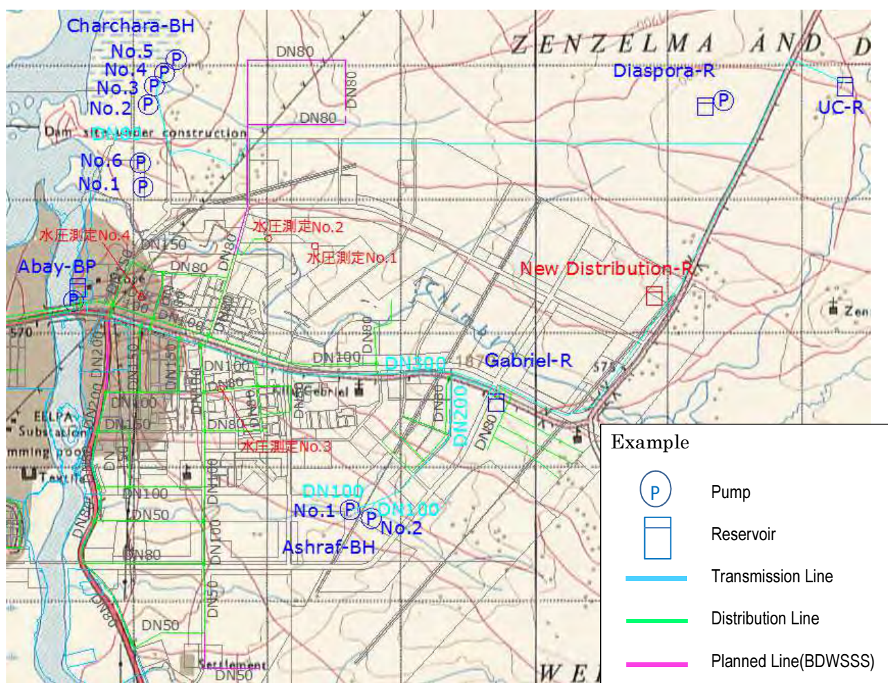
図 2-4 Zone 2 既設配水管位置図
