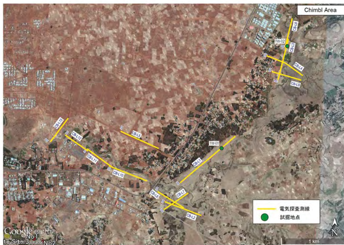
図 3-4 Chimbl 地区電気探査実施位置および試掘位置図
