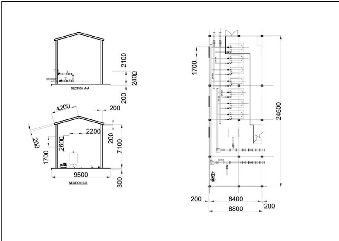
図 3-10 加圧ポンプ場ポンプ室 レイアウト図
