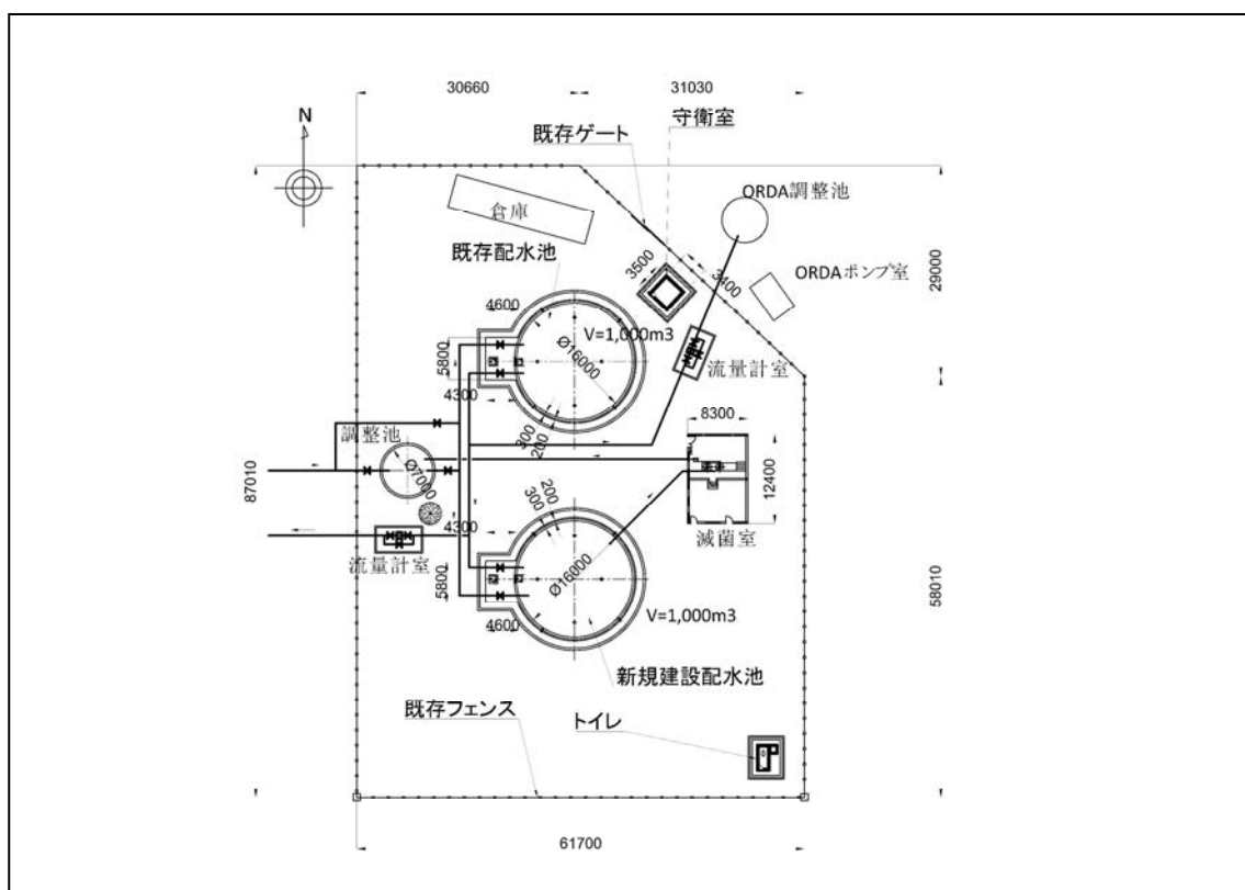
図 3-11 ディアスポラ配水場 レイアウト図
