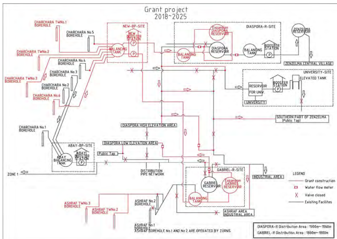
図 3-7 Zone 2 の計画水道施設フロー
