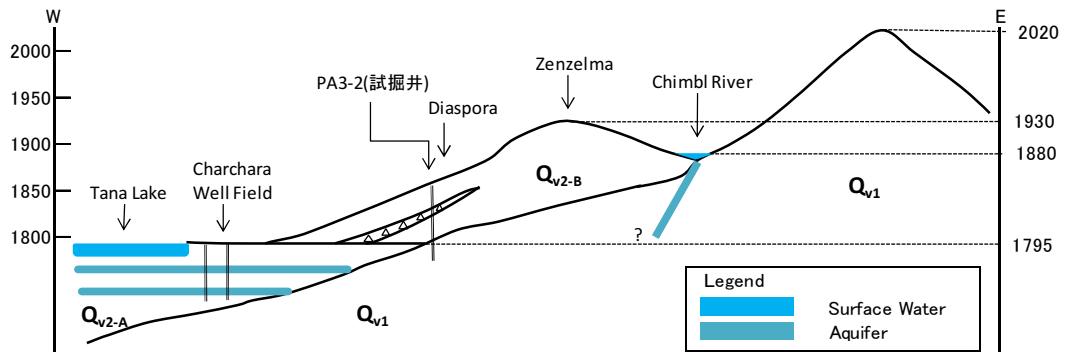
図 2-9 Charchara 地区模式水理地質断面図 (Charchara-Zenzerma)
