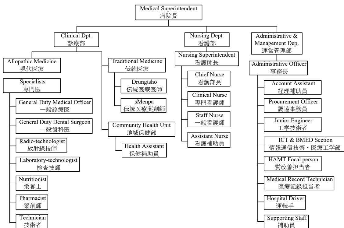
図 2-3 MERRH 組織図
