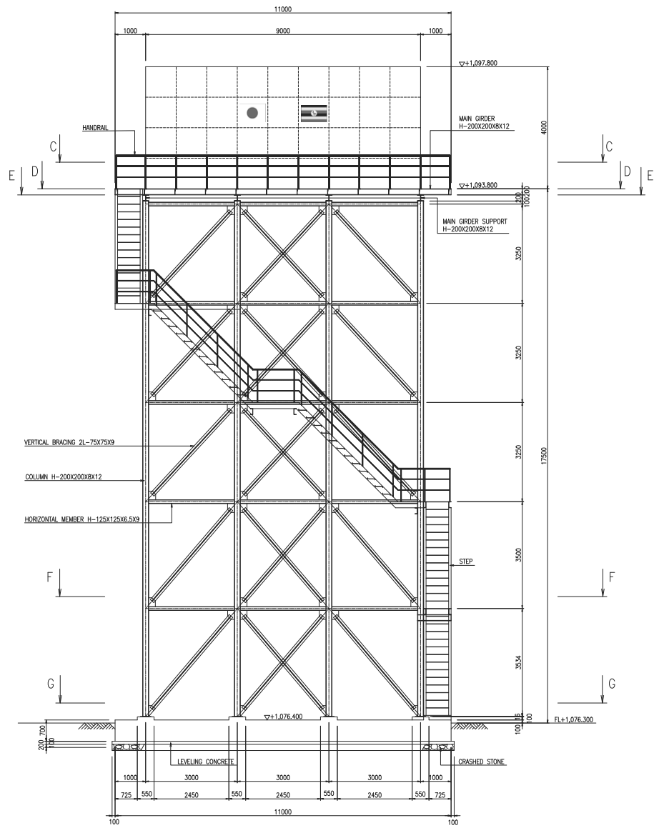
SECTION A-A
