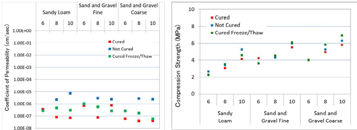
Նկար 4-9 Գրունտացեմենտի նվազող մակարդակով ջրաթափանցության (ձախ) և անսահմանափակ սեղման (աջ) թեստեր
