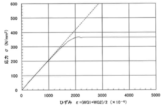
図-4 応力-ひずみ曲線 (鋼板 t=4mm)
