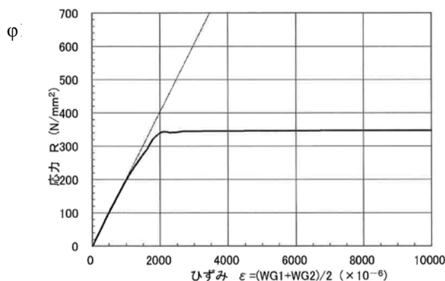
図-1 応力-ひずみ曲線 (φ6mm)
