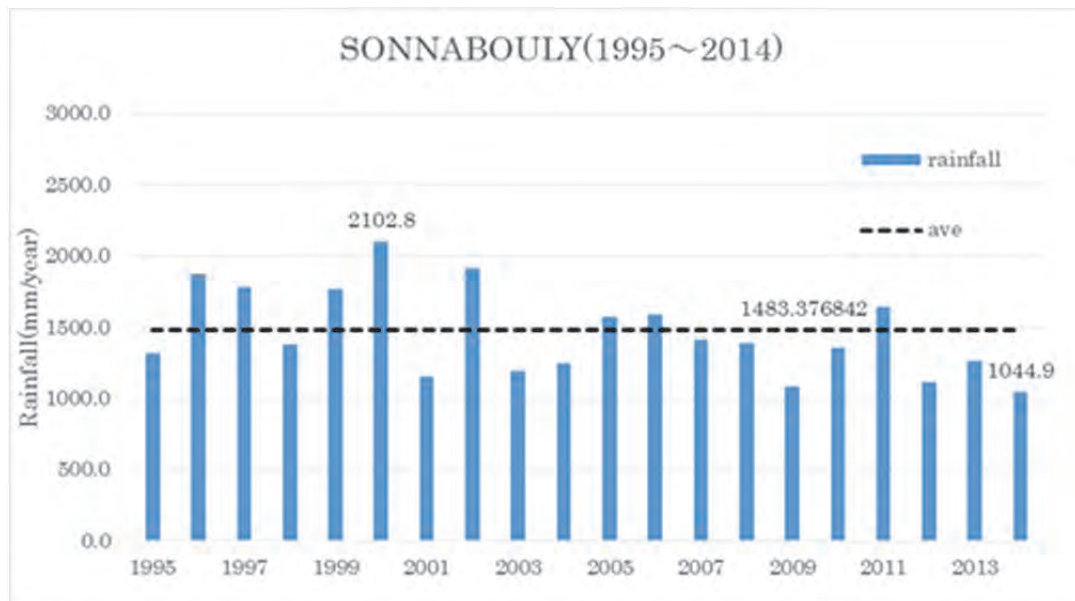
図 2.2.23 年間降水量
