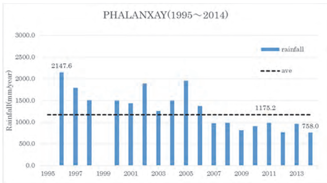
図 2.2.11 年間降水量
