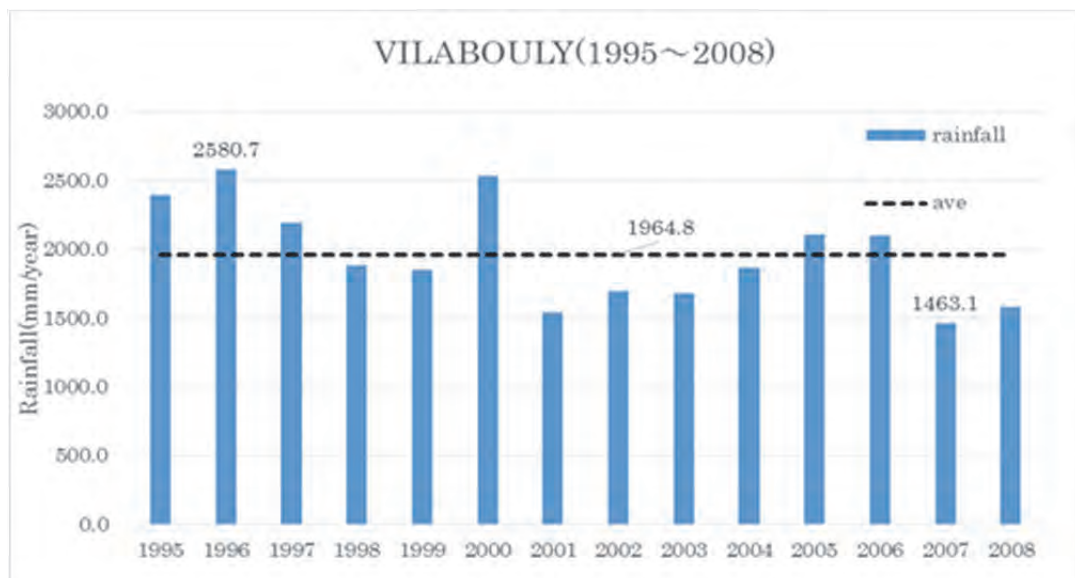
図 2.2.27 年間降水量
