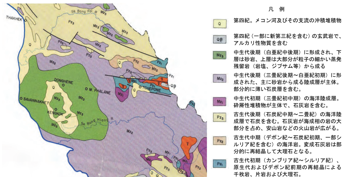
図 2.2.42 地質図
