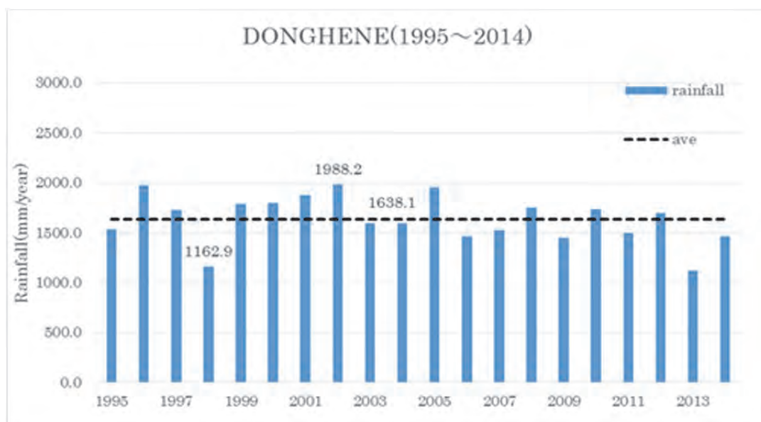
図 2.2.7 年間降水量
