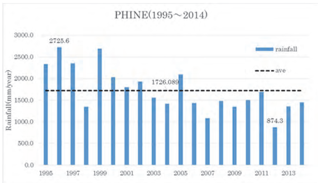
図 2.2.15 年間降水量
