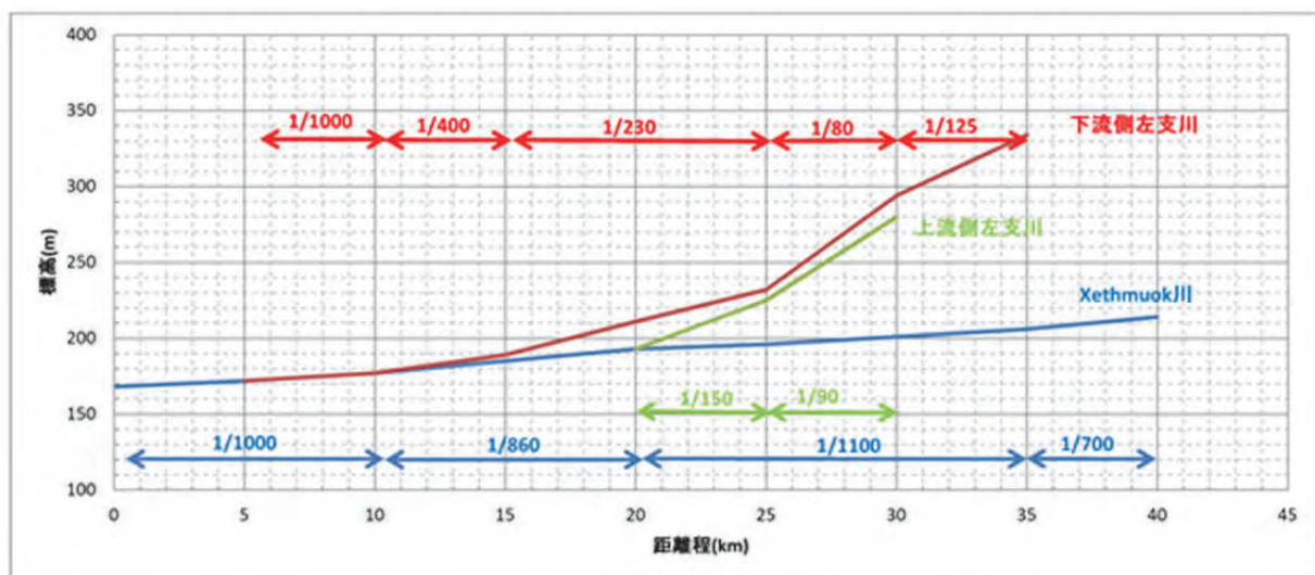
図 2. 2. 34 Xethamouk 川河川縦断図
