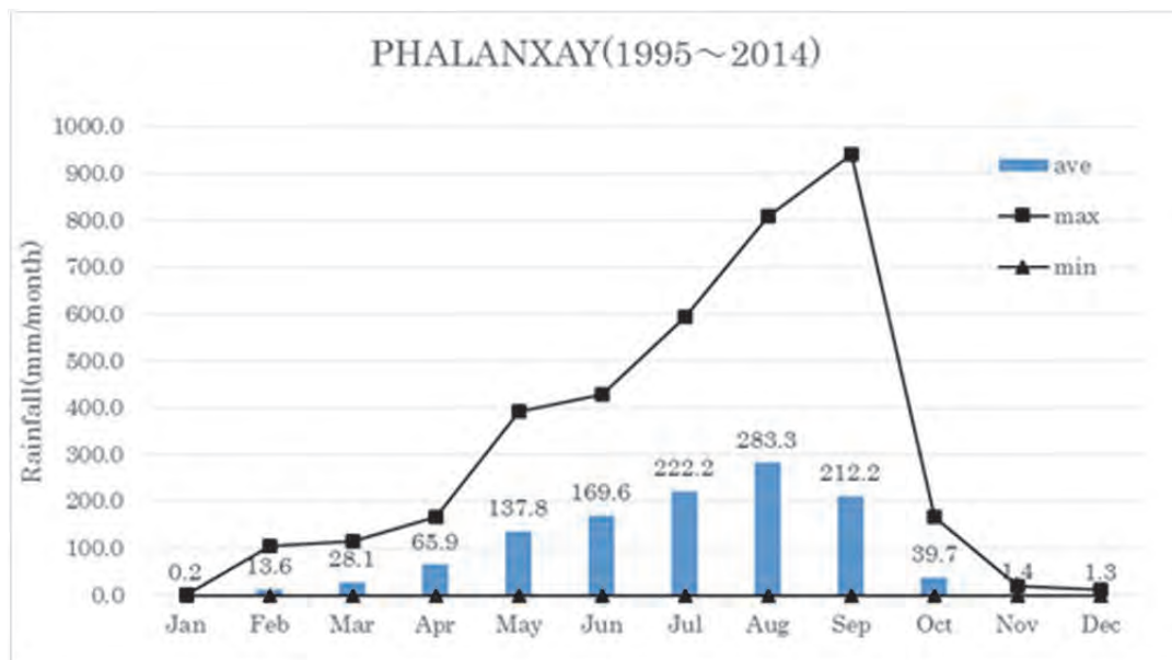
図 2.2.12 月別降水量
