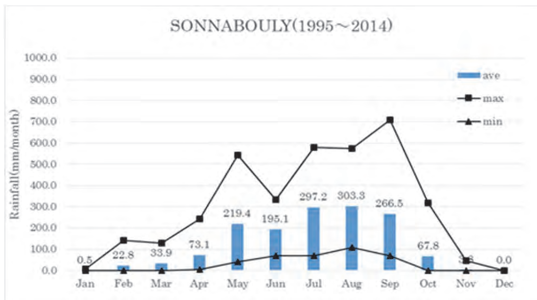
図 2.2.24 月別降水量
