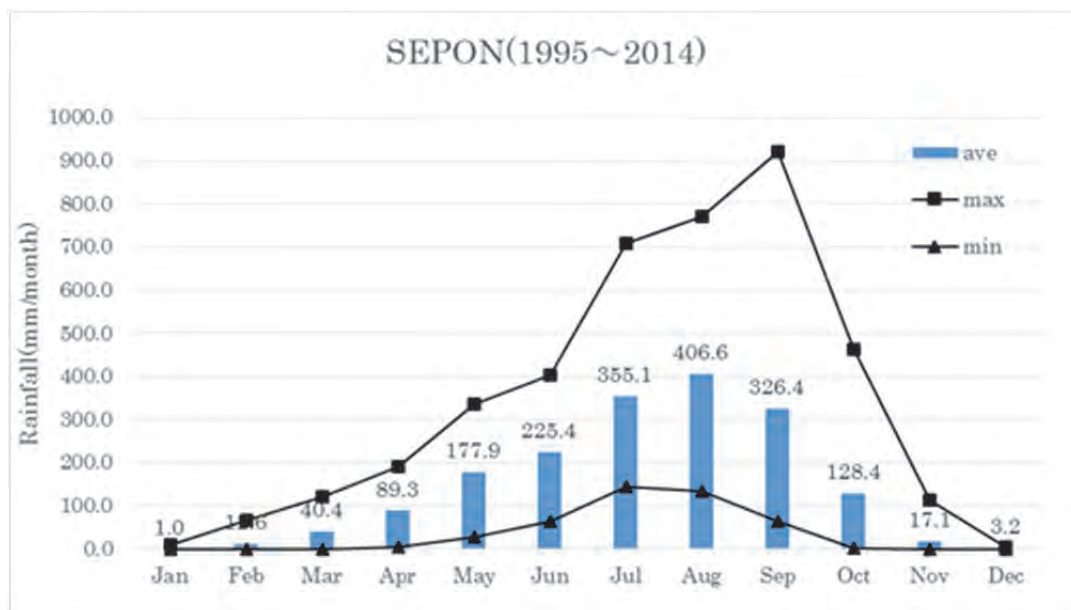
図 2.2.20 月別降水量
