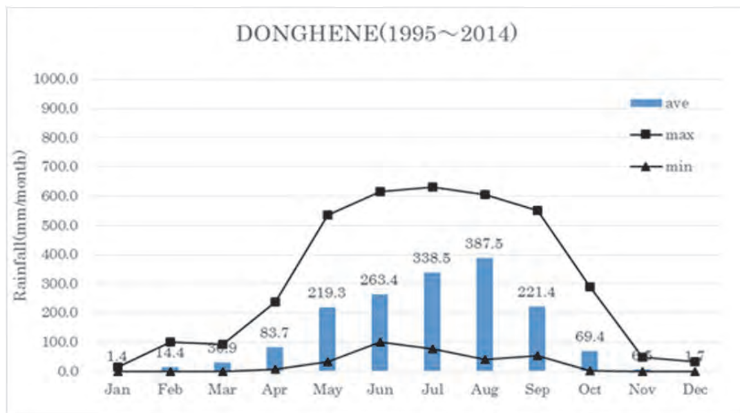
図 2.2.8 月別降水量
