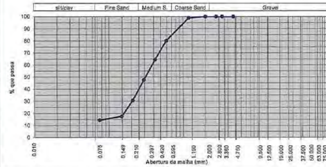
GRANULOMÉTRIC ACURVE
