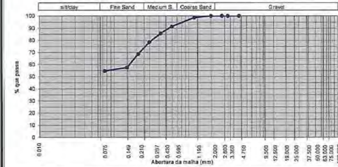
GRANULOMÉTRIC CURVE
