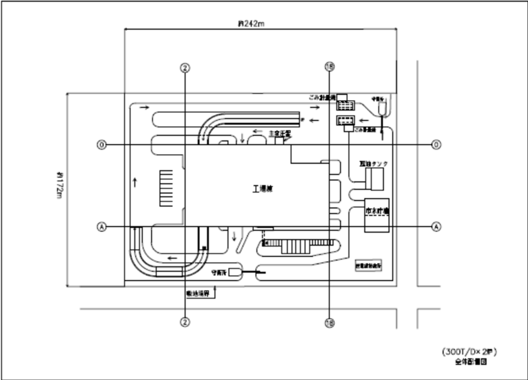
図3-8 全体配置図
