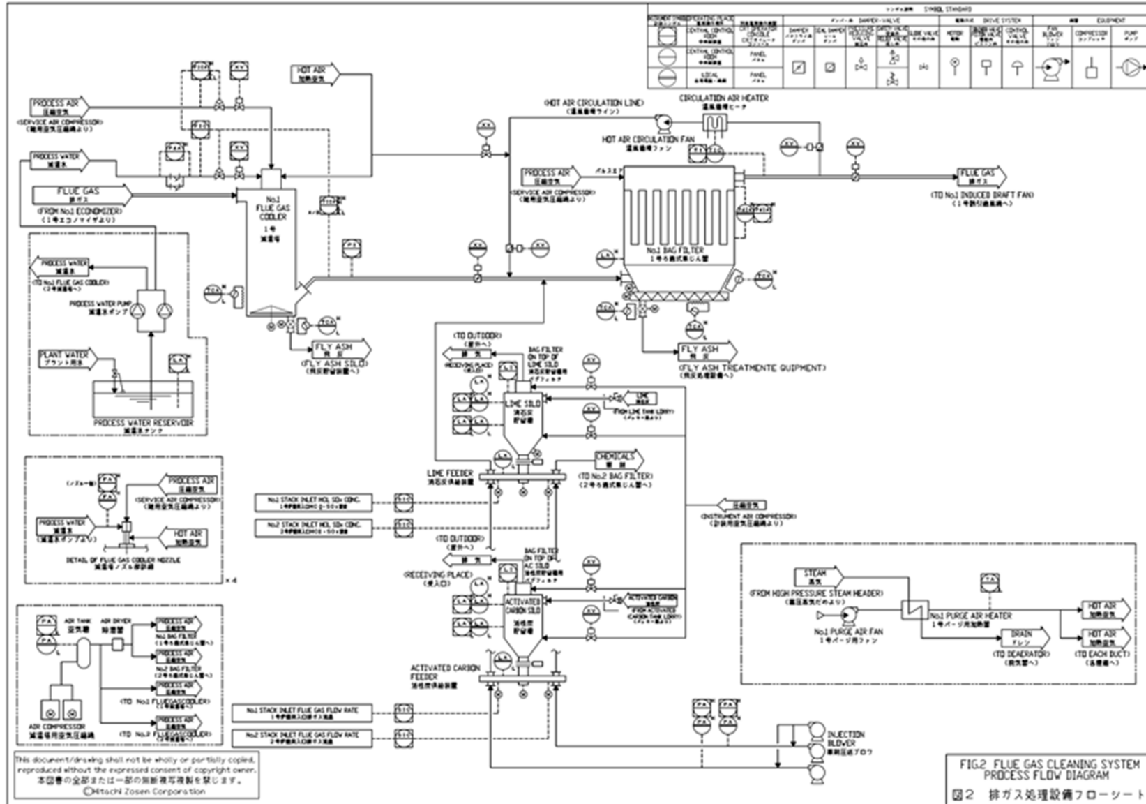
図3-13 排ガス処理フローシート
