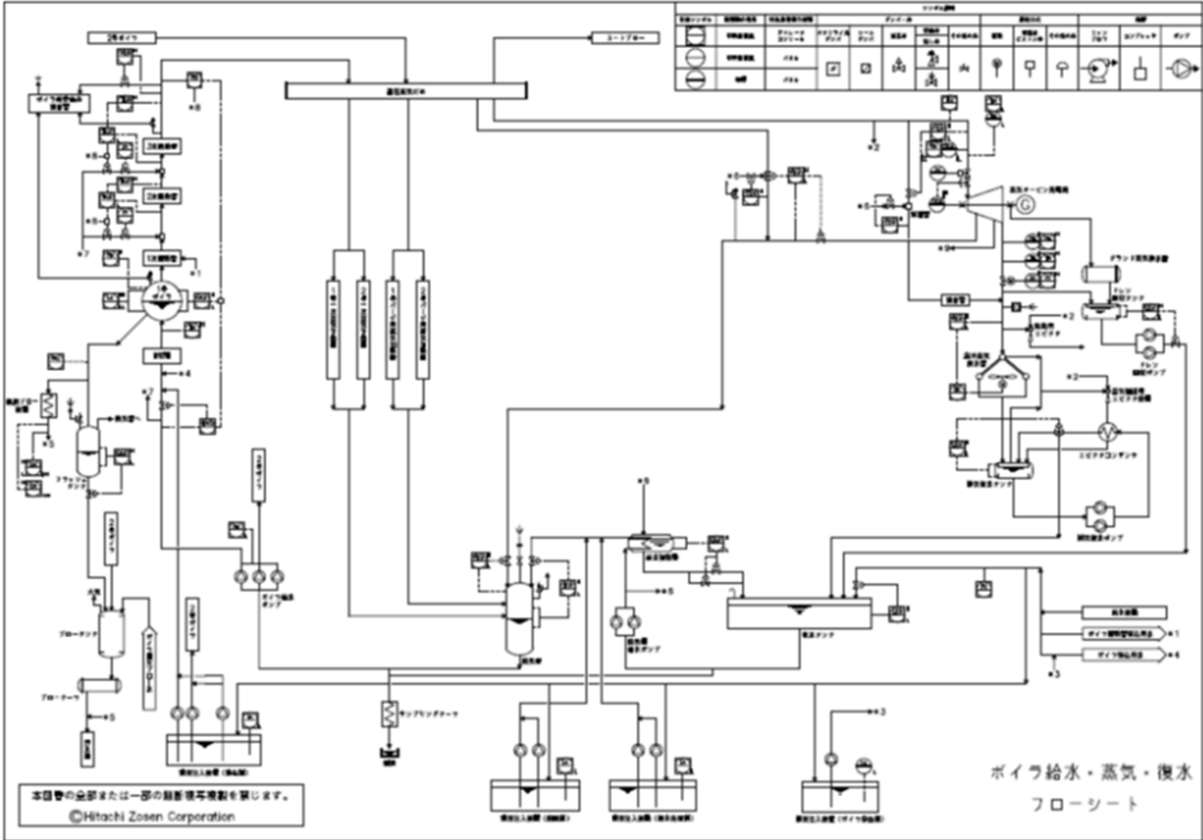
図3-14 ボイラー・復水フローシート
