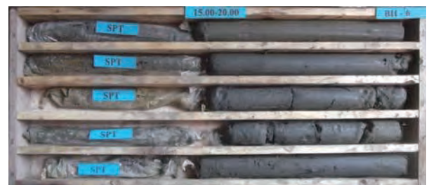
B-6 Box 4 Depth 15.00 - 20.00 m.
