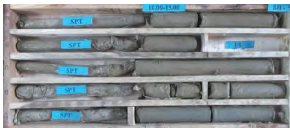
B-5 Box 3 Depth 10.00 - 15.00 m.
