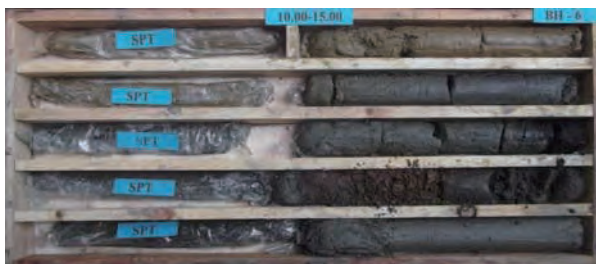
B-6 Box 3 Depth 10.00 - 15.00 m.
