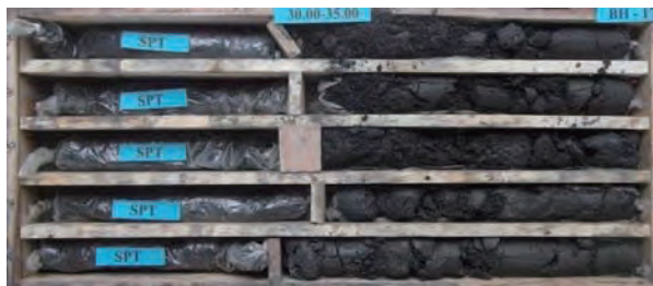
B-17 Box 7 Depth 30.00 - 35.00 m.
