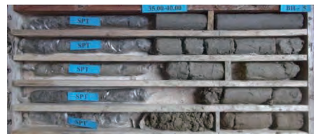
BH- Box 8 Depth 35.00 - 40.00 m.
