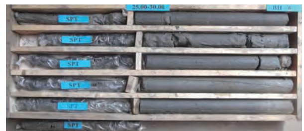
B-6 Box 6 Depth 25.00 - 30.00 m.
