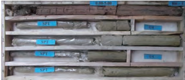
B-5 Box 1 Depth 0.00 - 5.00 m.
