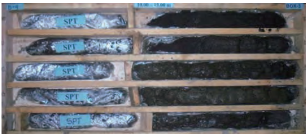
BH-4 Box 3 Depth 10.00 - 15.00 m.
