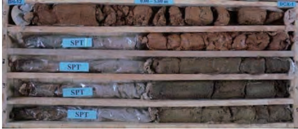
B-12 Box 1 Depth 0.00 - 5.00 m.
