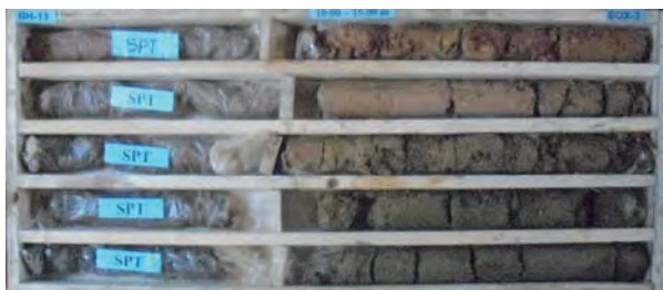
B-13 Box 3 Depth 10.00 - 15.00 m.
