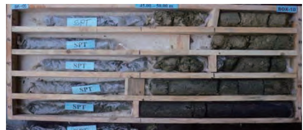
BH-3 Box 10 Depth 45.00 - 50.00 m.
