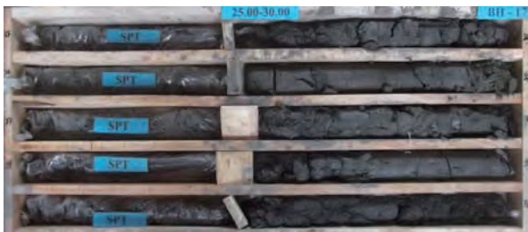
B-17 Box 5 Depth 20.00 - 25.00 m.
