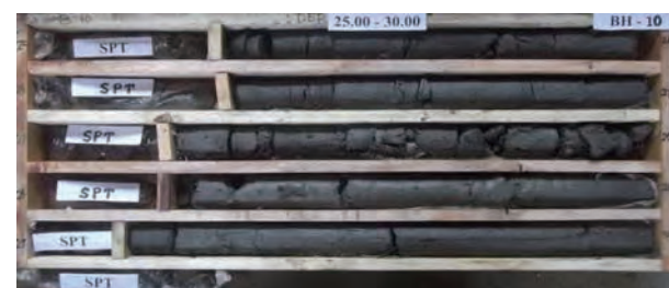
B-10 Box 6 Depth 25.00 - 30.00 m.
