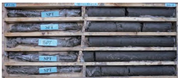
B-11 Box 9 Depth 40.00 - 45.00 m.
