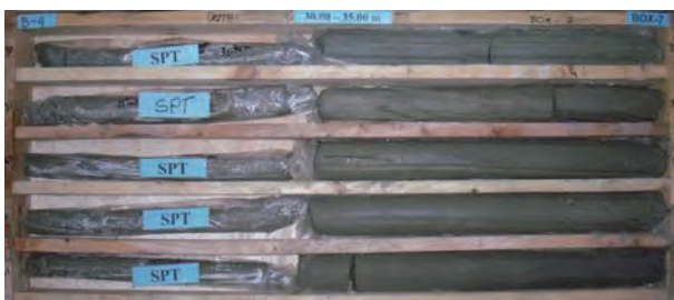
BH-4 Box 7 Depth 30.00 - 35.00 m.
