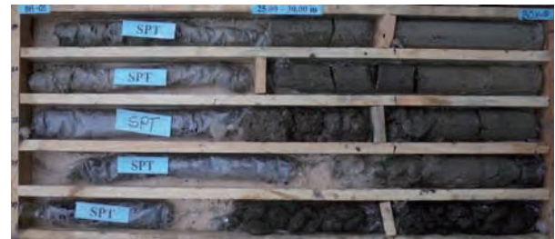
BH-3 Box 6 Depth 25.00 - 30.00 m.
