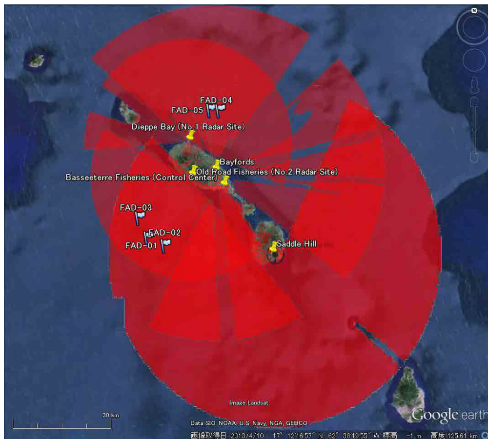
図 2-3 レーダー監視可能範囲（シミュレーション結果）
