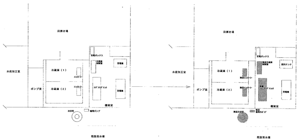
マリゴット漁港 冷蔵庫設備平面配置図
