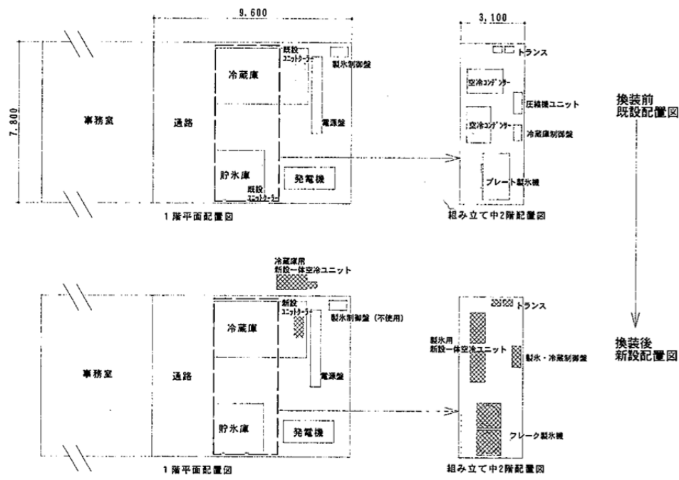
アーリング漁港 新設製氷・冷蔵冷却設備配置図
