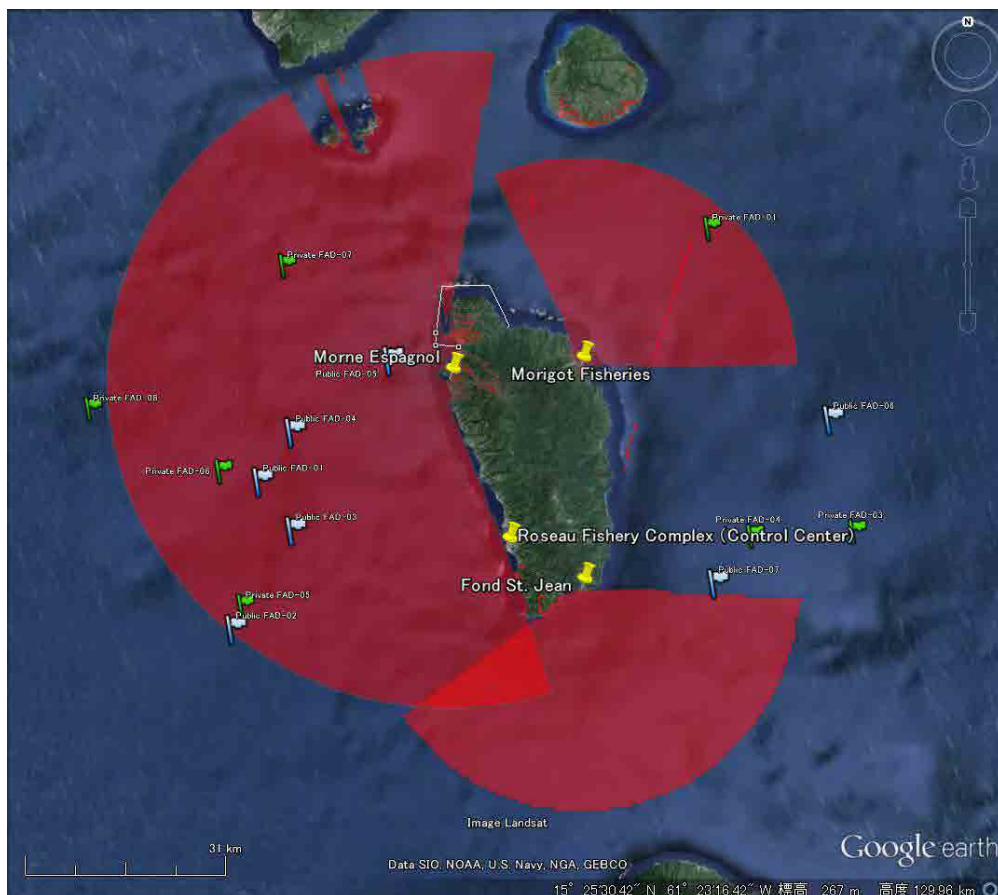
図 3-5 レーダー監視可能範囲（シミュレーション結果）
