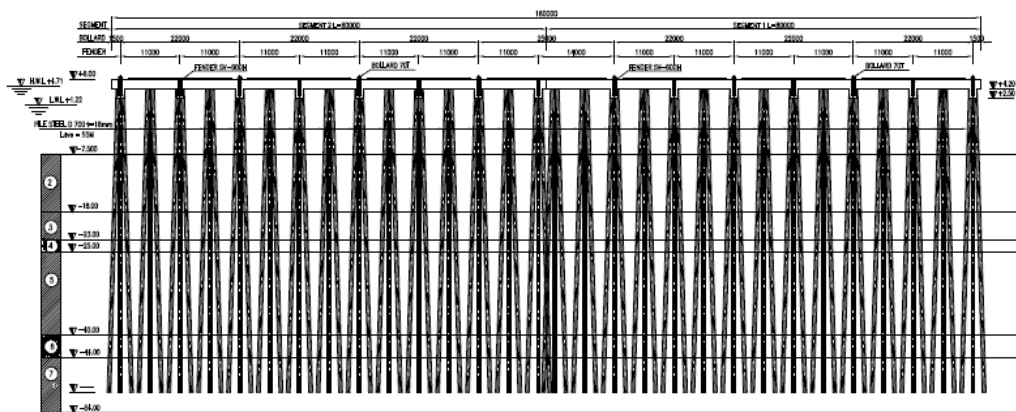
図 5.3.17 10,000DWT 棧橋側面図
