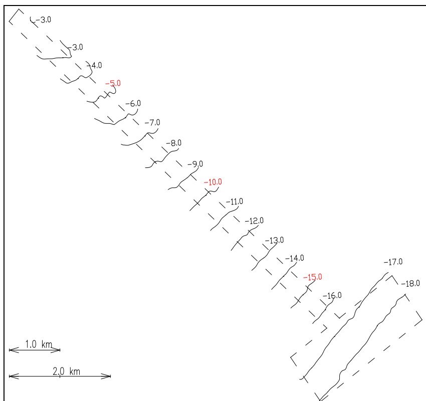
図 3.1.2 計画地域（連絡橋予定地）における深浅測量結果
