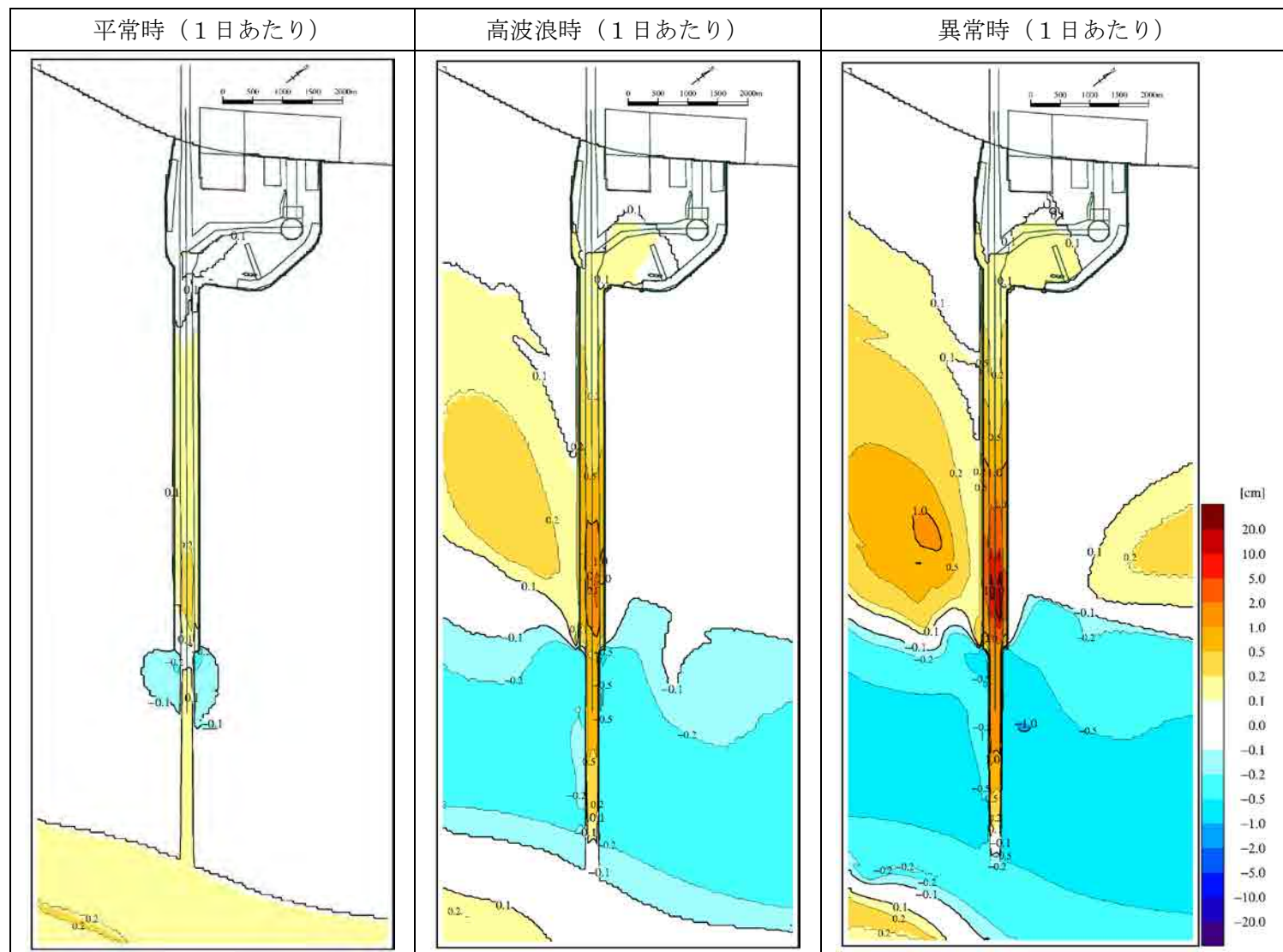
図 4.6.5(1) 埋没計算結果 (1 st Phase-E : 防砂堤 6,000m)
