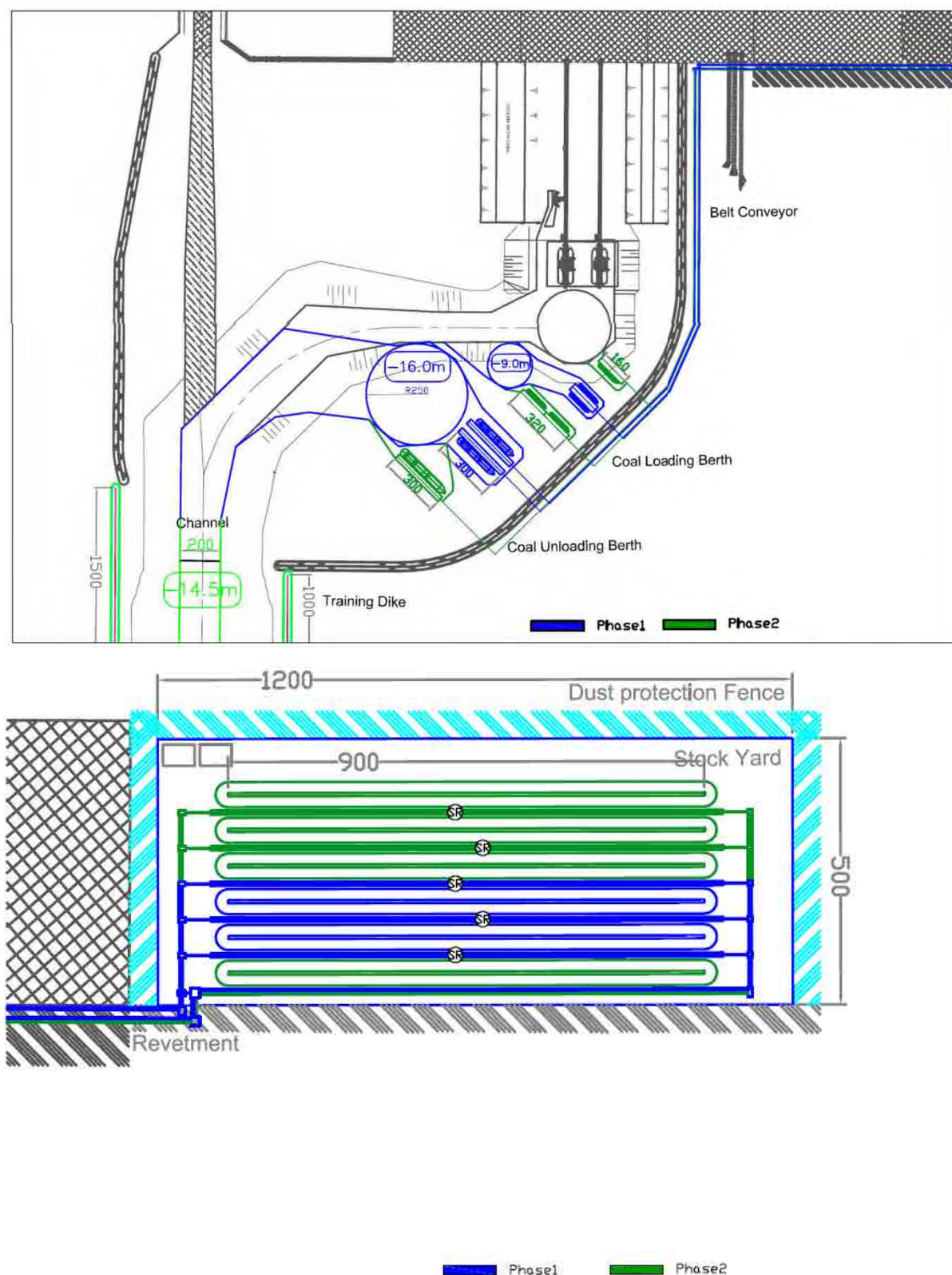
図 9.2.5 港湾・ターミナル中期整備計画平面図
