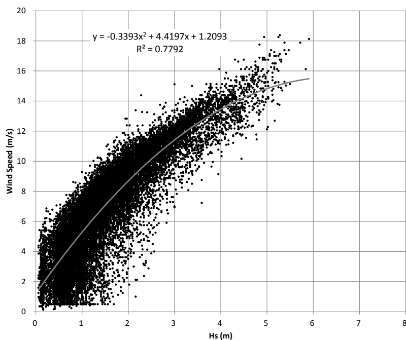
図 4.2.4 代表波浪の設定地点における波高と風速の関係
