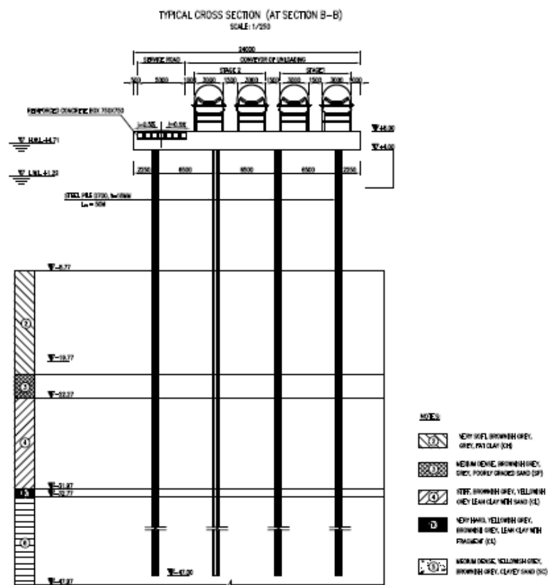
図 5.3.21 トレッセル設計図（平面、側面、断面）
