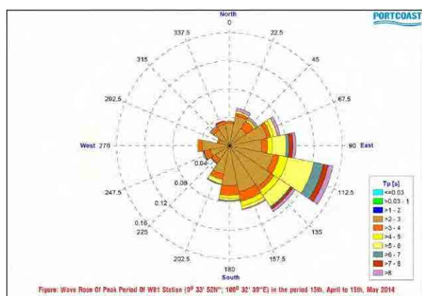
図 3.3.3 波向・周期頻度図
