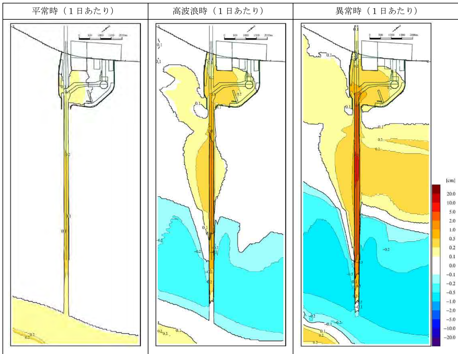
図 4.6.1(1) 埋没計算結果 (1 st Phase-A : 防砂堤なし)
