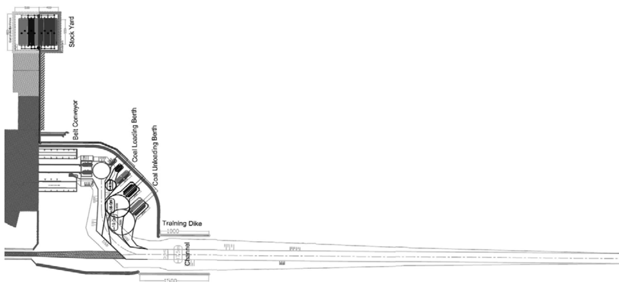
図 5.3.31 航路配置図
