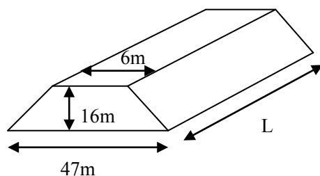
図 5.2.8 ストックパイル形状
