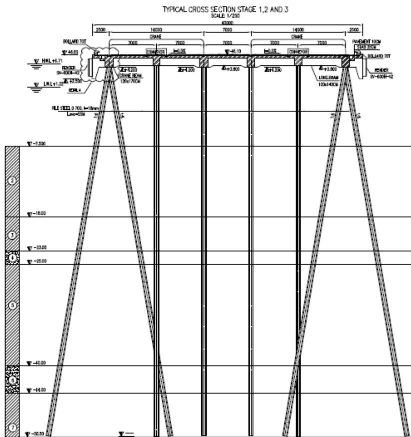
図 5.3.18 10,000DWT 栈橋標準断面図
