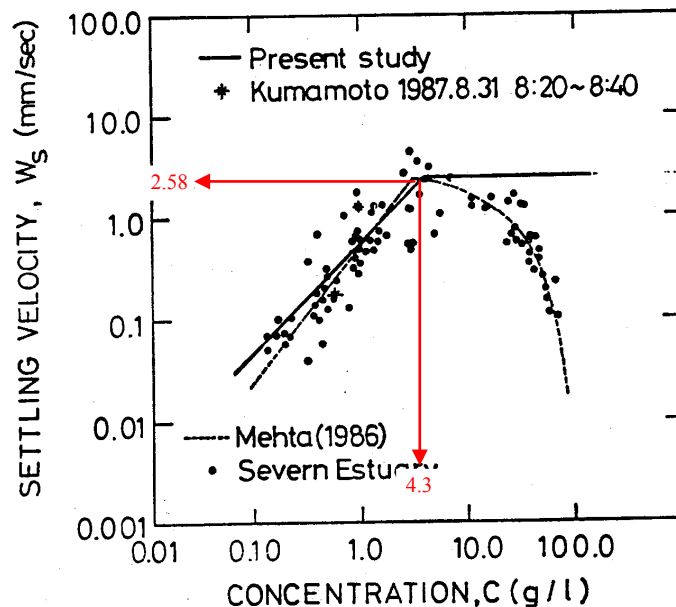
図 4.4.1 泥の濃度と沈降速度の関係
