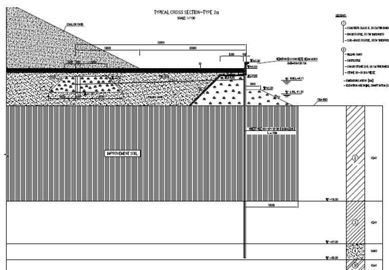
図 5.3.20 護岸標準断面図
