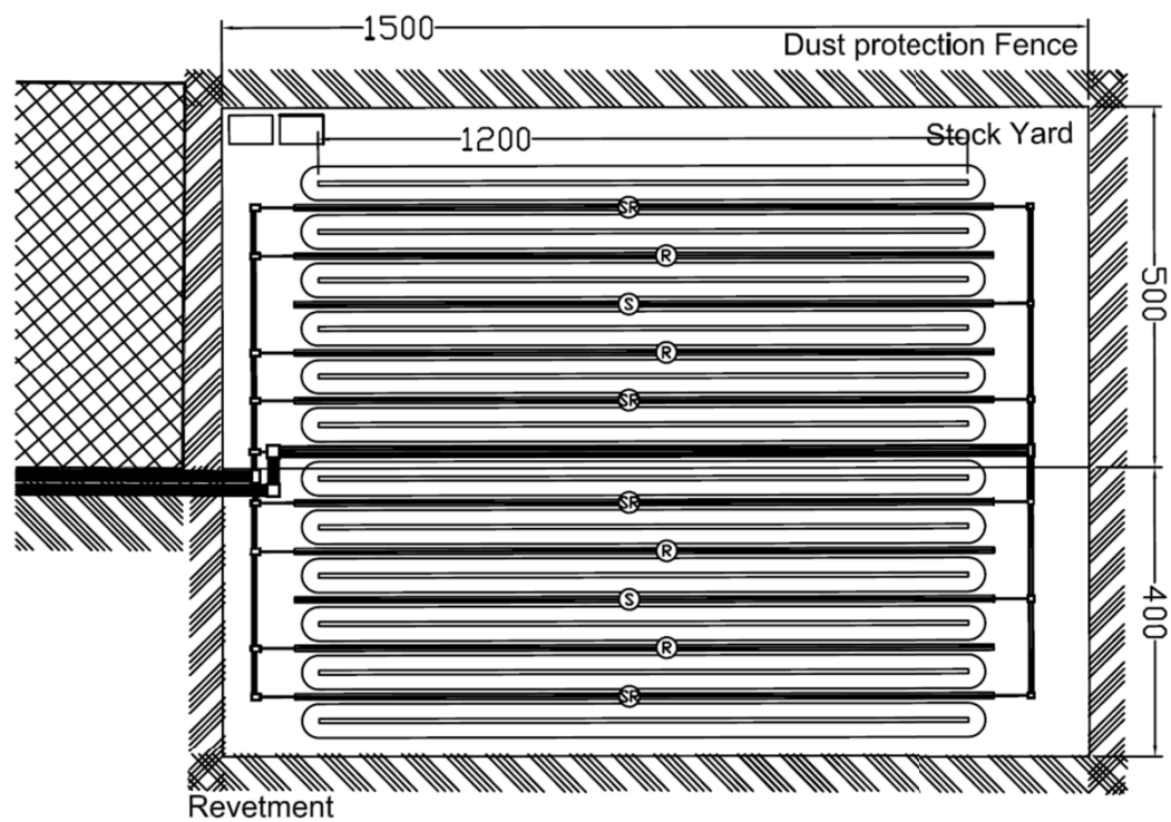
図 5.2.10 ターミナルレイアウト (港外案 (防波堤あり))
