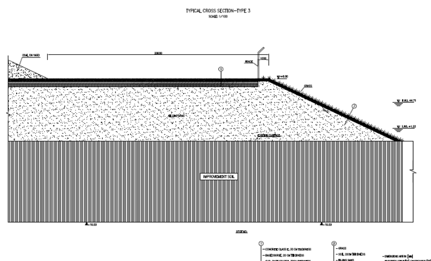
図 5.3.26 陸上部造成斜面部断面図
