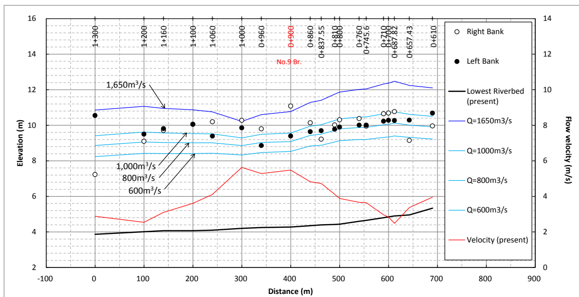
図 2-2-13 現況河道の水位縦断面図（新線橋）
