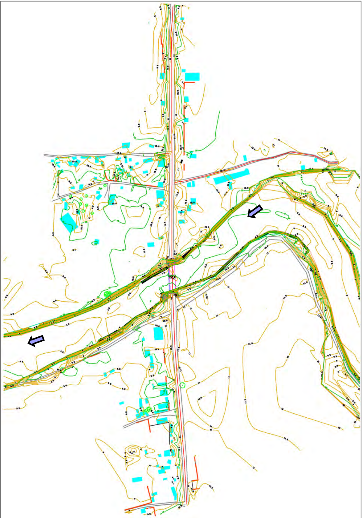
図 2-2-17 新線橋梁地形図
