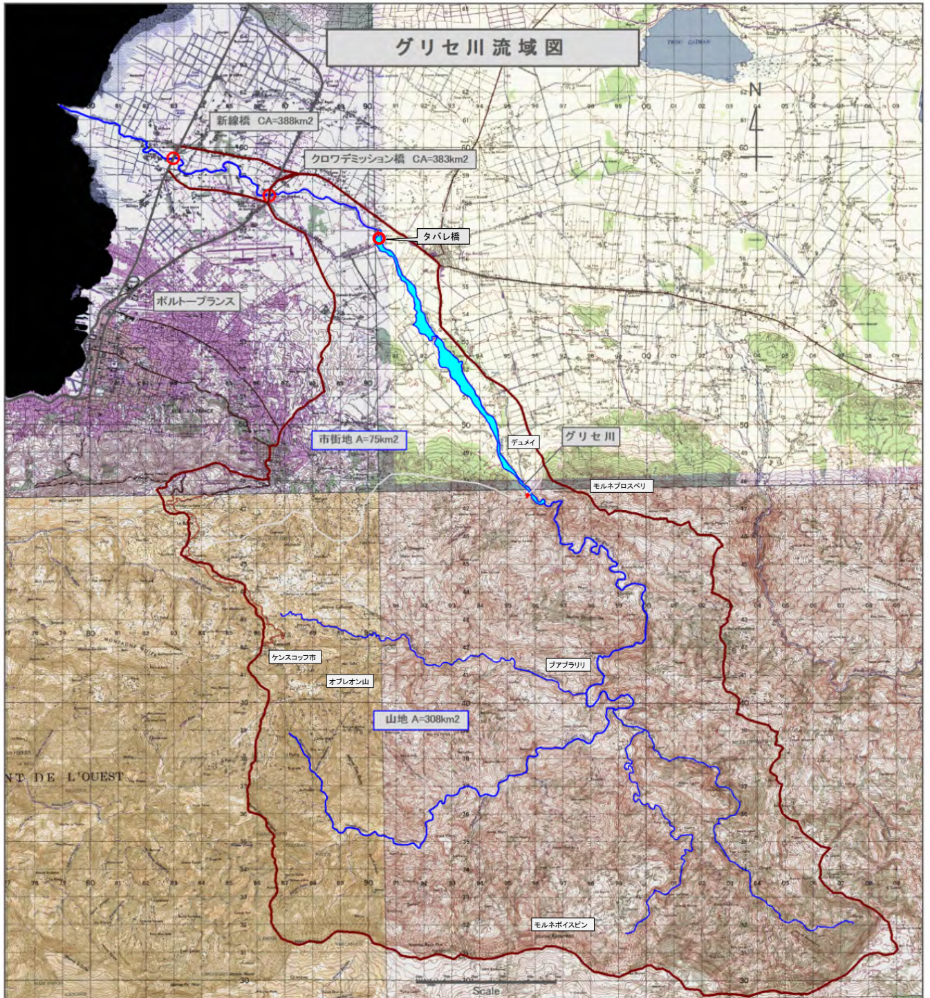
図 2-2-10 グリセ川流域図
