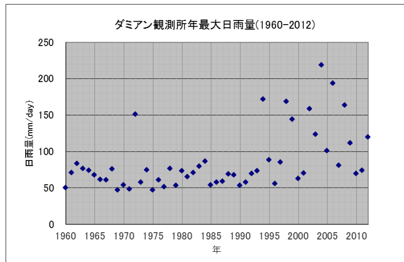
図 2-2-9 年最大日雨量の経年変化
