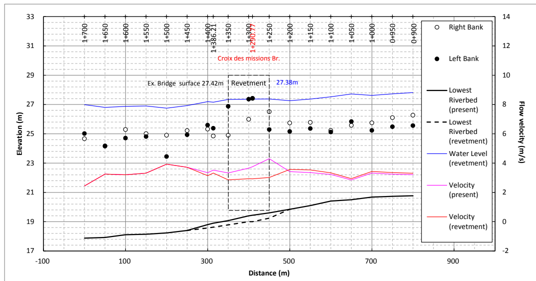
図 2-2-14 河川改修後の水位縦断図（クロワデミッション橋梁）
