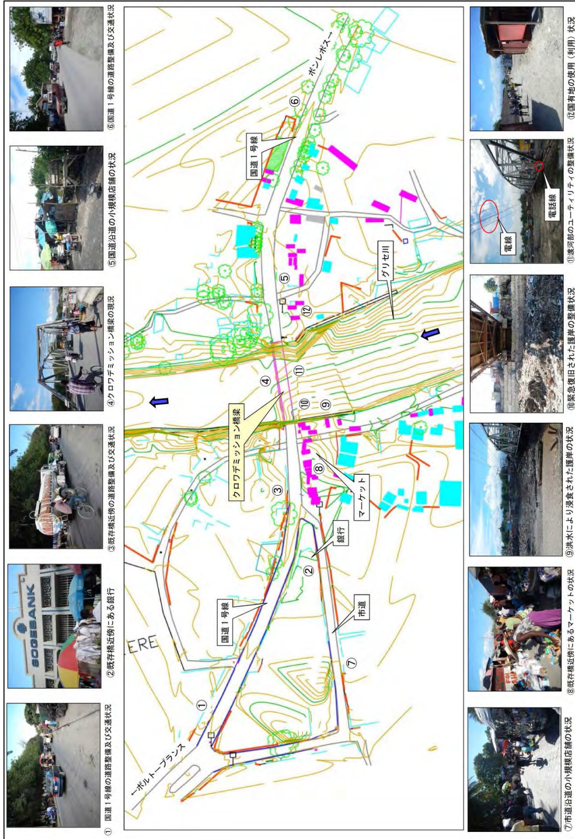
図 2-2-1 国道1号線及びクロワデミッション橋梁の整備状況
