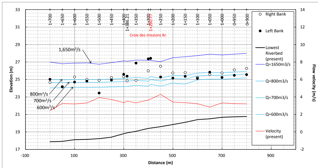
図 2-2-12 現況河道の水位縦断面図（クロワデミッション橋）
