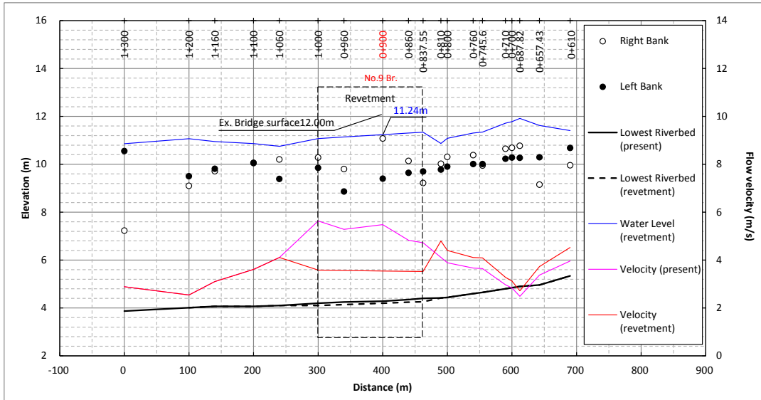
図 2-2-15 河川改修後の水位縦断図（新線橋梁）
