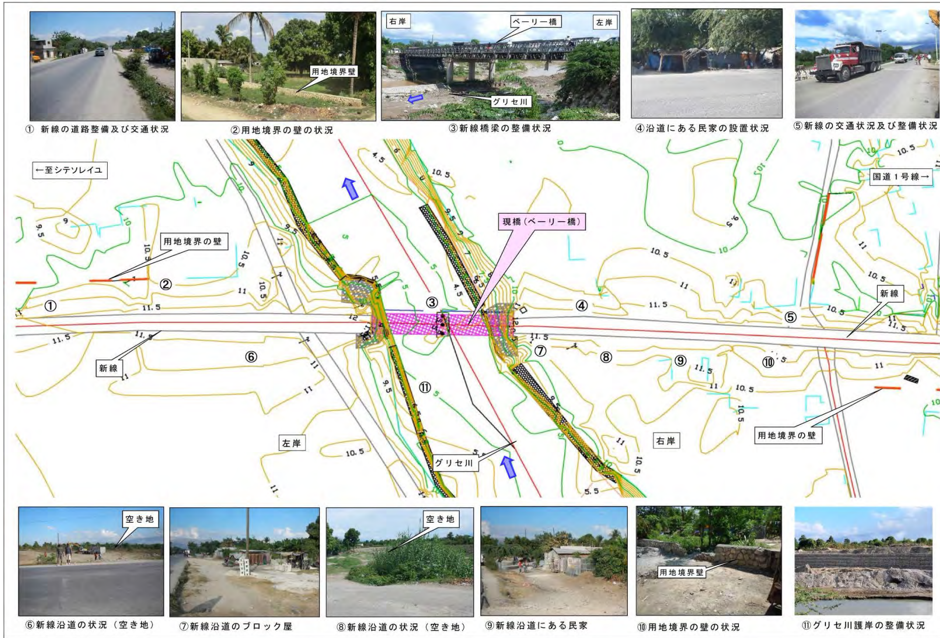
図 2-2-2 新線及び新線橋梁の整備状況
