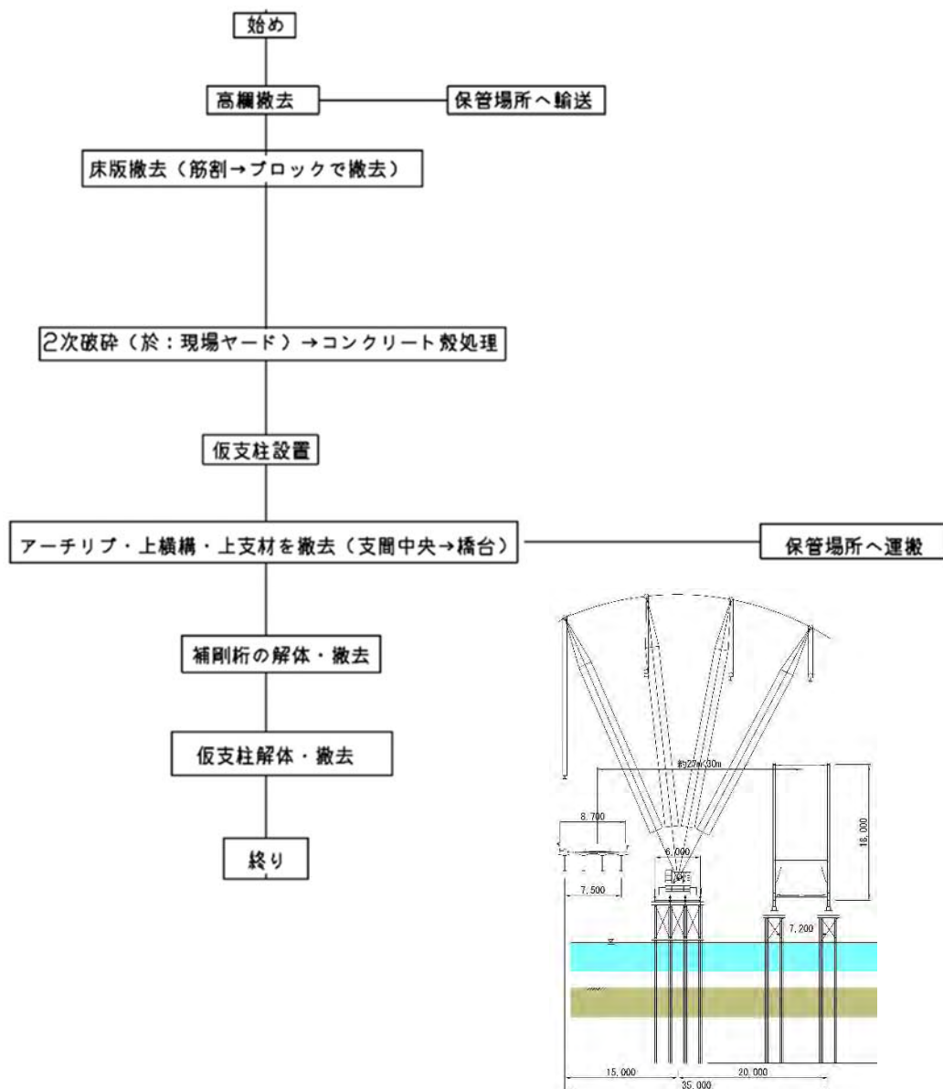
図 3.2.44 カピウラ橋撤去図 (その1)
