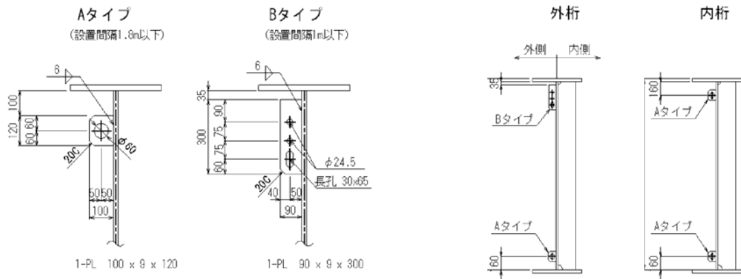
図 3.2.37 吊り金具
