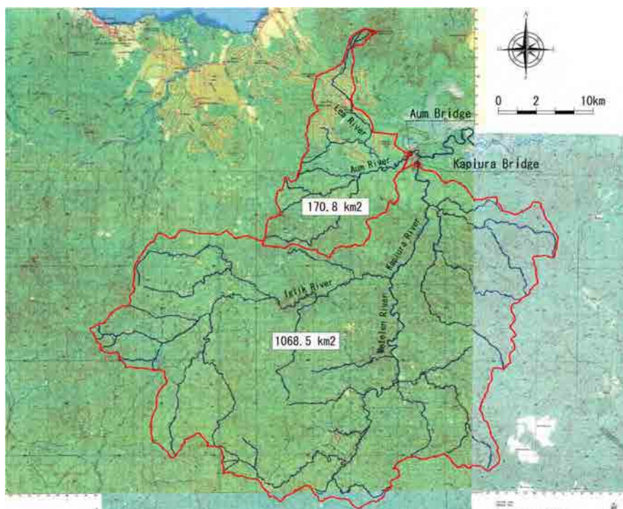
図 3.2.3 流域図
