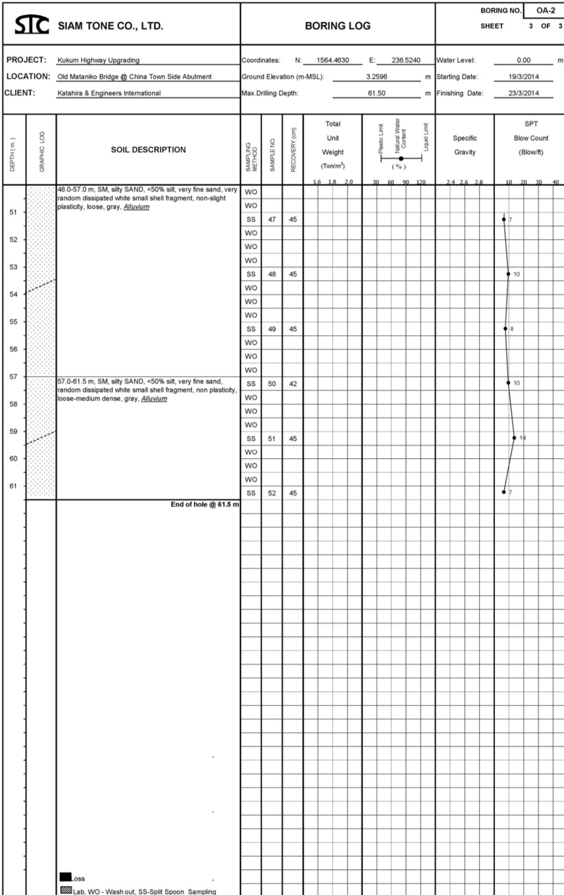
図 12-3-3 (3) ボーリング柱状図 (旧マタニコ橋 OA-2 (BH-3))
