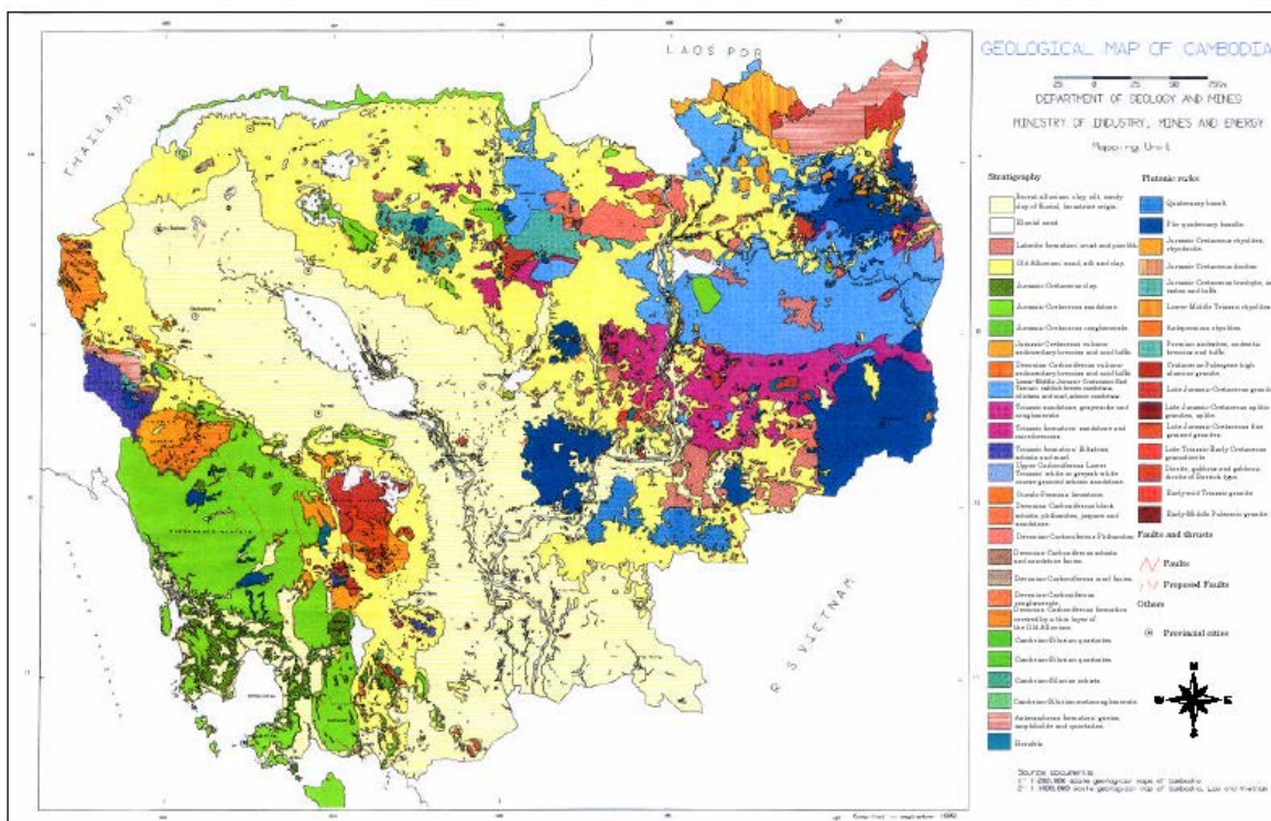
図 7.1-23 「カ」国の地質図
