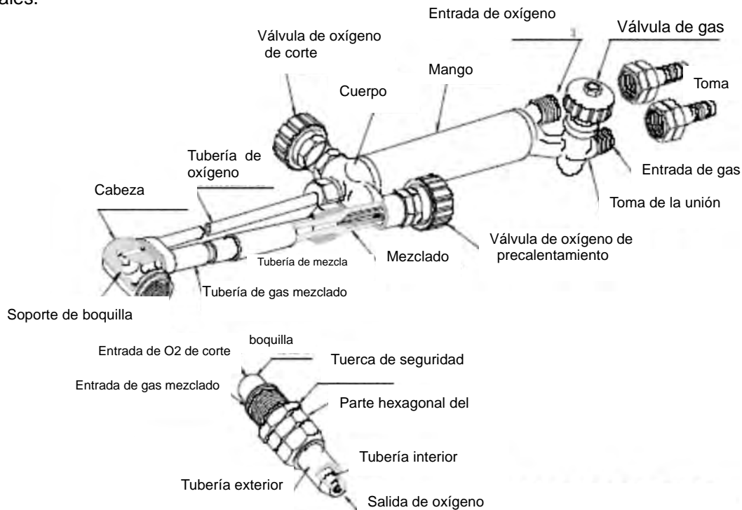
Estructura de cortador
