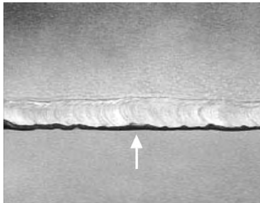
Foto 4: Grieta por baja temperatura generada en la parte influida por el calor de soldadura (Prueba penetrante)
