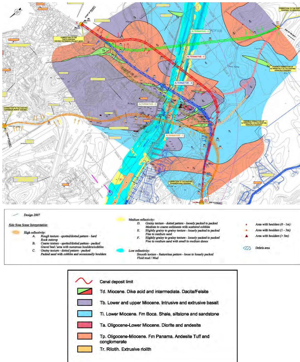
図 4.3 本事業地域の土質状況図
