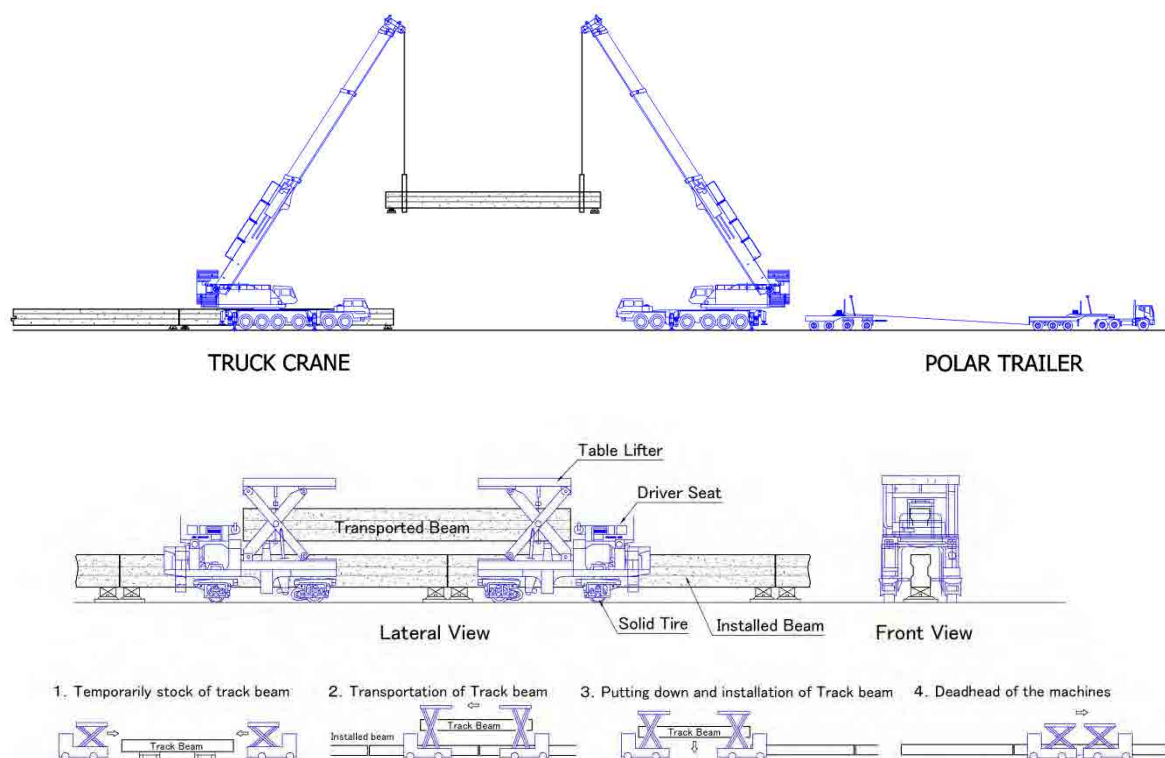
図 8.3 クレーンによる架設と桁運搬架設機
