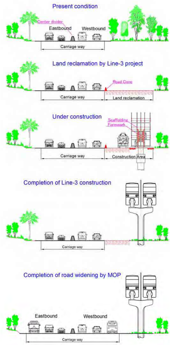
図 8.1 パンアメリカン道路車線拡幅区間工事手順
