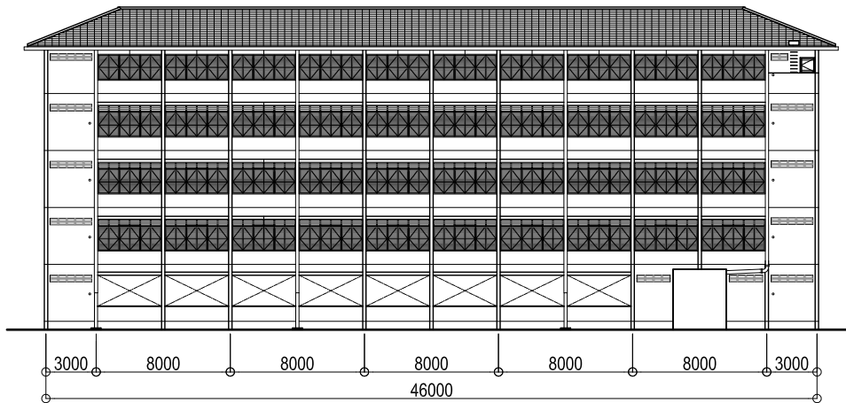
立面図 (教室側)
