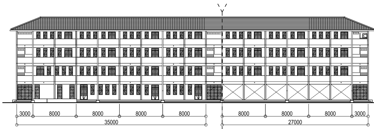
立面図 (廊下側)
