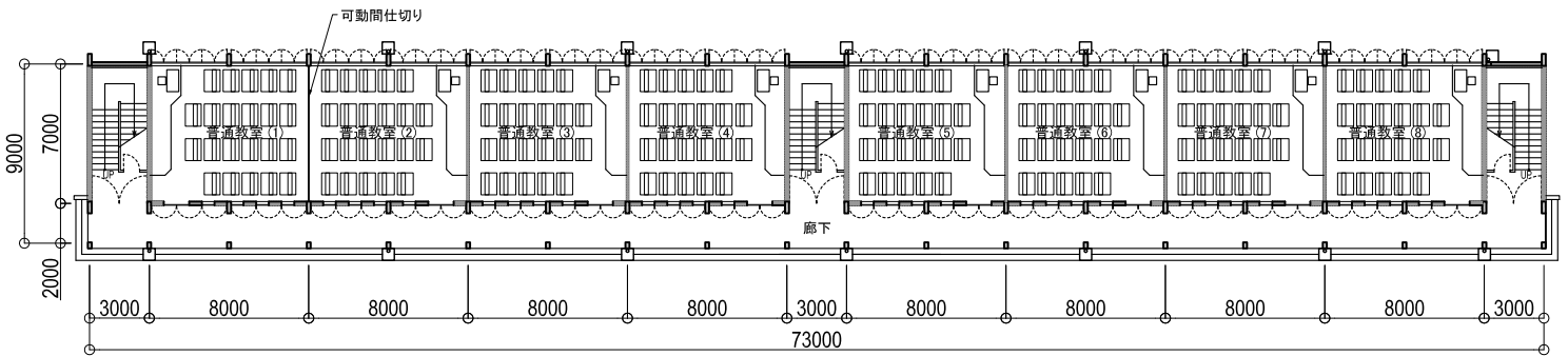
1階 平面図
