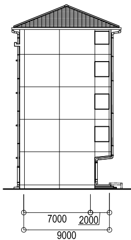
立面図 (妻側)
