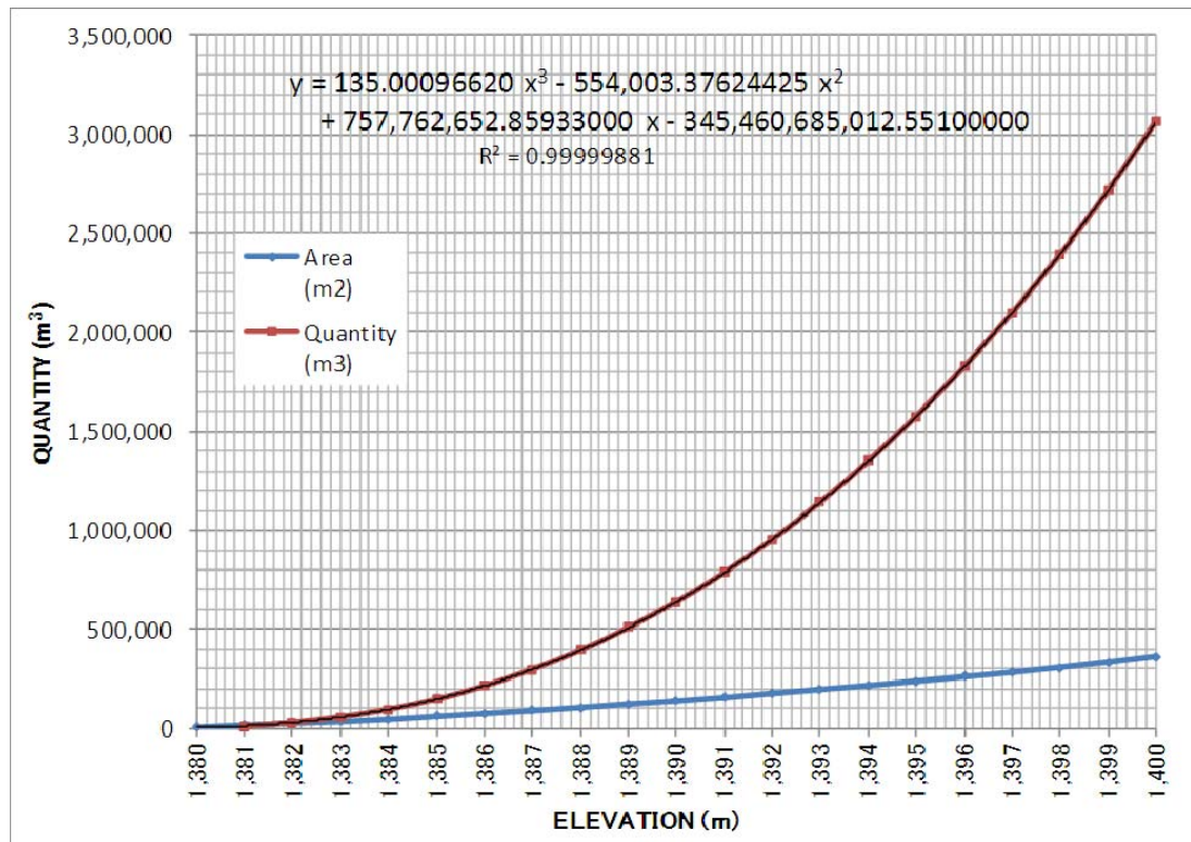
図 3.2.2.11 貯水池の水深と貯水量および湖面面積の関係
