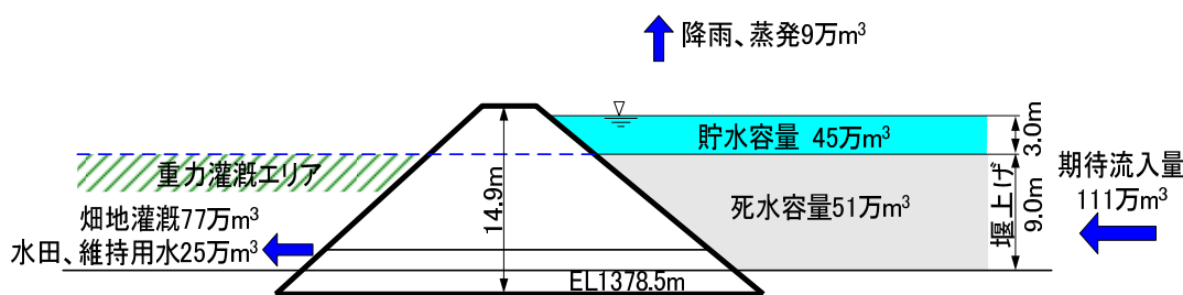
図 3.2.2.14 水収支概念図
