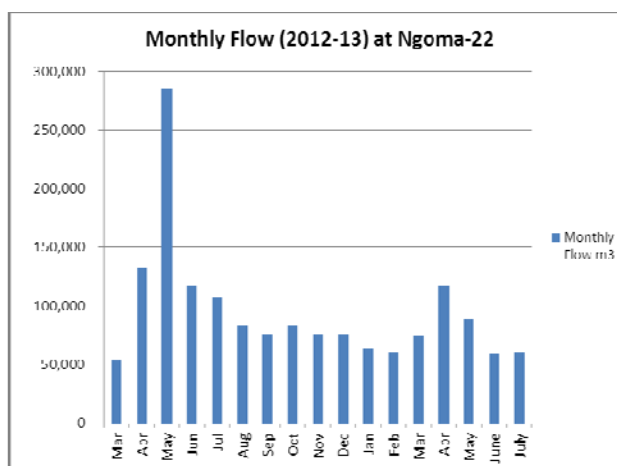
図 3.2.1.3 月毎の河川流量の観測値
