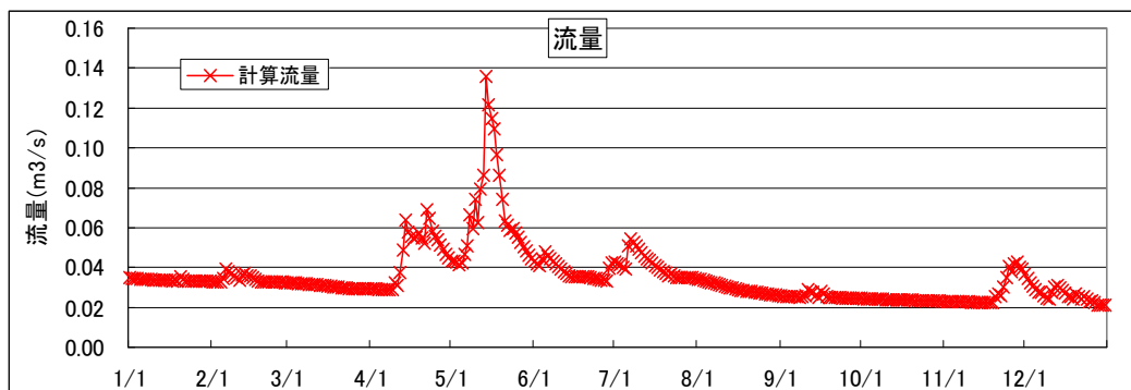
図 3.2.2.7 ダムサイト期待流入量
