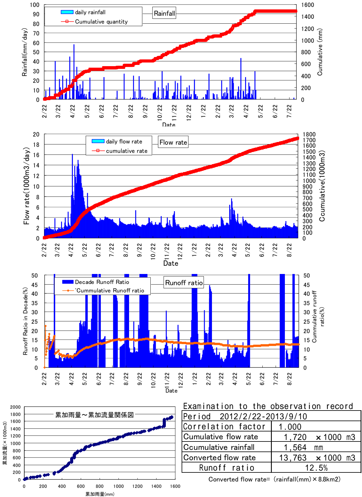
図 3.2.2.1 流量・雨量の観測結果
