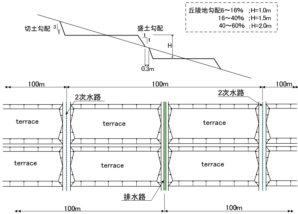
図 3.2.2.16 テラシングの基本構造
