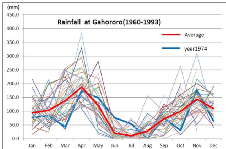
図 3.2.1.2 ガホロロ観測所の雨量記録 (1960～1993年)
