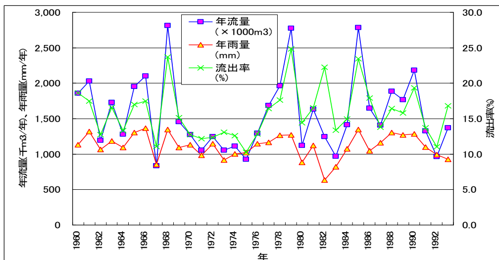
図 3.2.2.5 タンクモデルによる各年流量計算結果
