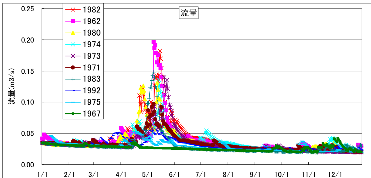
図 3.2.2.12 渇水年のダム地点流入量
