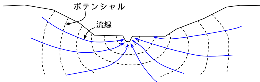
図 3.2.2.8 水田下方浸透水の還元
