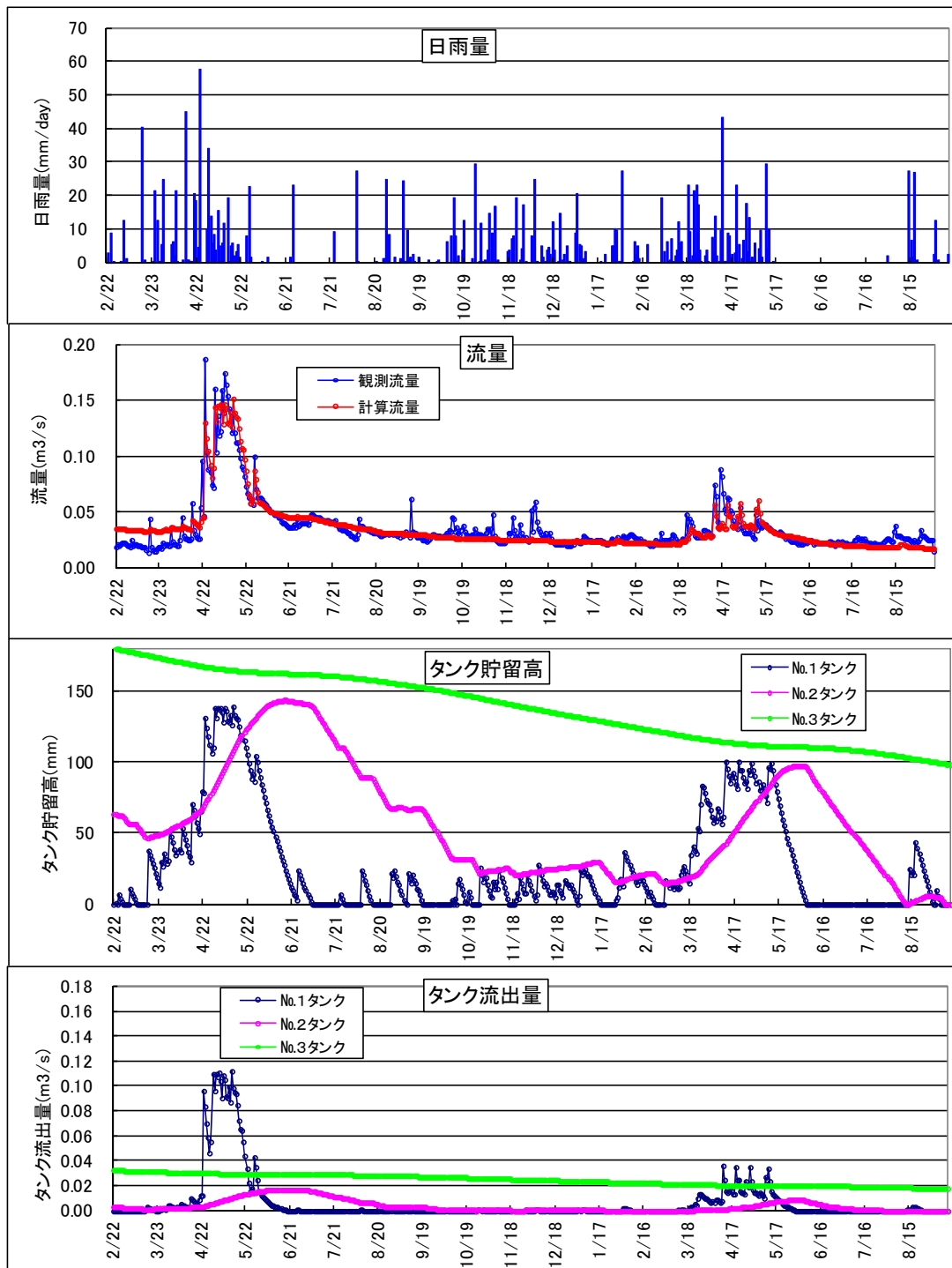
タンクモデル計算結果
