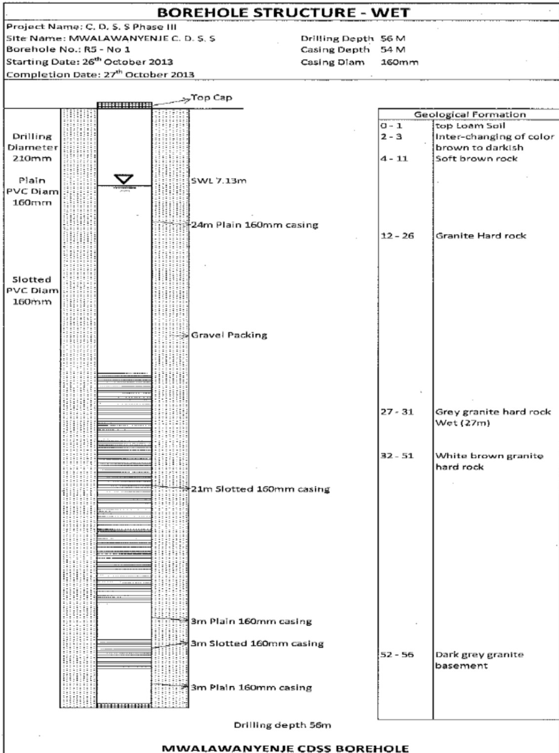
図 2-26 R5 Mwalawanyenje CDSS (No.1) 試掘井戸柱状図
