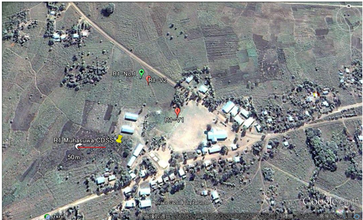
図 2-1 Muhasuwa CDSS 試掘調査位置図
