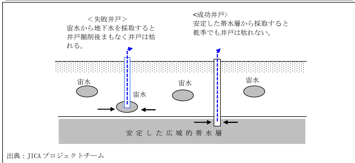
図 8-17 成功井戸と失敗井戸の帯水層の違い
