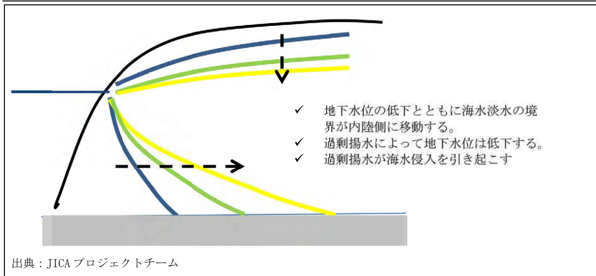
図 8-5 塩水侵入と地下水位の関係
