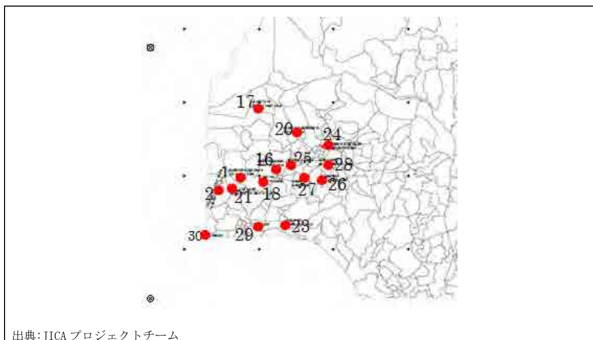
図 4-18 モニタリング浅井戸の位置
