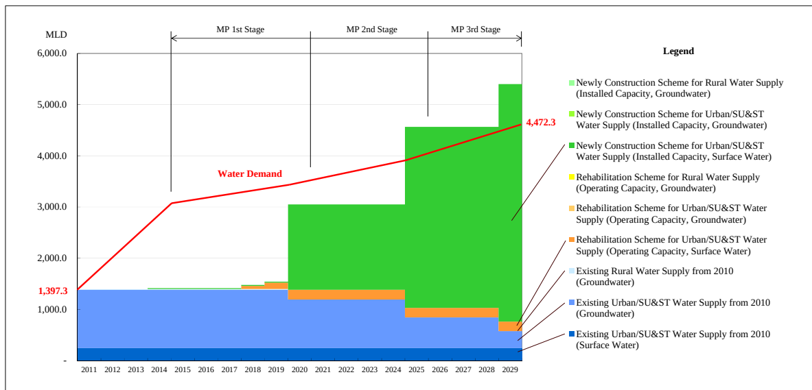
図 7-4 施設計画上の給水開発計画における需要-供給グラフ (Lagos 州、シナリオ B)
