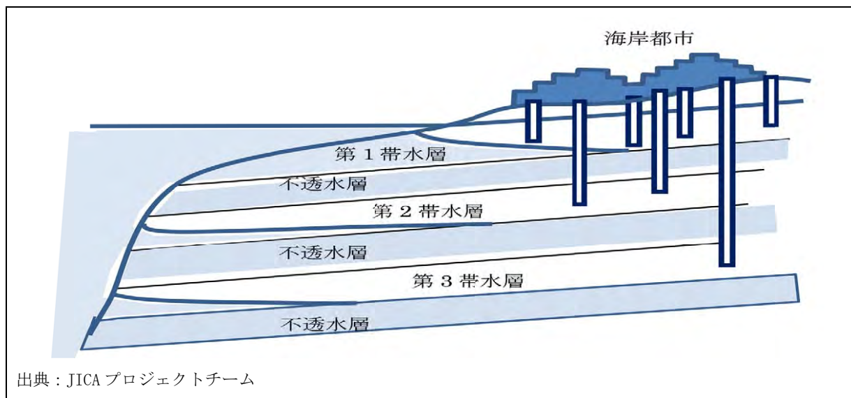
図 8-6 Ogun-Oshun 流域 臨界都市における帯水層と海水侵入の状況
