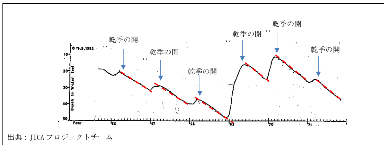
図 8-19 地下水位変動のパターン
