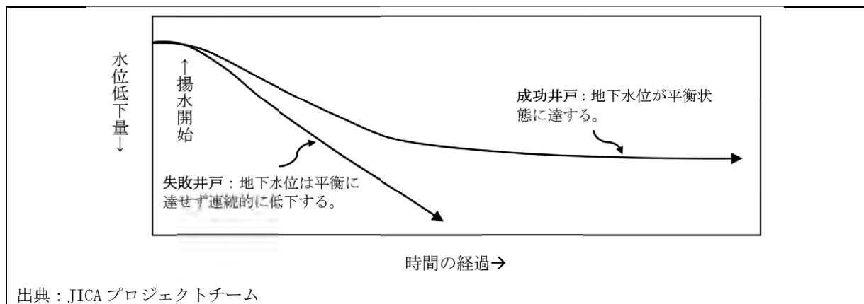
図 8-18 成功井戸と失敗井戸の揚水試験結果
