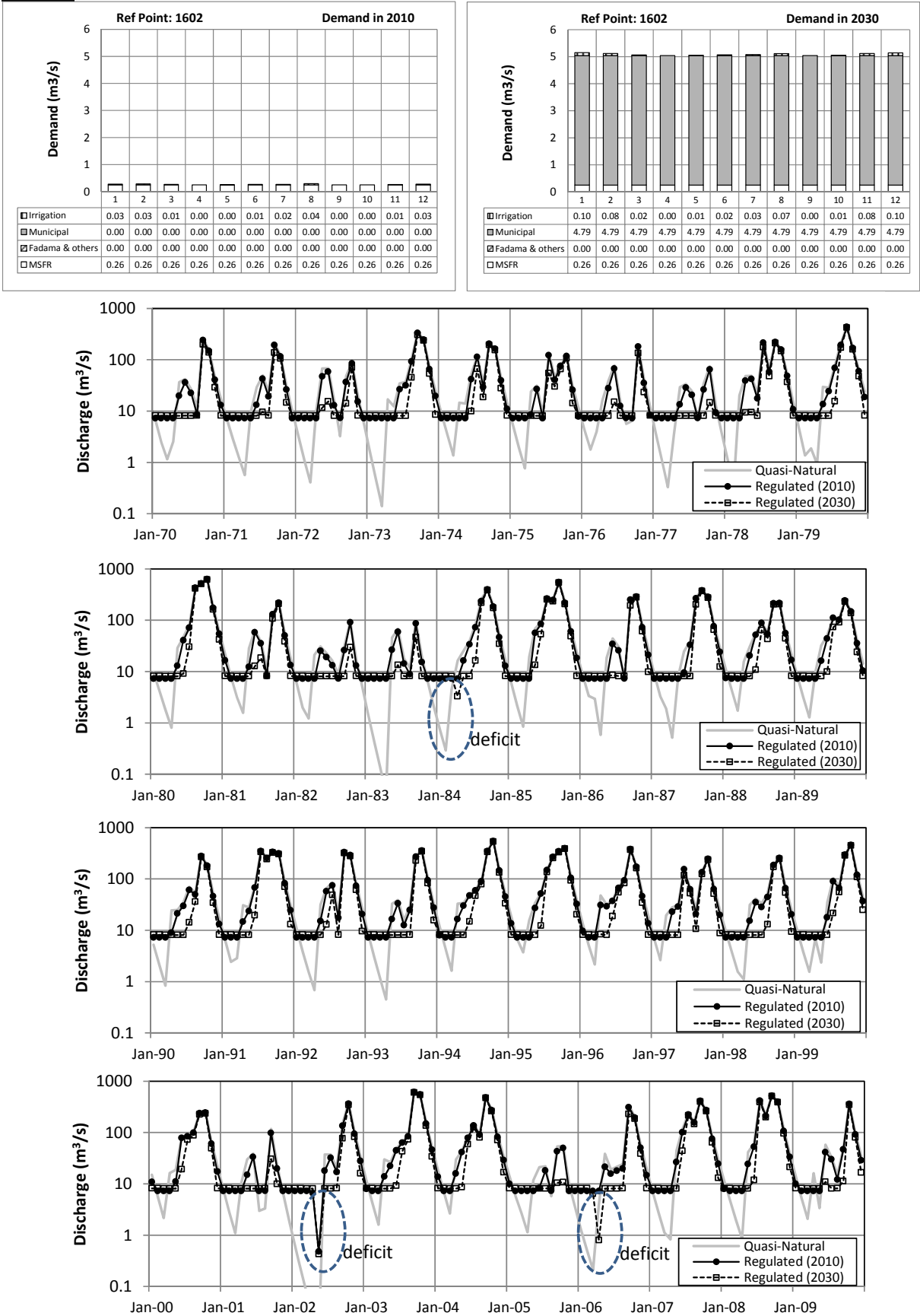
付図 5-1 代表地点における水バランス (2/2)
