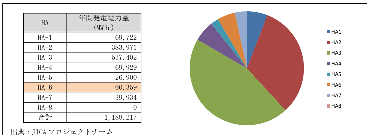
図 7-9 HA 毎の年間発電電力量（賦存量）
