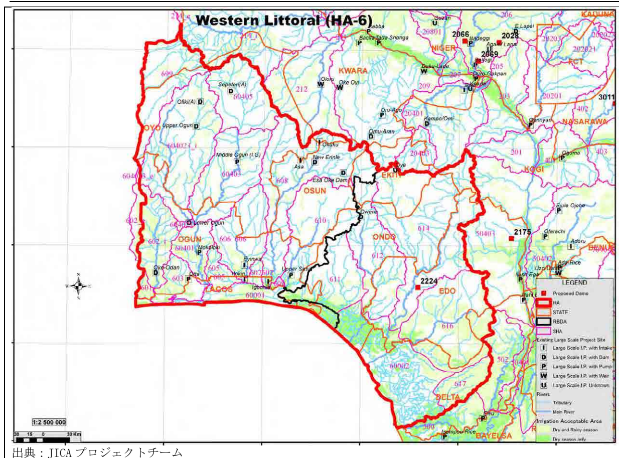
図 7-8 灌漑計画 (HA-6)
