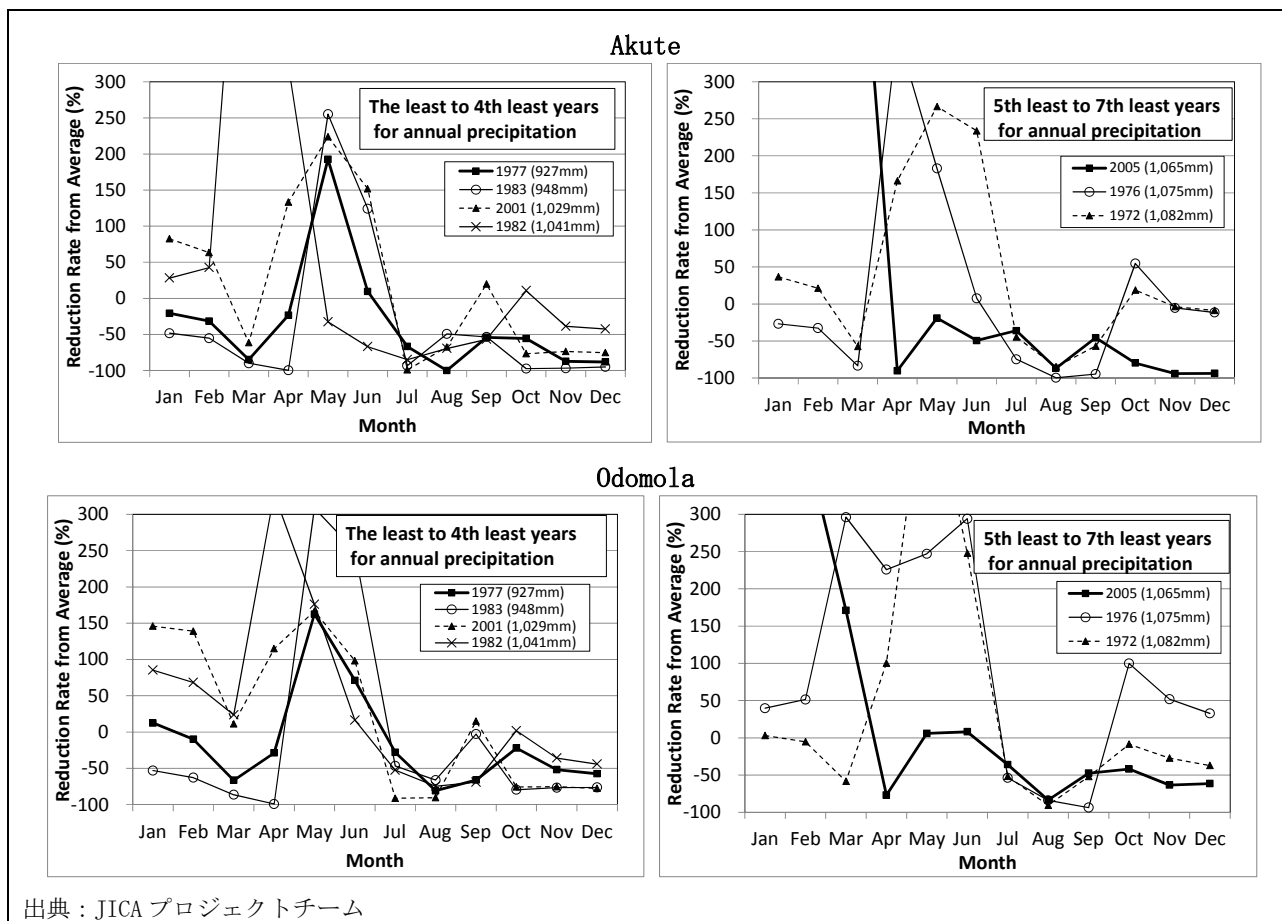
図 4-14 少雨年における月ごとの流量減少率
