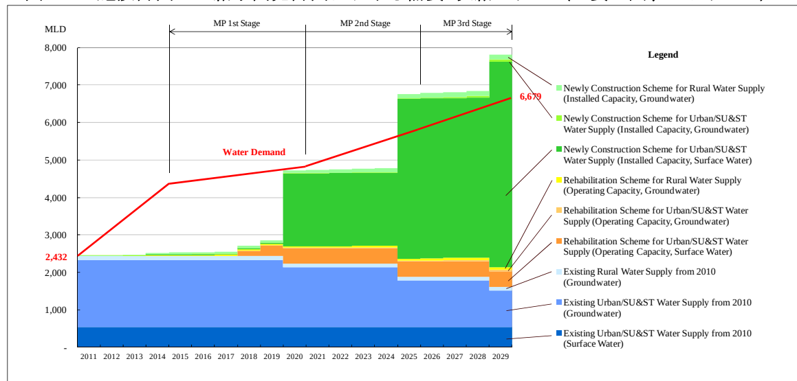
図 7-1 施設計画上の給水開発計画における需要-供給グラフ（主要 4 州、シナリオ A）
