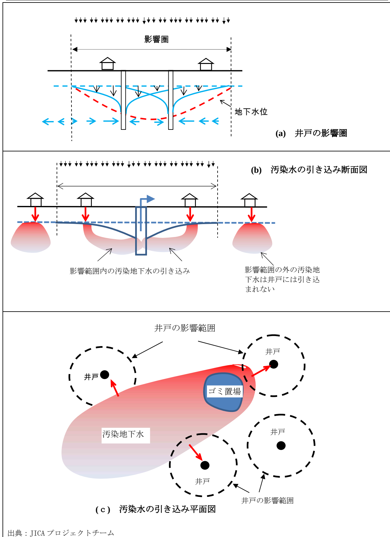
図 8-12 影響圏内の汚染地下水による地下水汚染のメカニズム
