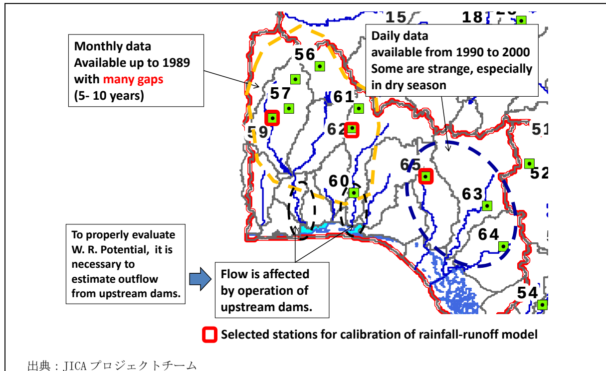
図 4-8 HA-6 における利用可能な水文データ
