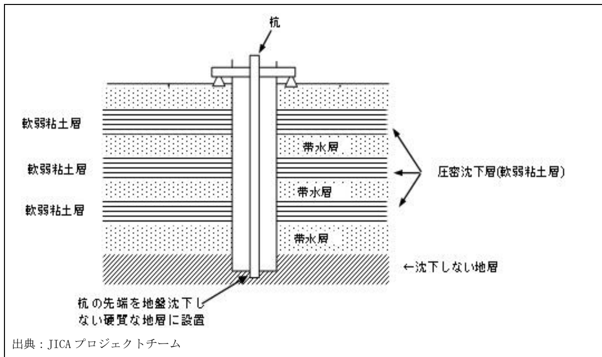
図 8-9 地盤沈下観測井戸の例
