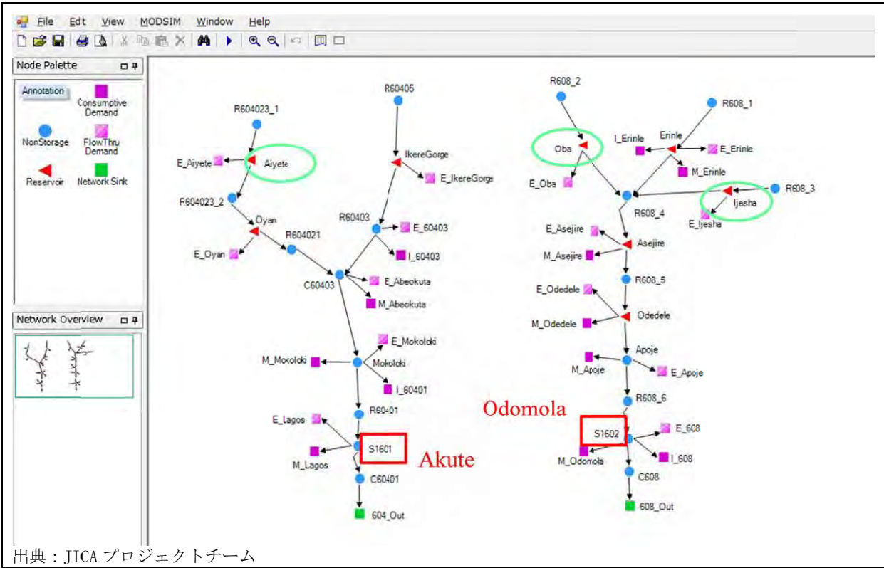
図 5-10 Ogun-Oshun 流域における MODSIM-DSS によるモデルネットワーク (シナリオ B)
