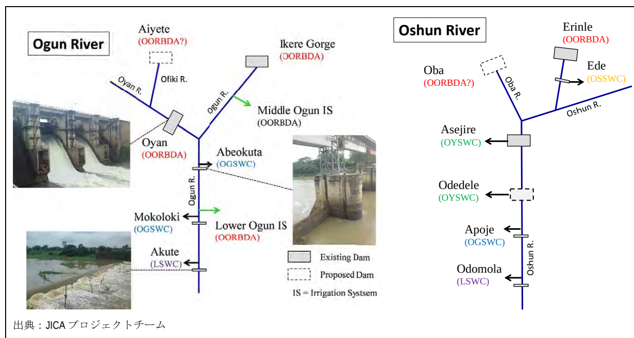
図 6-8 Ogun-Oshun 流域の主要ダムと主要取水施設
