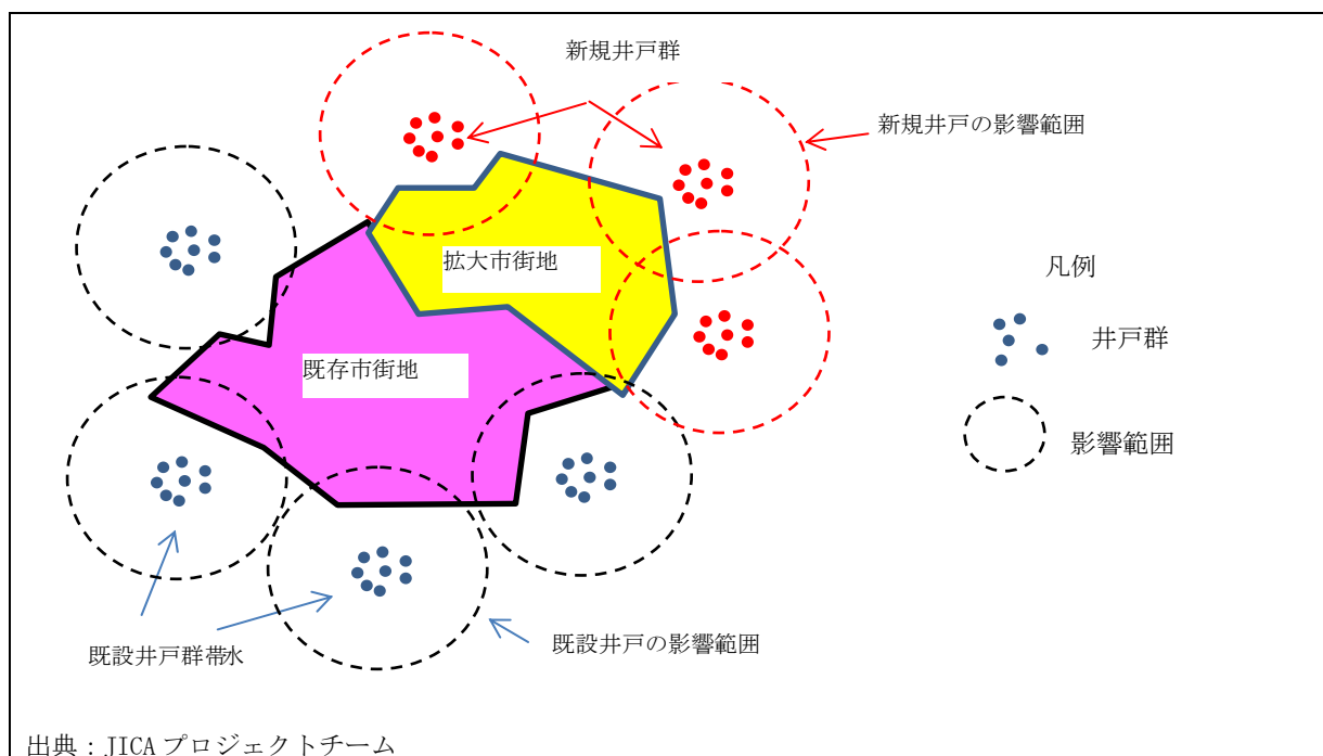
図 6-3 井戸群による給水のイメージ
