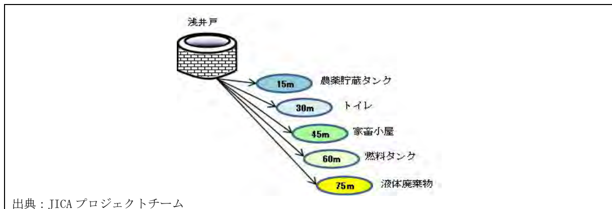
図 8-13 地下水汚染を防ぐための井戸と汚染源との距離の例
