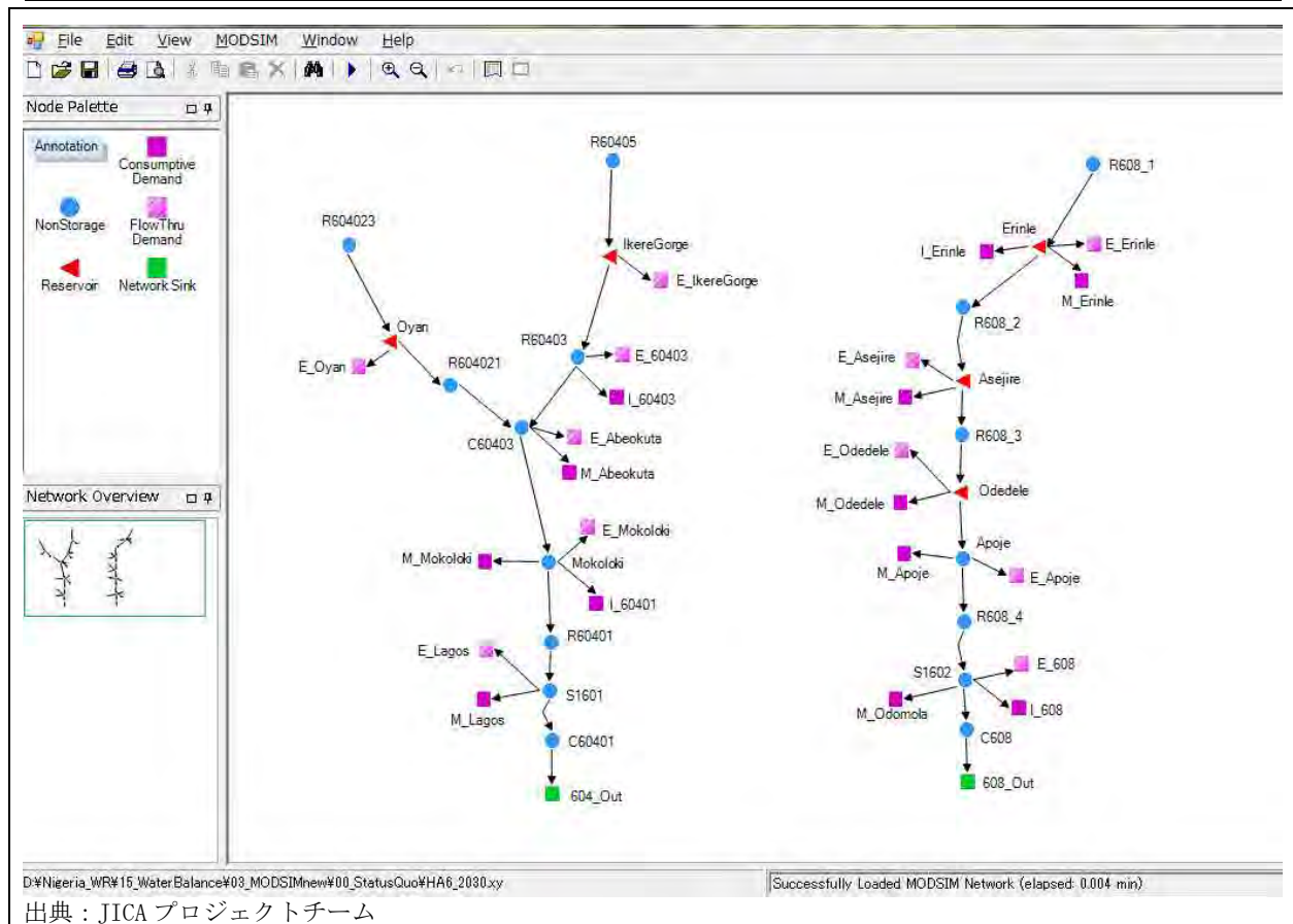
図 5-8 Ogun-Oshun 流域における MODSIM-DSS によるモデルネットワーク (シナリオ A)
