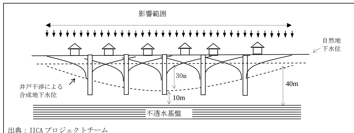
図 6-2 風化帯水層の揚水限界のイメージ
