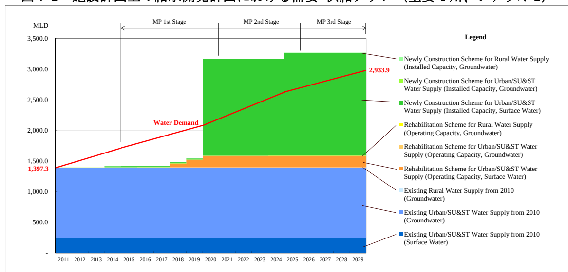
図 7-2 施設計画上の給水開発計画における需要-供給グラフ（主要 4 州、シナリオ B）
