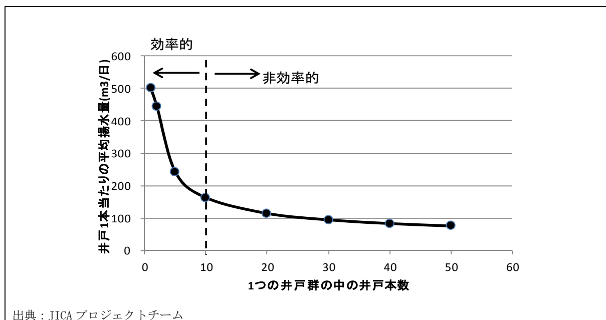
図 6-5 井戸群の井戸本数と揚水量の関係の例
