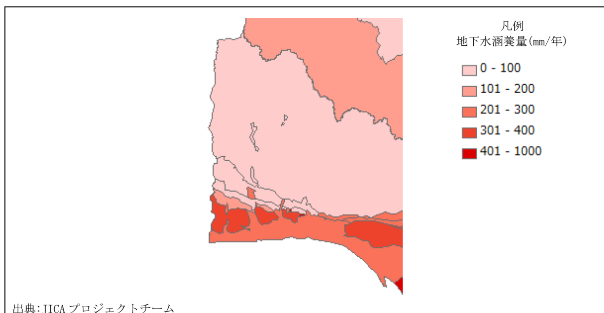
図 4-17 解析結果の帯水層ごとの地下水涵養量分布
