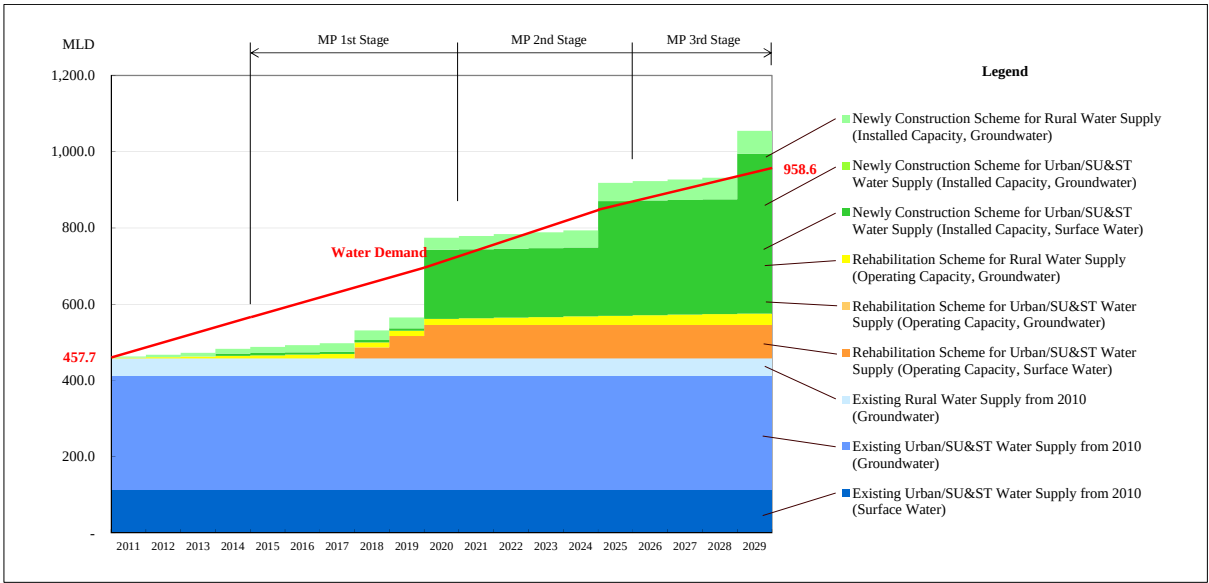
図 7-7 施設計画上の給水開発計画における需要-供給グラフ（Oyo 州）
