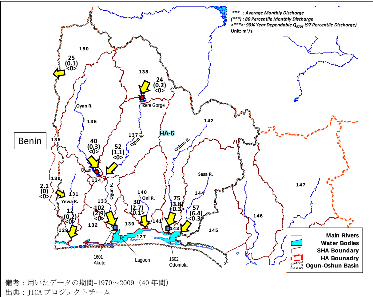
図 4-11 平均月流量、 Q_{80M} および Q_{97DS}90\%Y
