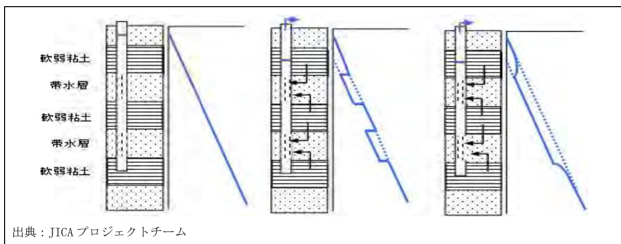
図 8-8 地盤沈下のメカニズム（軟弱粘土層の地下水絞りだし）
