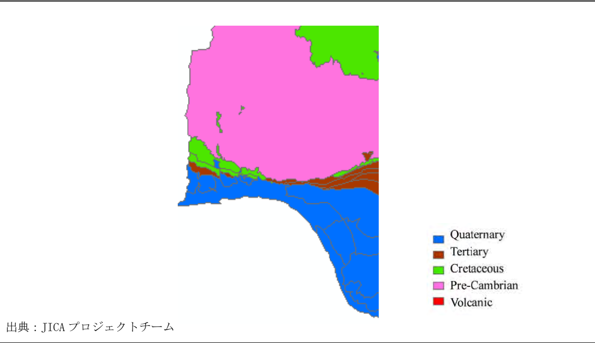
図 1-4 Ogun-Oshun 流域の地質概略
