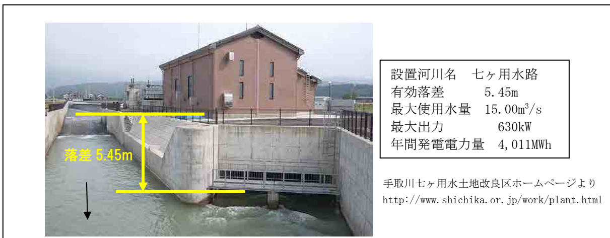
図 7-10 日本における低落差の発電所の事例
