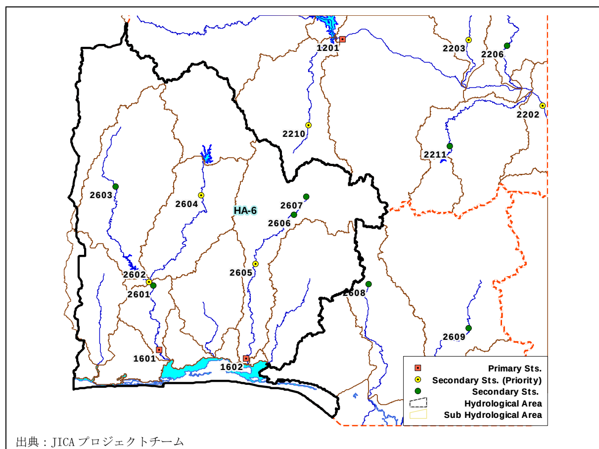
図 8-20 Ogun-Oshun 流域における提案表流水観測所
