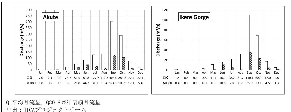
図 4-13 代表地点における流量の季節変動 (1/2)
