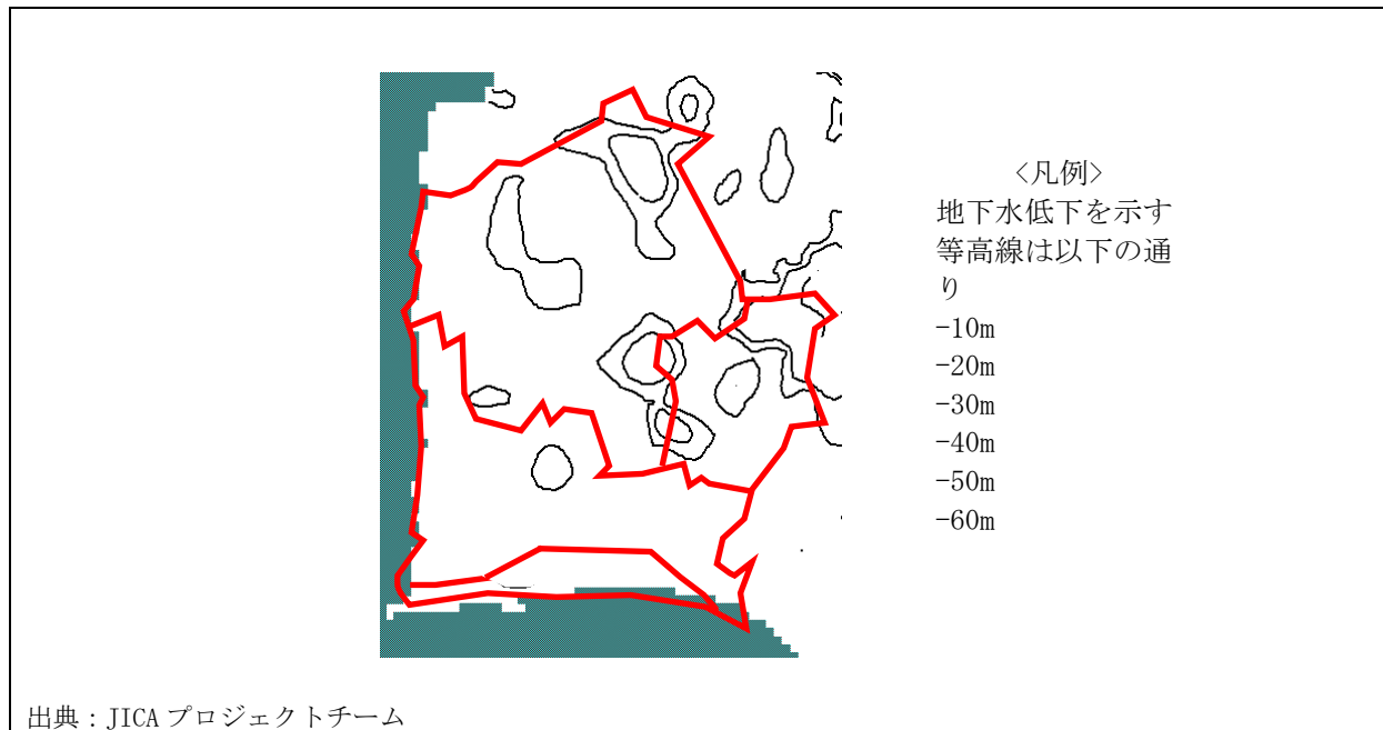
図 5-6 気候変動の影響を考慮した 2030 年における広域的地下水位低下の予測
