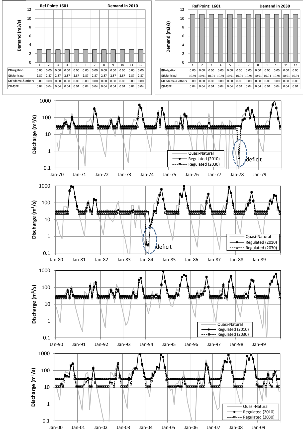
付図 5-1 代表地点における水バランス (1/2)
