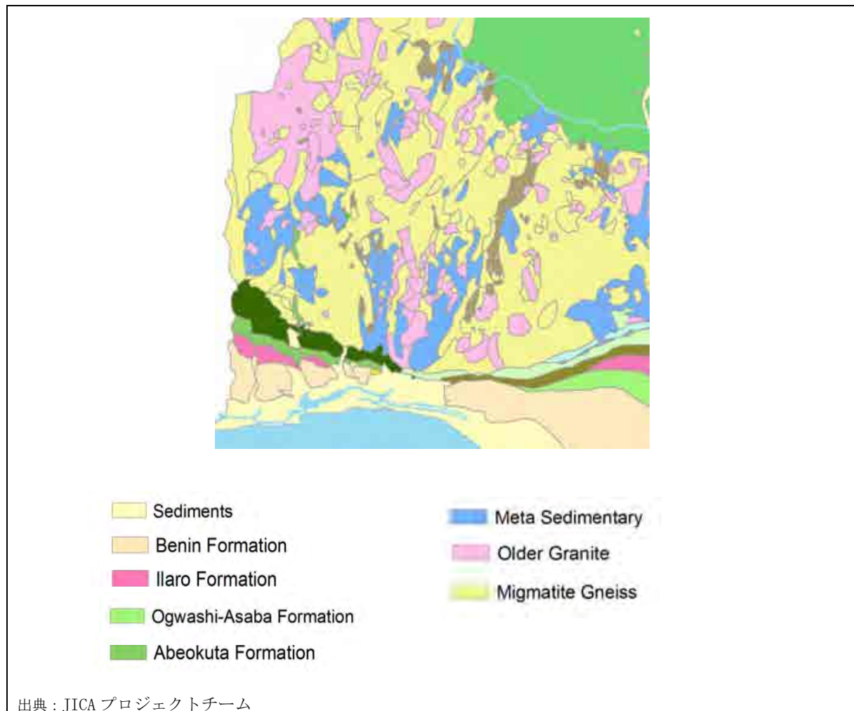
図4-16 Ogun-Oshun流域の地質図
