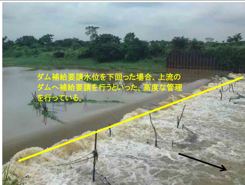
写真 8-1 Ogun-Oshun 流域における下流の取水堰堤 (ダム補給要請開始水位を設定した管理を行っている)
