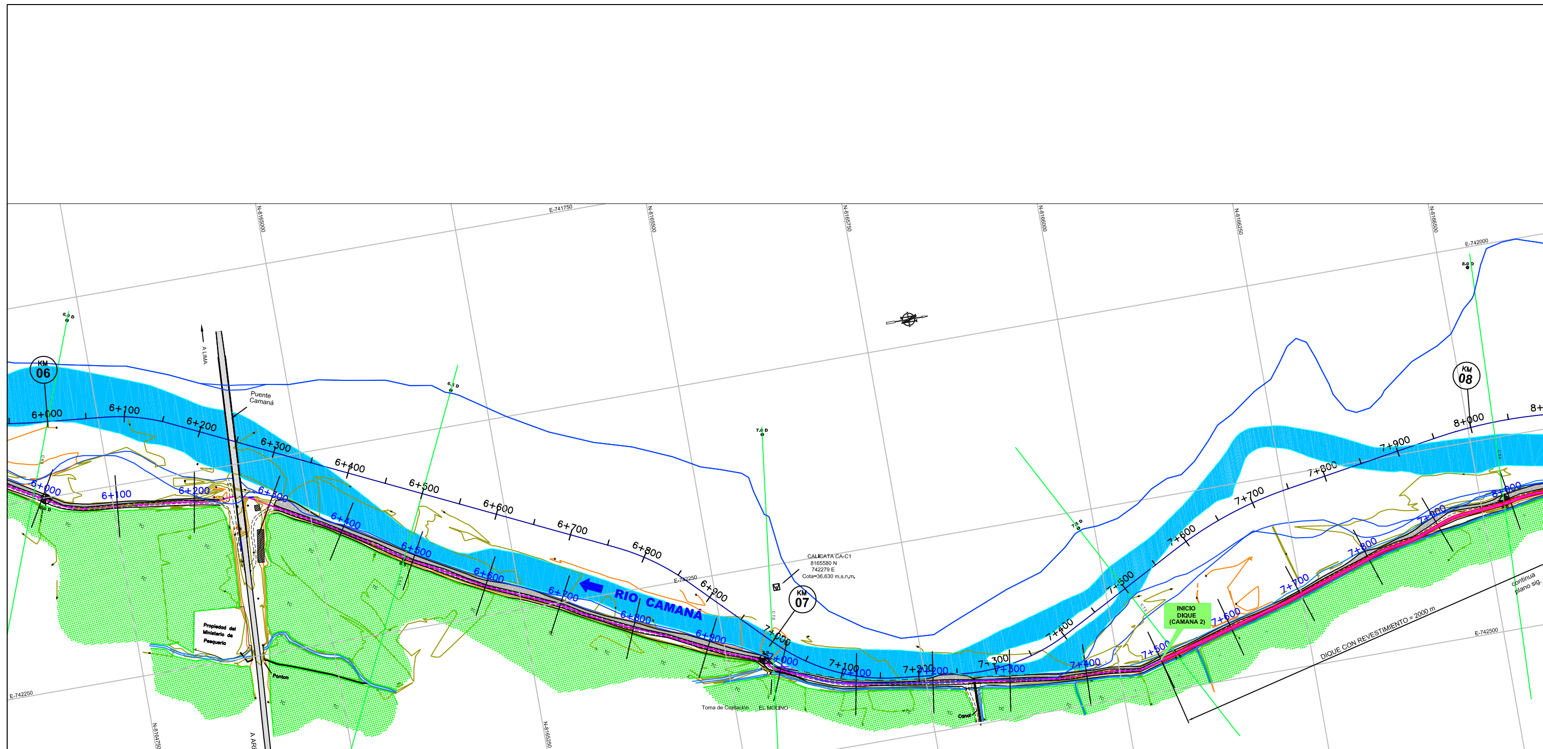
PLANTA Esc: 1/2,500
