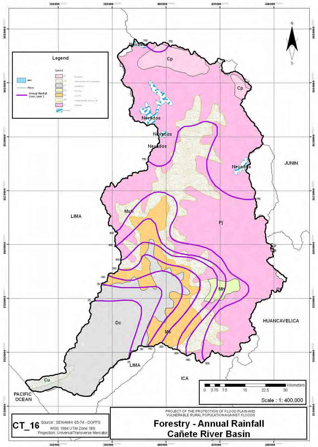
Apéndice 7-Figura 3.1 Precipitación anual y distribución de la vegetación (Cuenca del río Cañete)
