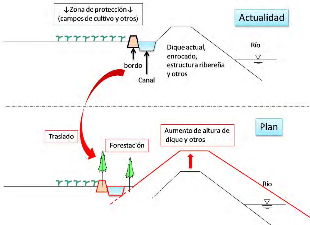
Figura 3.1-1 Diagrama Conceptual Forestación a lo largo de las estructuras ribereñas (Tipo A)
