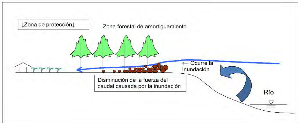
Figura 3.1-1 Diagrama Conceptual Forestación a lo largo de las estructuras ribereñas (Tipo A)
