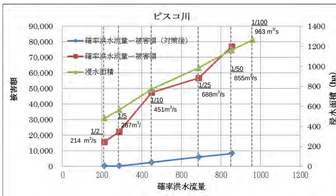
図-4.3.1-2 確率洪水規模流量と被害額および浸水面積（ピスコ川）
