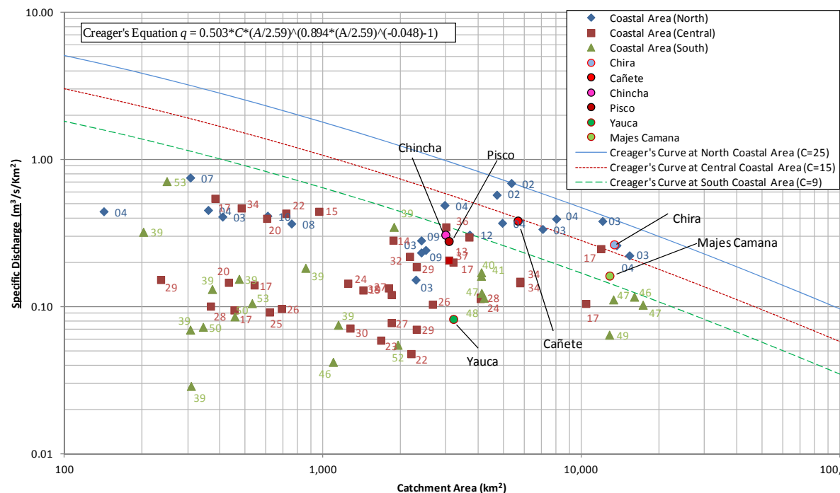
図-3.1.9.5-3 ペルー海岸域の地域別の確率洪水比流量図と本調査での確率洪水流量（50年確率）
