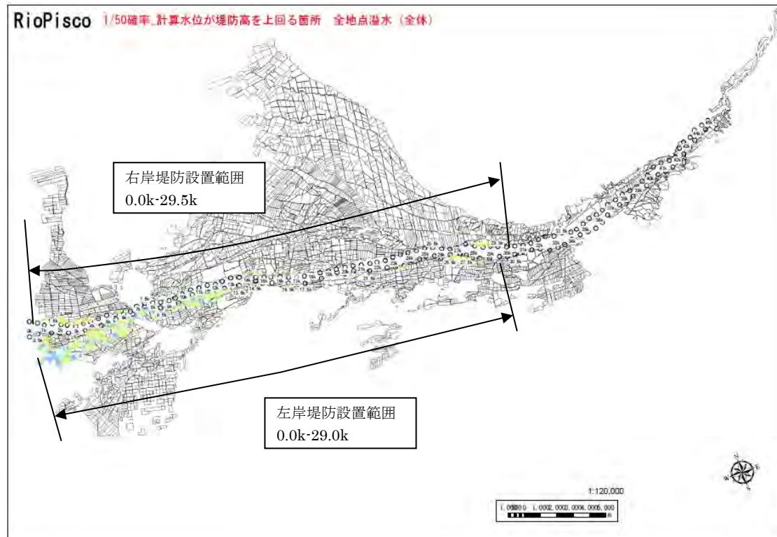
図-4.15.1-4 ピスコ川の堤防設置範囲
