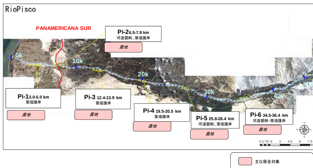
図-4.3.1-4 ピスコ川における重点洪水対策施設の位置
