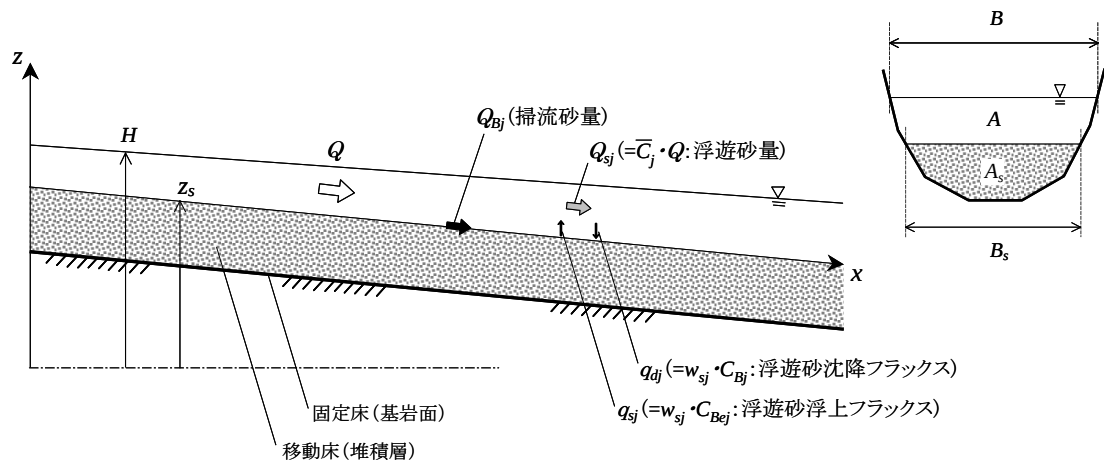
図-4.15.1-5 河床変動解析モデルの概念図
