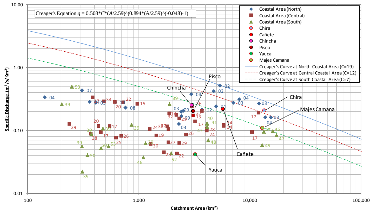
図-3.1.9.5-2 ペルー海岸域の地域別の確率洪水比流量図と本調査での確率洪水流量（20年確率）
