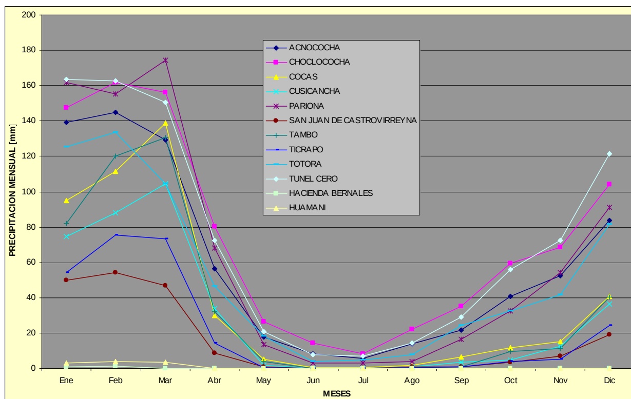
図 - 3.1.9.1-2 ピスコ川流域およびその近傍の流域における月平均降雨量の分布 (mm)
