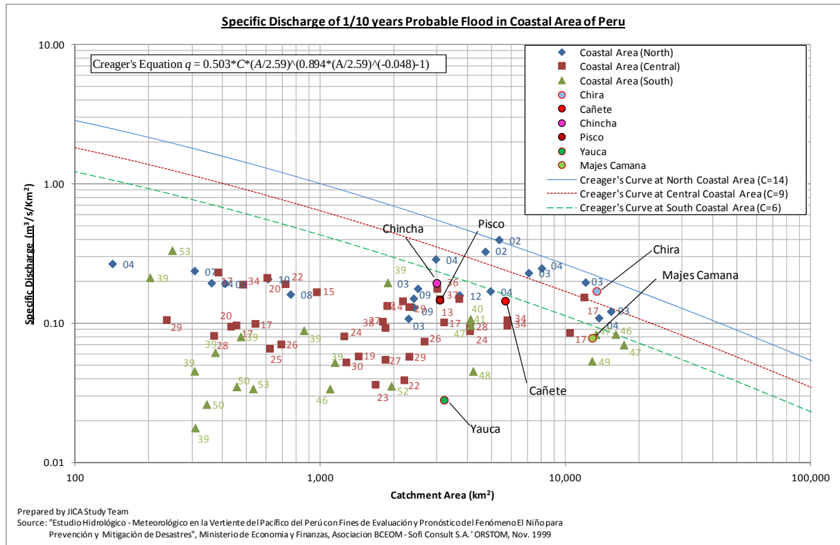
図-3.1.9.5-1 ペルー海岸域の地域別の確率洪水比流量図と本調査での確率洪水流量（10年確率）
