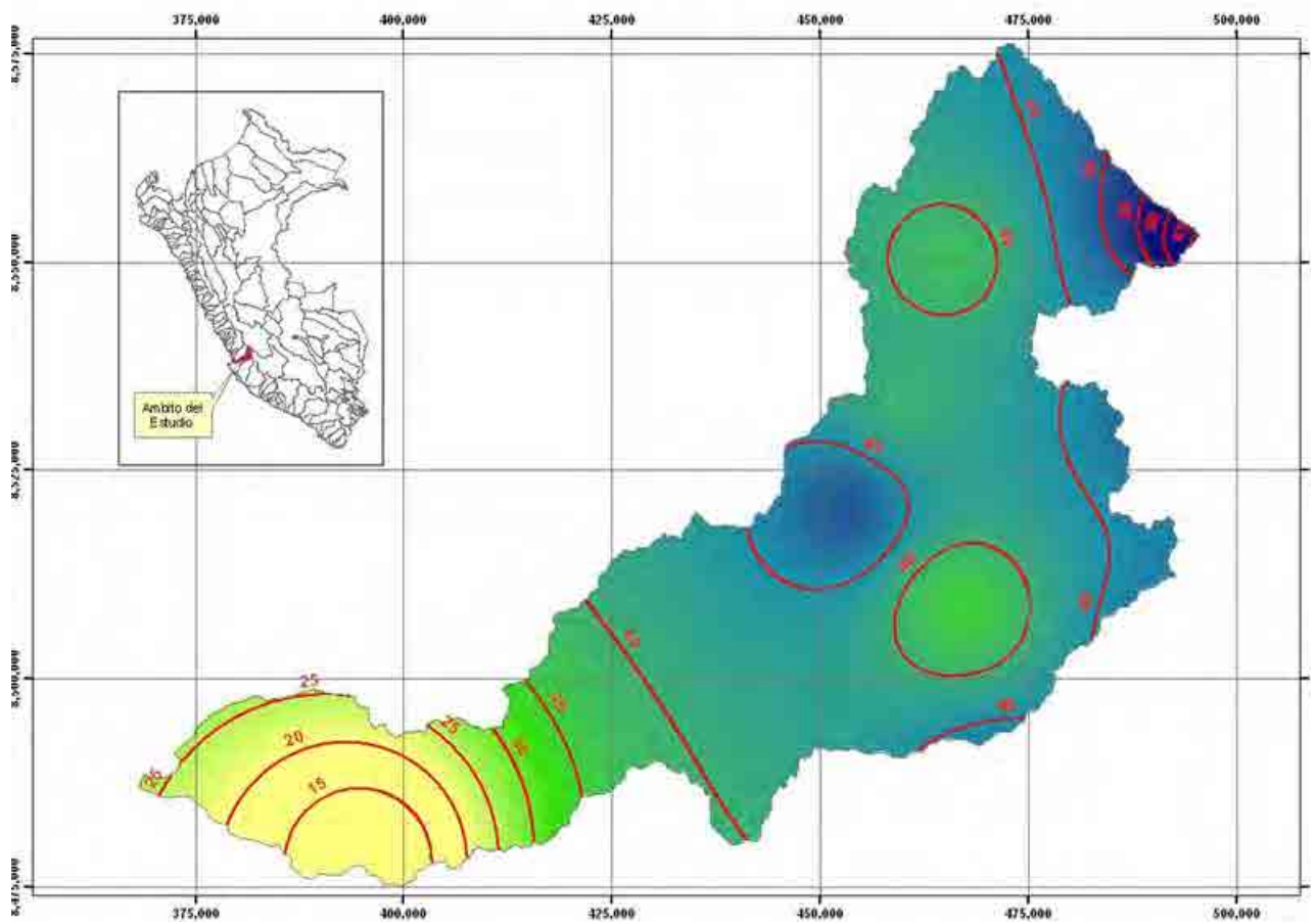
図-3.1.9.4-3 確率 50 年規模の 24 時間降雨量の等雨量線図 (ピスコ川)
