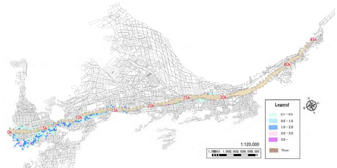
図-3.1.10-4 ピスコ川氾濫範囲（確率 50 年規模の洪水）
