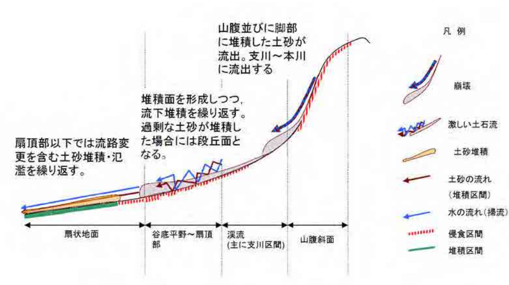
図-3.1.8-14 大規模出水時の土砂生産流出の状態（地質学的スケール）
