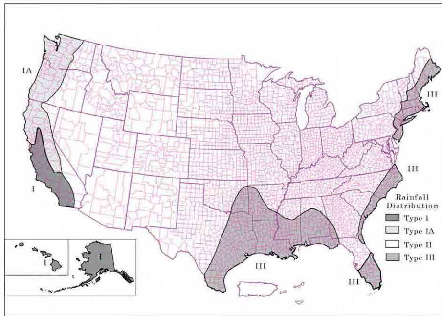
図-3.1.9.4-6 USA における 24 時間降雨量曲線のタイプと適用地域
