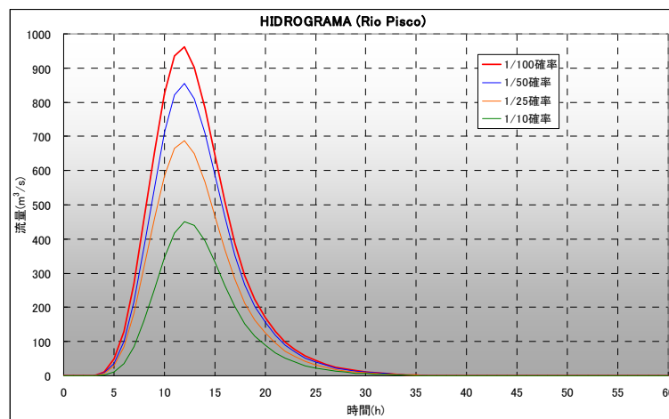
図-3.1.9.4-8 ピスコ川の洪水ハイドログラフ
