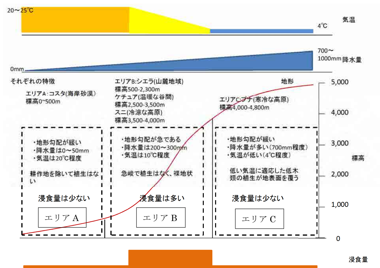
図-3.1.8-6 流域特性
