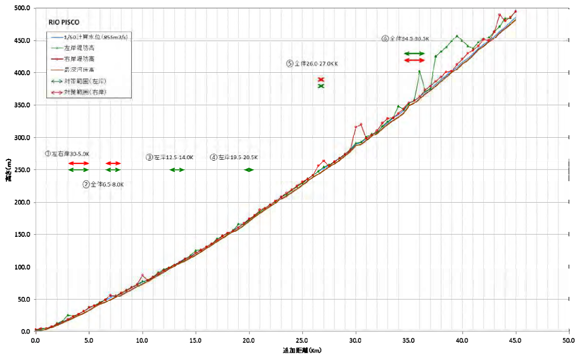
図-4.15.1-3 ピスコ川縦断面図
