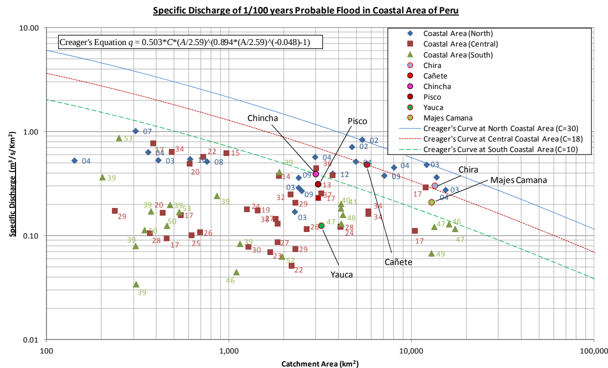
図-3.1.9.5-4 ペルー海岸域の地域別の確率洪水比流量図と本調査での確率洪水流量（100年確率）
