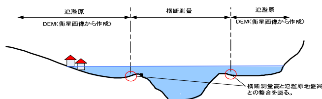
図-3.1.10-1 一次元モデルのイメージ
