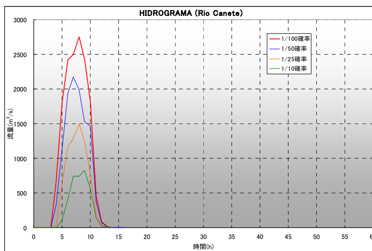
図-3.1.9.4-8 カニエテ川の洪水ハイドログラフ
