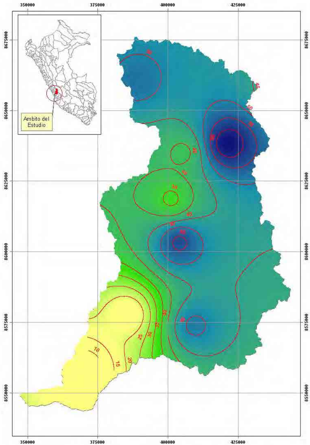
図-3.1.9.4-3 確率 50 年規模の 24 時間降雨量の等雨量線図 (カニェテ川)
