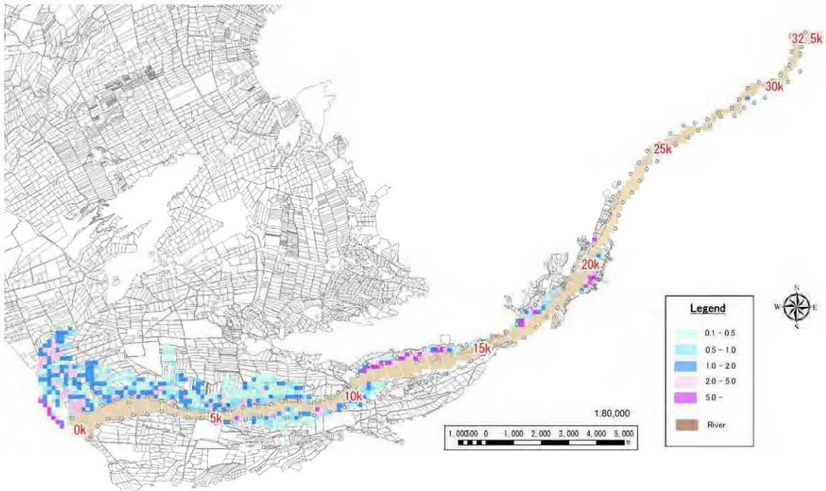
図-3.1.10-4 カニェテ川氾濫範囲 (確率 50 年洪水)
