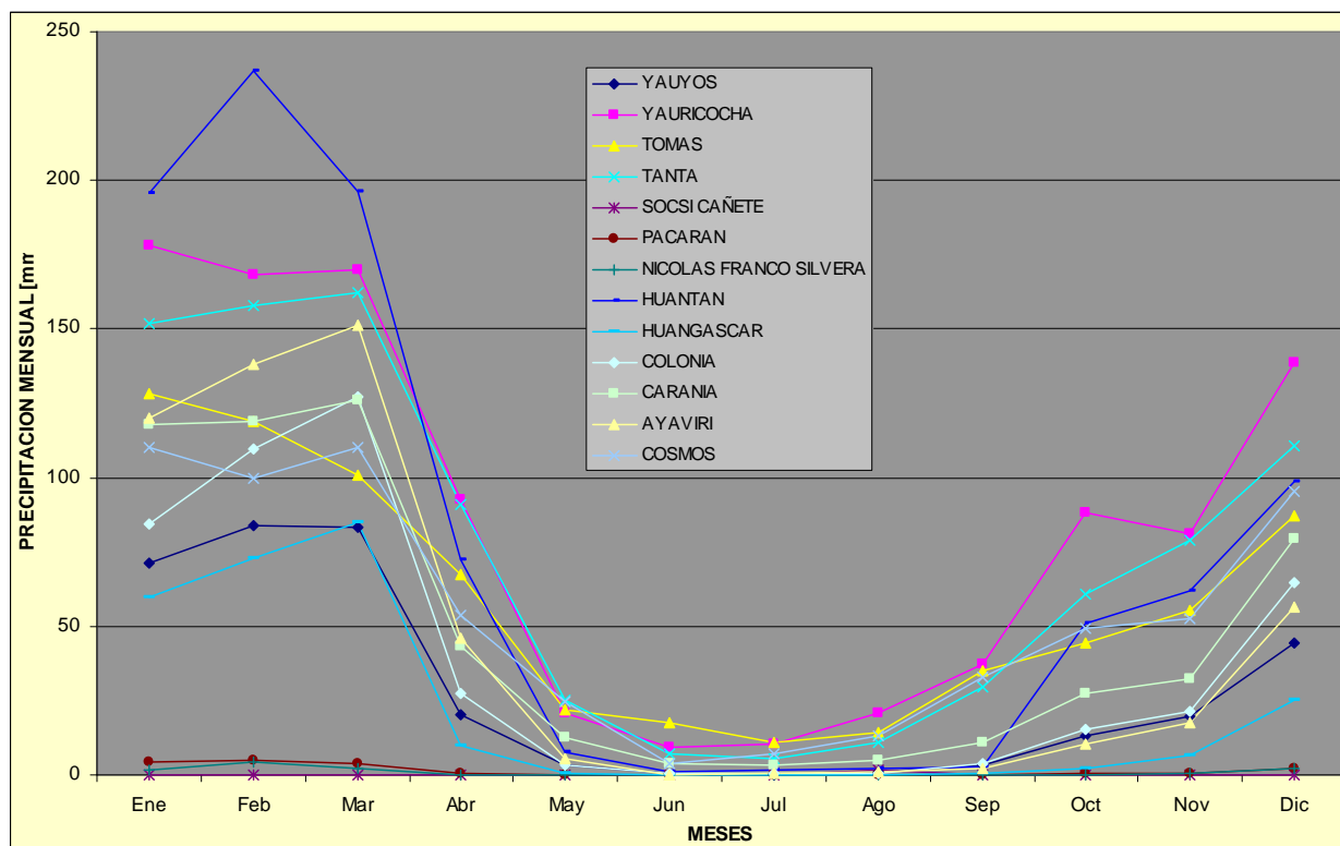
図-3.1.9.1-2 カニエテ川流域およびその近傍の流域における月平均降雨量の分布 (mm)
