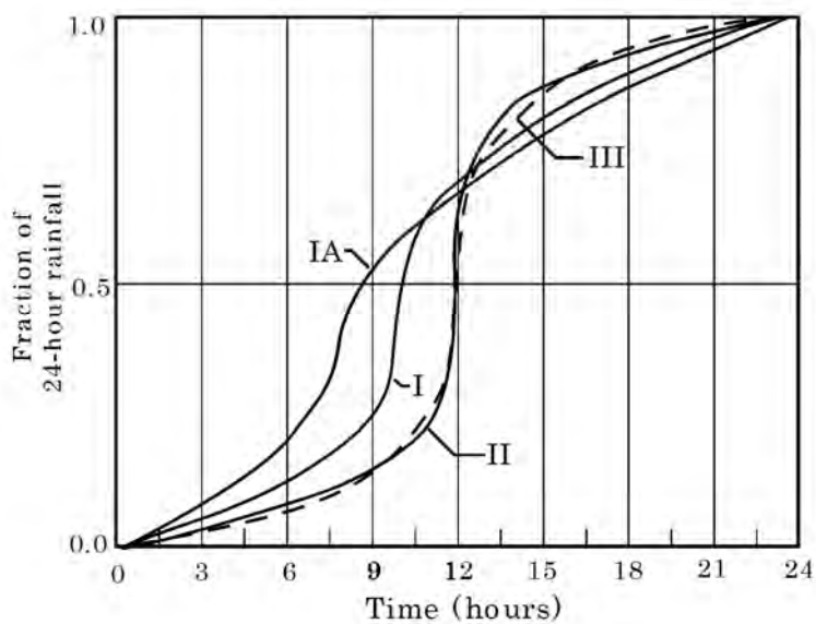
図-3.1.9.4-4 24 時間雨量の降雨量分布
