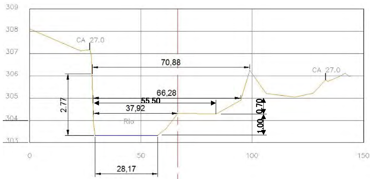
図-3.1.9.5-5 Sosci 流量観測所地点断面図
