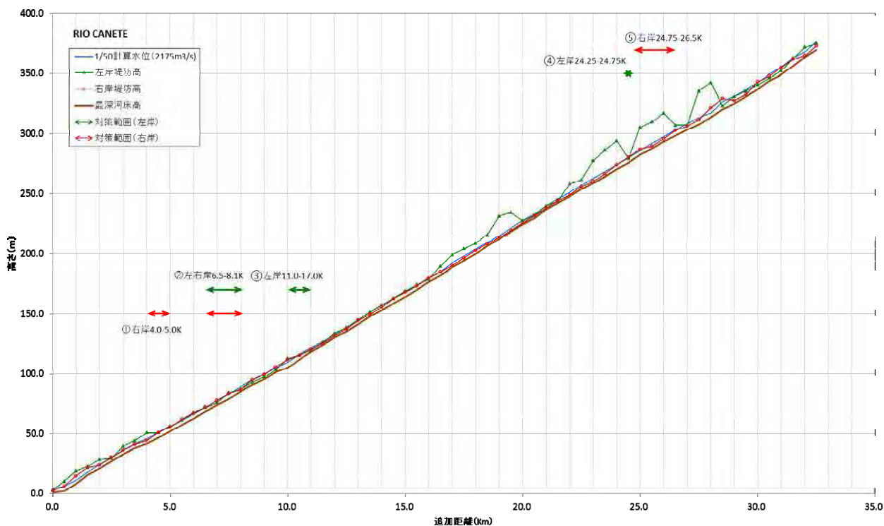
図-4.15.1-3 カニエテ川縦断面図
