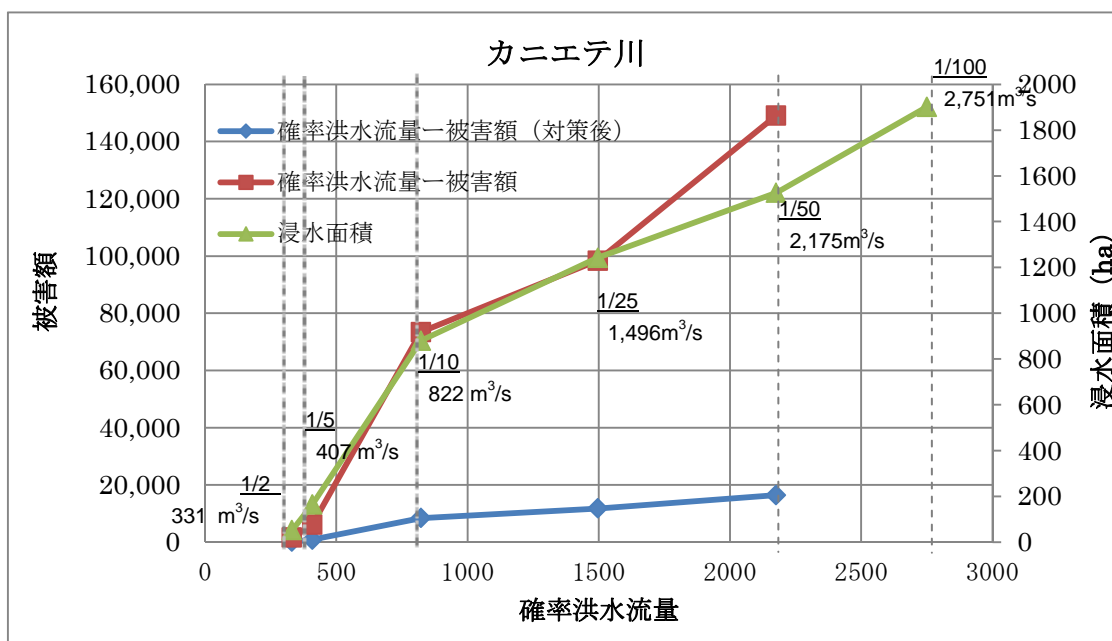
図-4.3.1-2 確率規模洪水流量と被害額および浸水面積 (カニエテ川)
