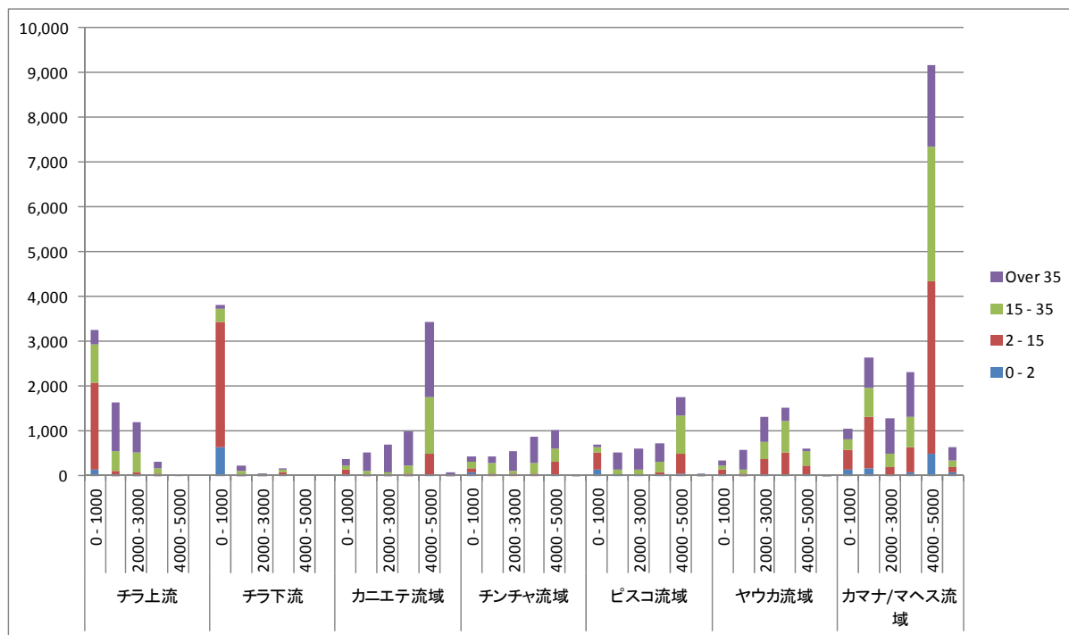
図 3.1.8-12 各流域における斜面勾配と標高の関係
