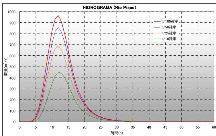
図 3.2.5-4 ピスコ川の洪水ハイドログラフ
