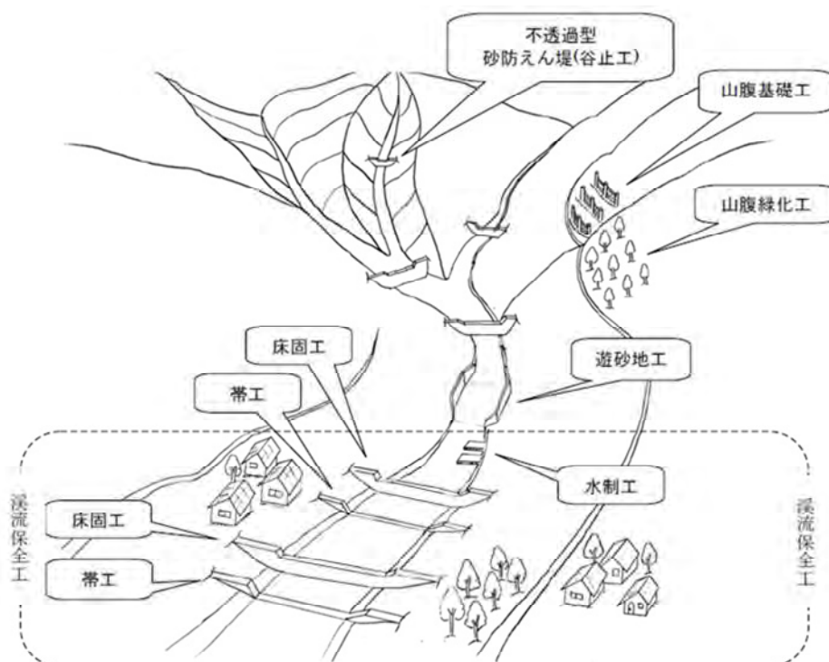
図-4.3.2.2-1 土砂制御対策
