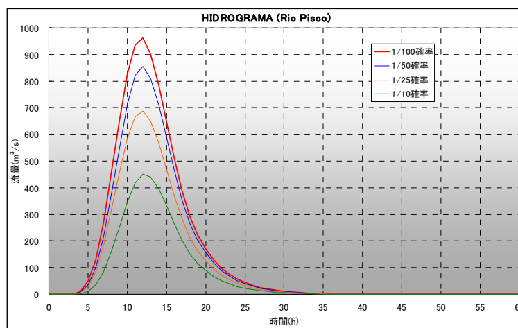
図-3.1.9.4-8 ピスコ川の洪水ハイドログラフ
