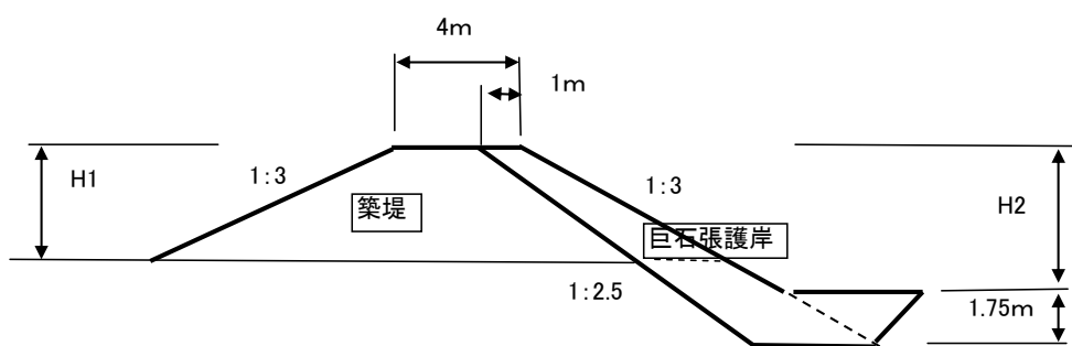
図-4.3.1-5 堤防の標準断面
