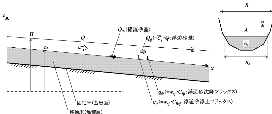
図-4.15.1-5 河床変動解析モデルの概念図
