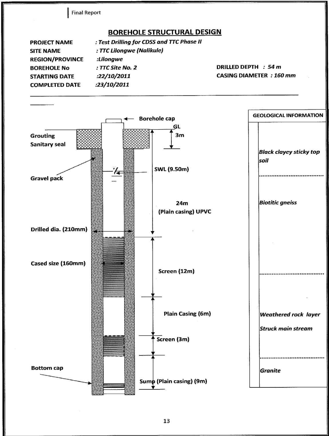
図-3 TTC No. 2 試掘井戸柱状図
