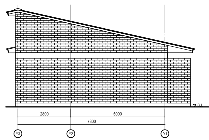
西立面図
