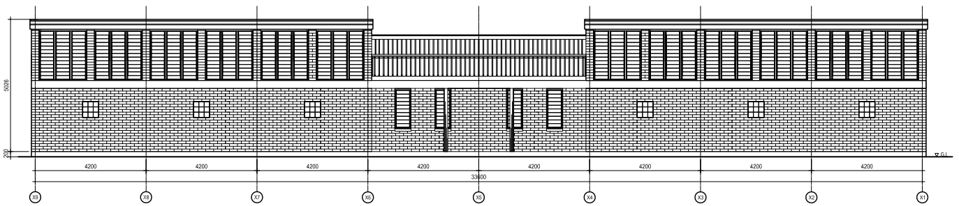
北立面図
