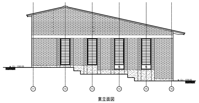
東立面圖
