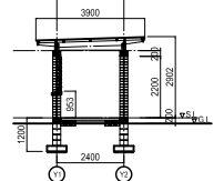
断面图 A-A
