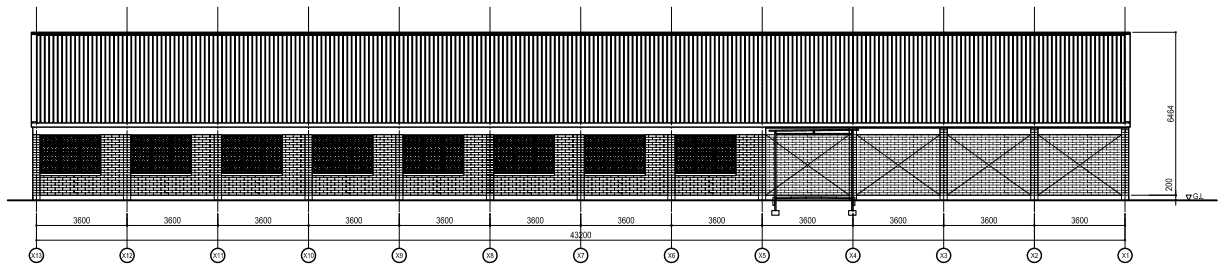
北立面図
