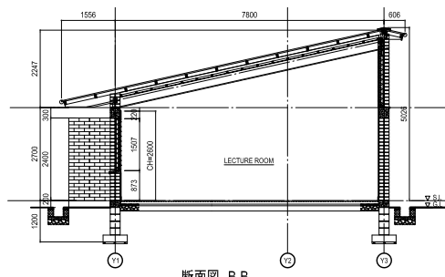
断面図 B-B
