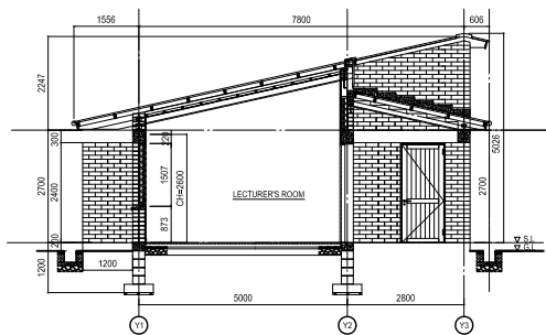
断面図 A-A
