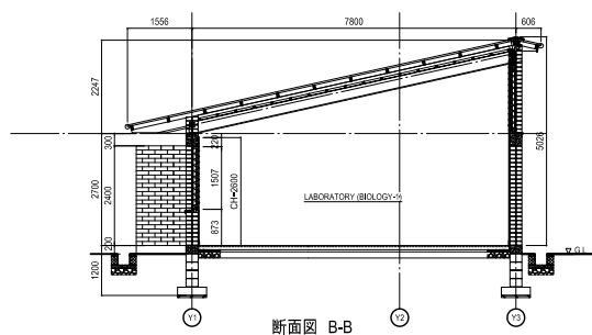
断面図 B-B
