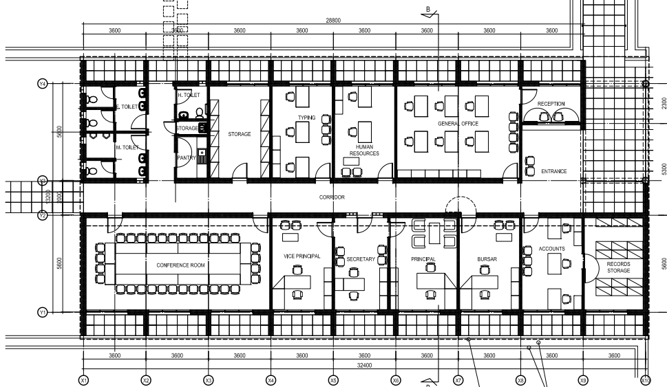
事務管理棟 A 平面圖
