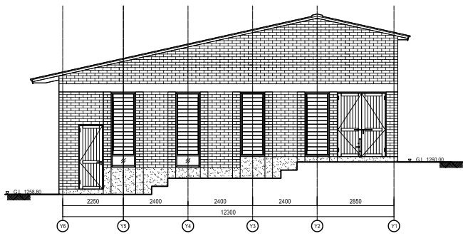
西立面圖
