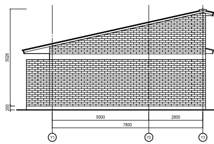
東立面図
