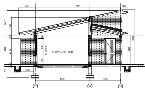
断面図 A-A
