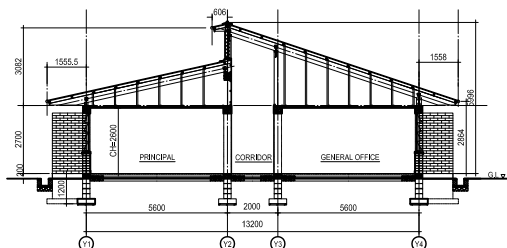
断面圖 B-B 事務管理棟 A
