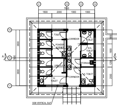
便所 平面图
