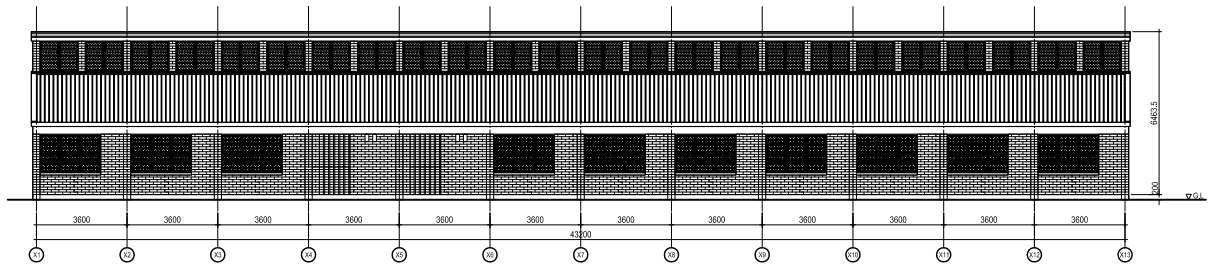
南立面図
