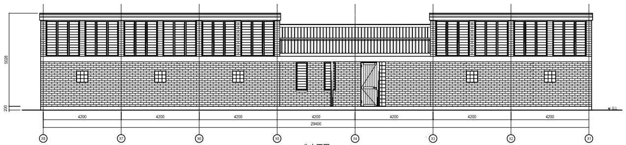
北立面図
