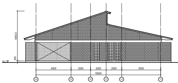
西立面図
