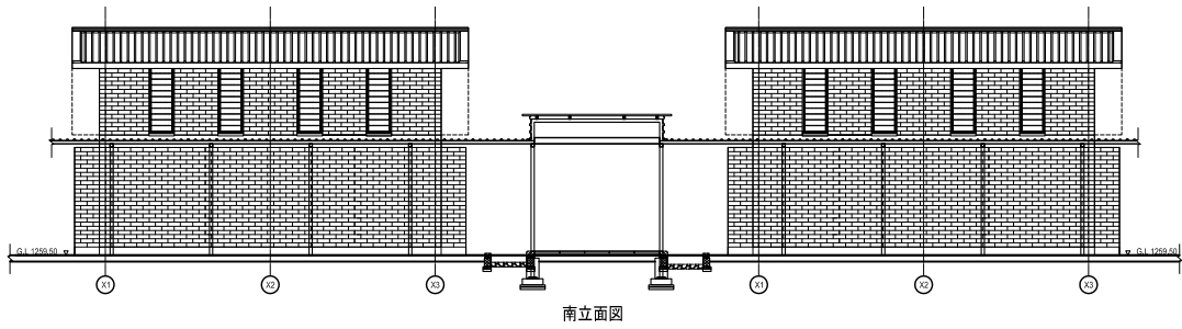
南立面圖
