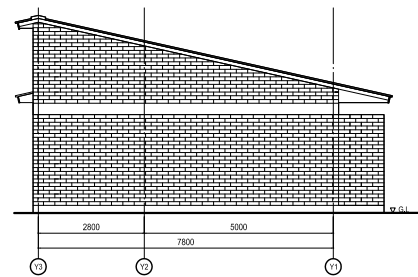
西立面図
