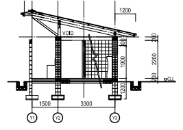
断面图 B-B
