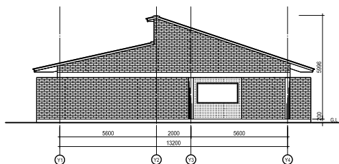
東立面圖 事務管理棟 A
