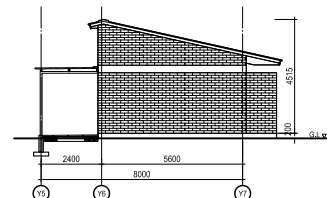
東立面圖 教務管理棟 B
