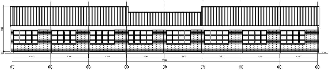
南立面図
