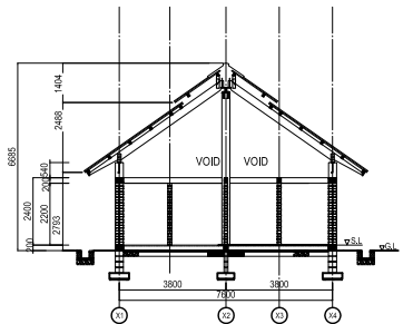
断面图 A-A
