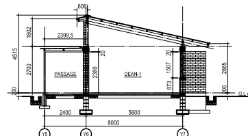
断面圖 A-A 教務管理棟 B
