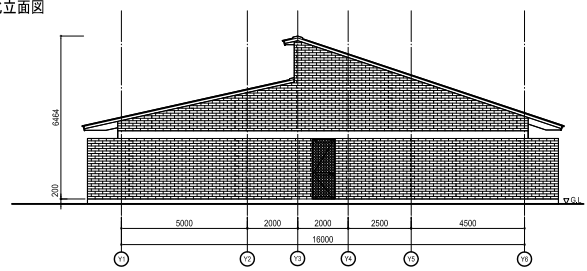
東立面図
