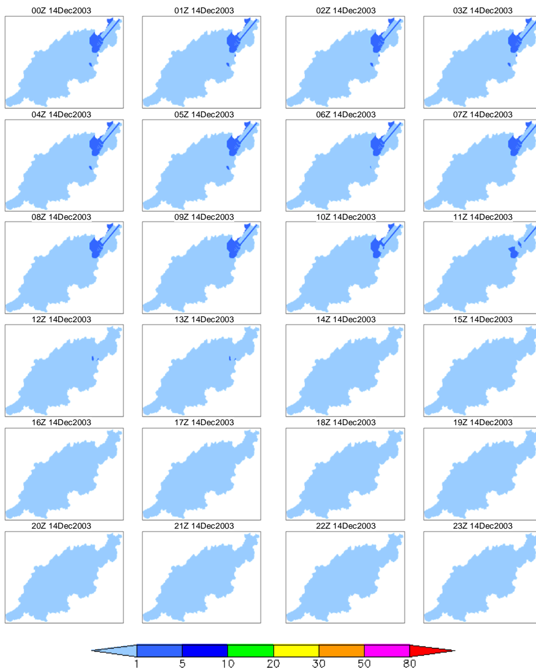
付図 7-e 5日降雨 100年確率降雨の時空間分布 (2003年12月14日(5日目)のケース)
