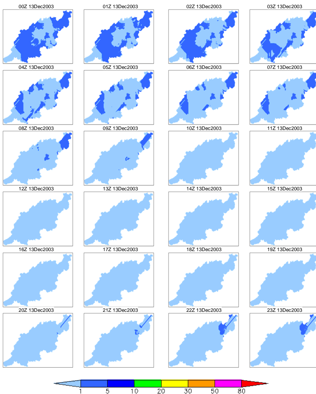
付図 7-d 5日降雨 100年確率降雨の時空間分布 (2003年12月13日(4日目)のケース)
