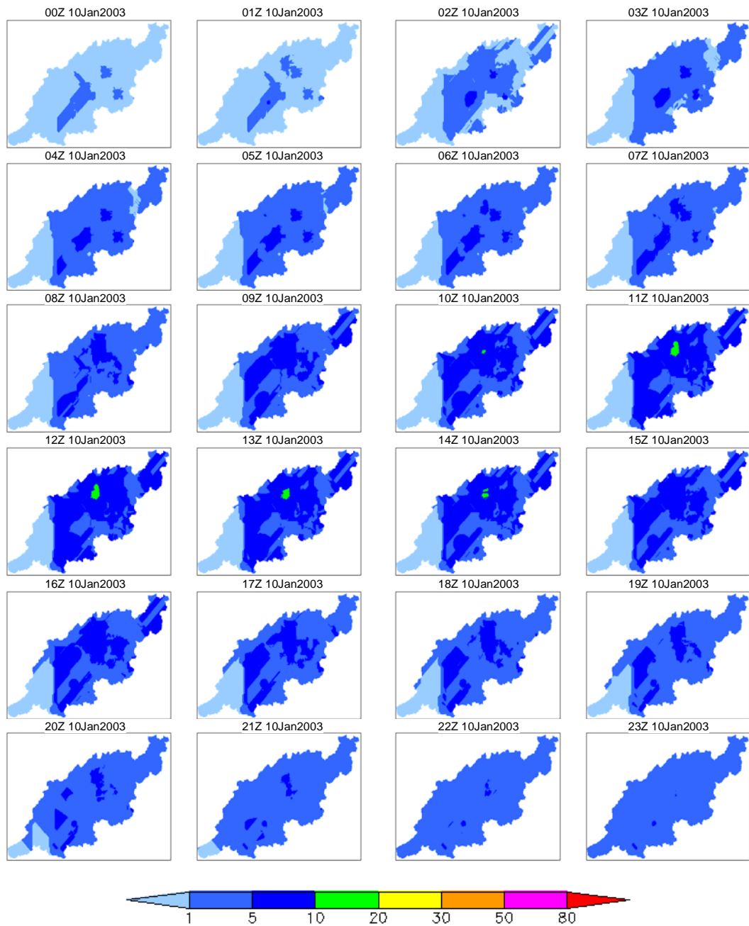
付図 6-c 5日降雨 100年確率降雨の時空間分布 (2003年1月10日(3日目)のケース) 図の時刻表示は、左上が00Zで右に1時間ずつ増加し、右下が23Zを示す。
