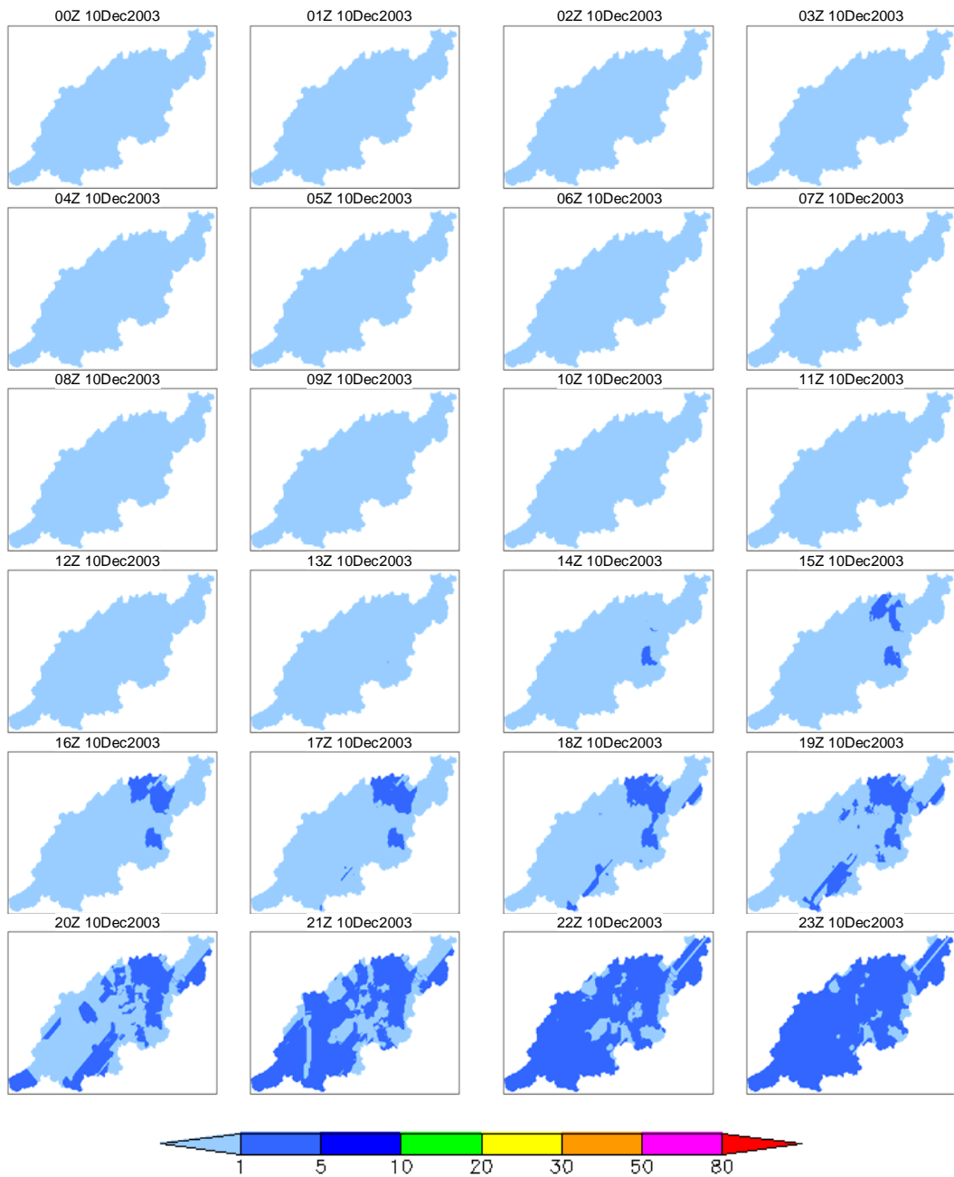
付図 3-a 4日降雨 100年確率降雨の時空間分布 (2003年12月10日(1日目)のケース)
