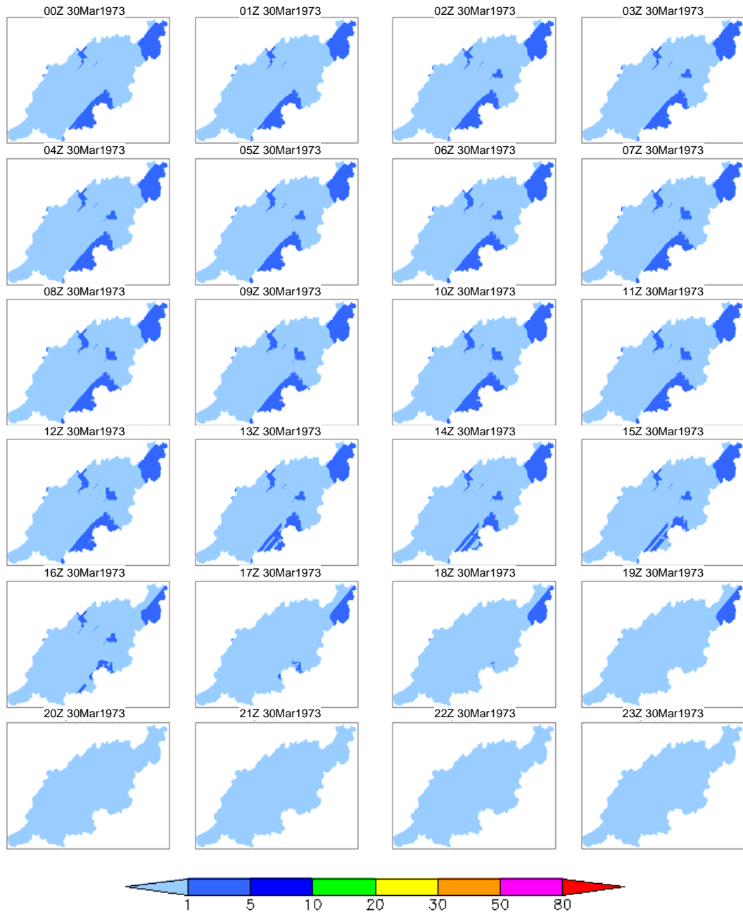
付図 4-e 5日降雨 100年確率降雨の時空間分布 (1973年3月30日(5日目)のケース) 図の時刻表示は、左上が00Zで右に1時間ずつ増加し、右下が23Zを示す。
