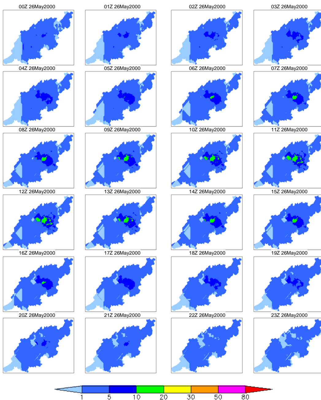
付図 5-d 5日降雨 100年確率降雨の時空間分布（2000年5月26日（4日目）のケース） 図の時刻表示は、左上が00Zで右に1時間ずつ増加し、右下が23Zを示す。
