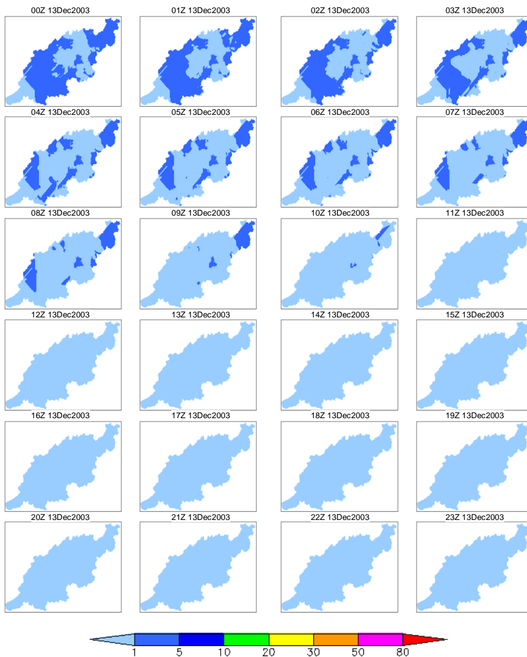
付図 3-d 4日降雨 100年確率降雨の時空間分布 (2003年12月13日(4日目)のケース)
