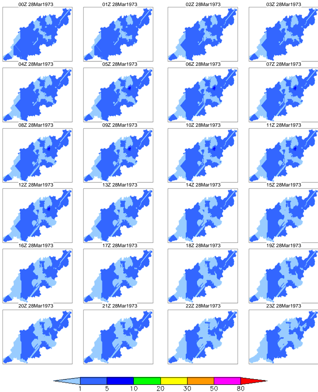
付図 1-c 4日降雨 100年確率降雨の時空間分布 (1973年03月28日(3日目)のケース)
