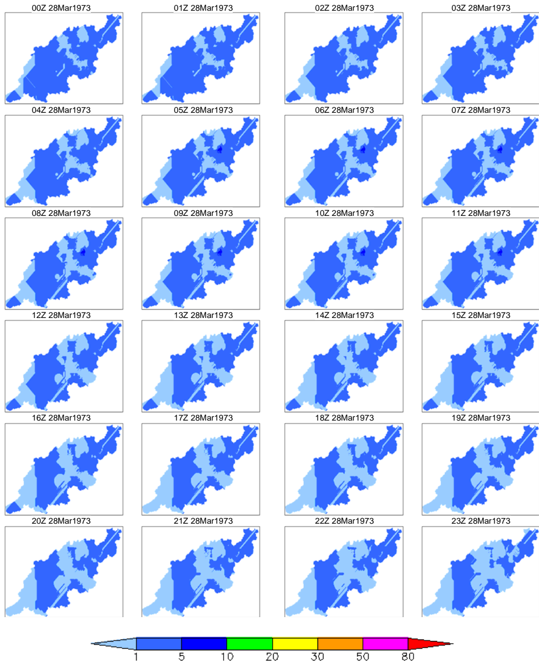
付図 4-c 5日降雨 100年確率降雨の時空間分布（1973年3月28日（3日目）のケース） 図の時刻表示は、左上が00Zで右に1時間ずつ増加し、右下が23Zを示す。
