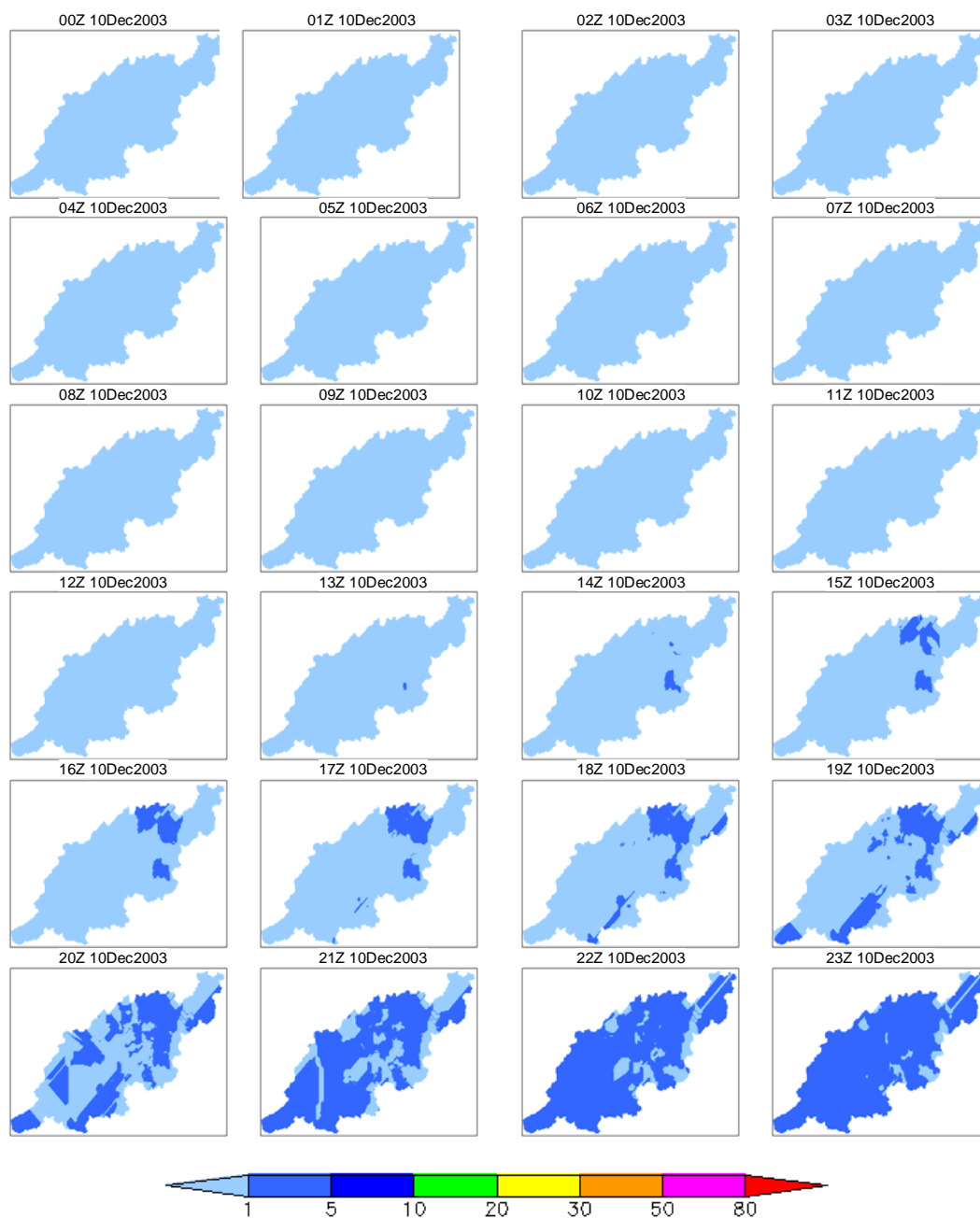
付図 7-a 5日降雨 100年確率降雨の時空間分布 (2003年12月10日(1日目)のケース)
