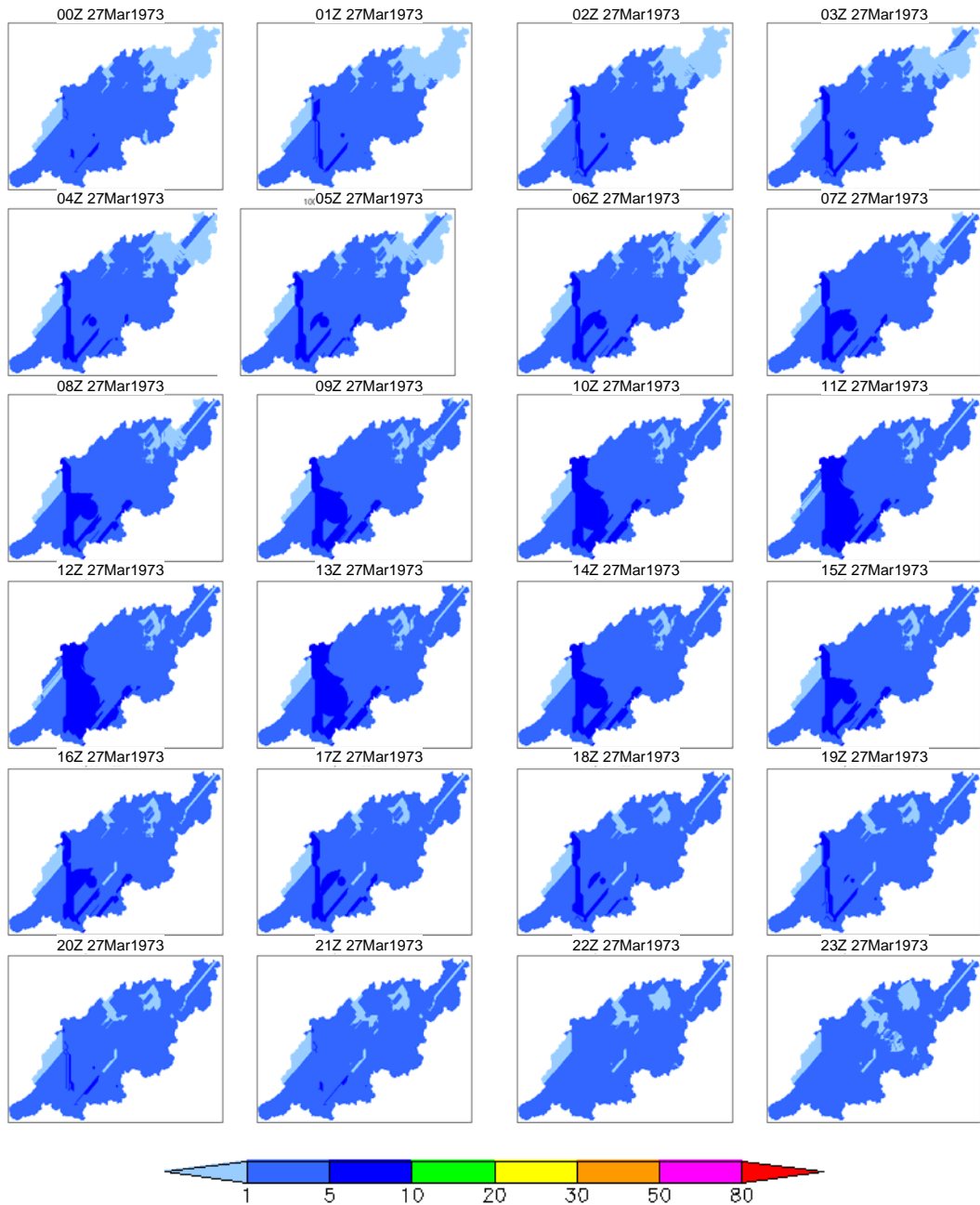
付図 4-b 5日降雨 100年確率降雨の時空間分布（1973年3月27日（2日目）のケース） 図の時刻表示は、左上が00Zで右に1時間ずつ増加し、右下が23Zを示す。
