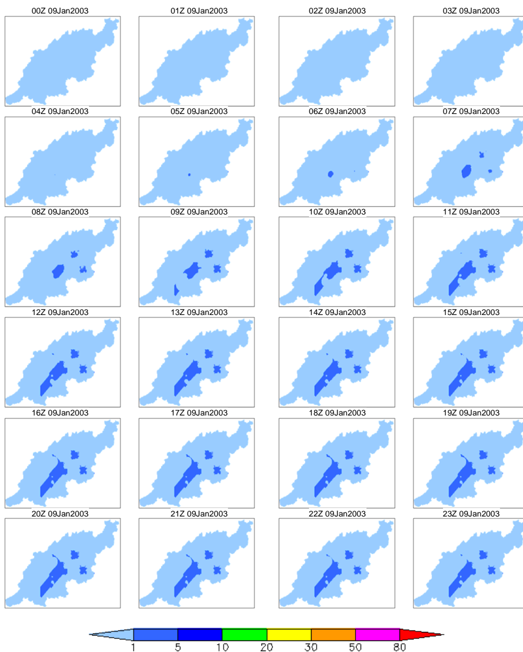
付図 2-a 4日降雨 100年確率降雨の時空間分布 (2003年01月09日(1日目)のケース)
