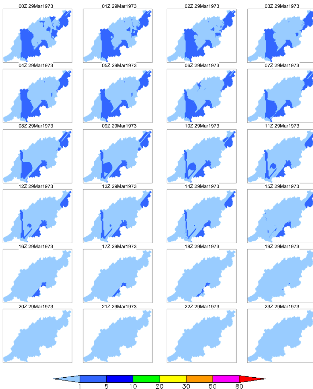
付図 1-d 4日降雨 100年確率降雨の時空間分布 (1973年03月29日(4日目)のケース)
