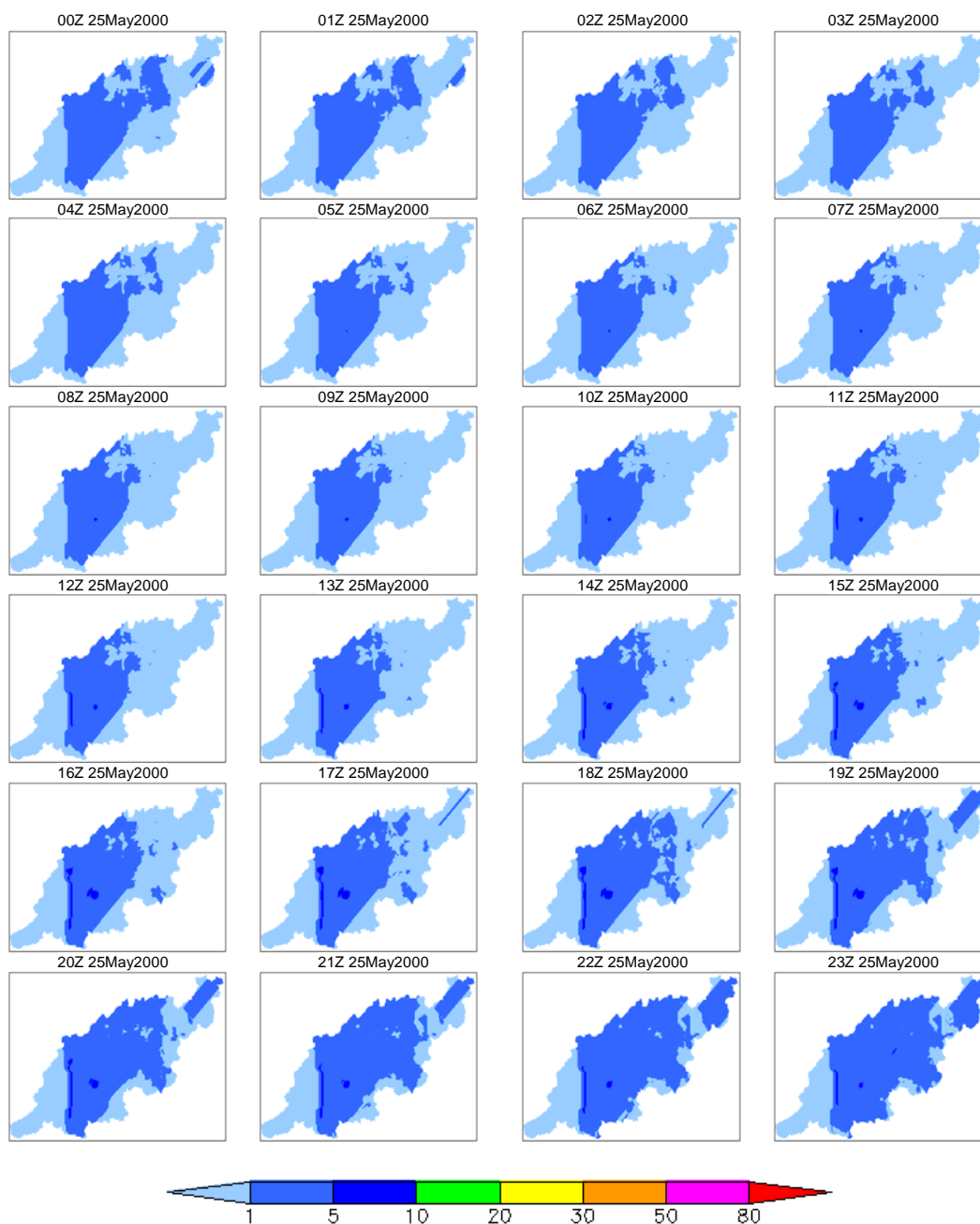
付図 5-c 5日降雨 100年確率降雨の時空間分布（2000年5月25日（3日目）のケース） 図の時刻表示は、左上が00Zで右に1時間ずつ増加し、右下が23Zを示す。
