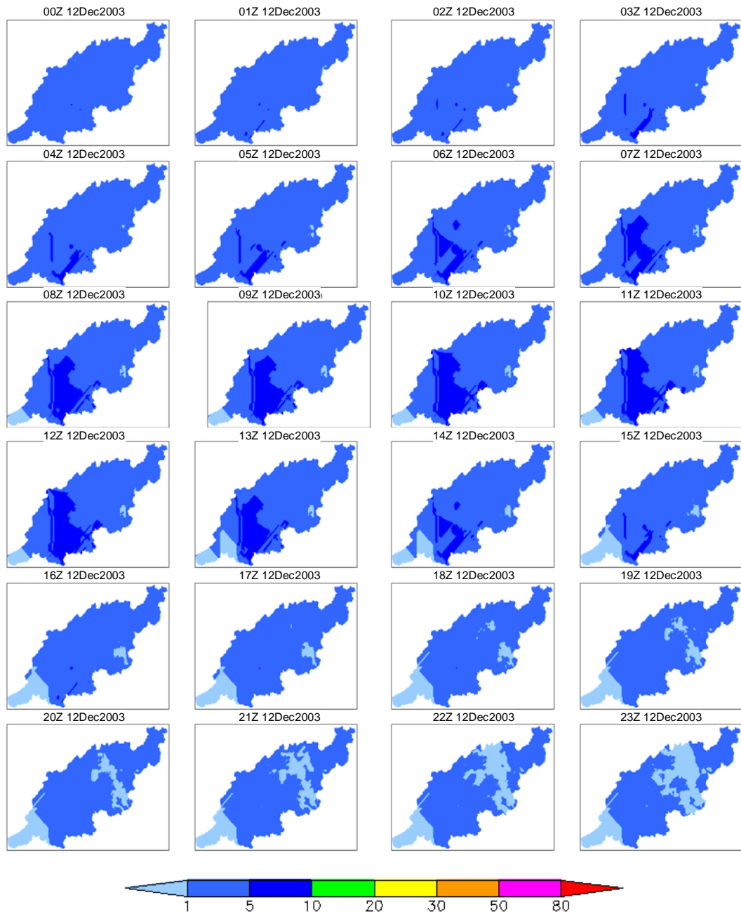
付図 7-c 5日降雨 100年確率降雨の時空間分布 (2003年12月12日(3日目)のケース)
