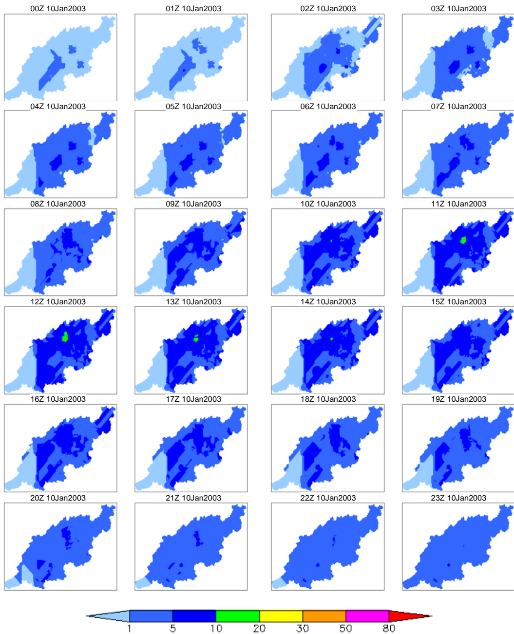
付図 2-b 4日降雨 100年確率降雨の時空間分布 (2003年01月10日(2日目)のケース)
