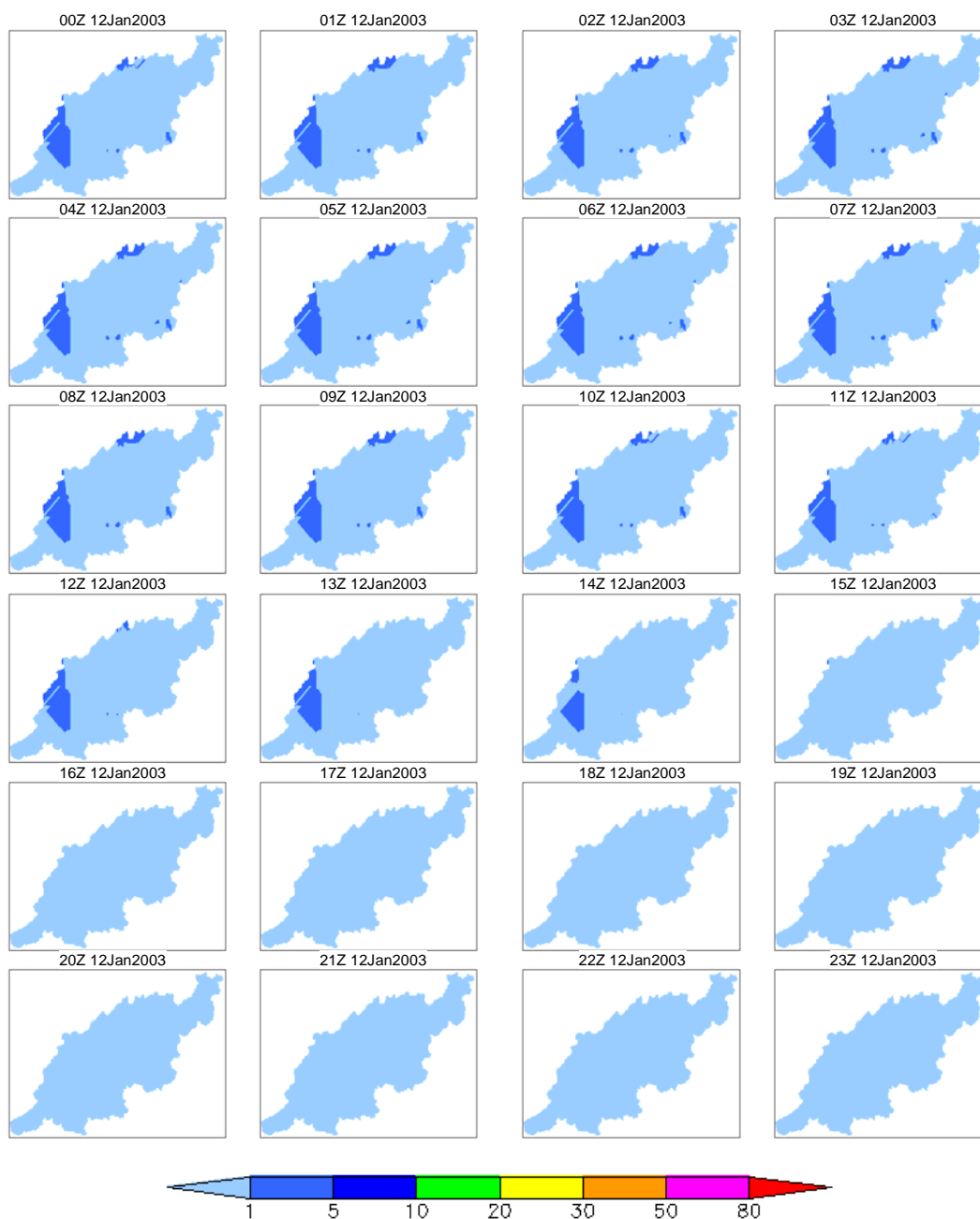
付図 6-e 5日降雨 100年確率降雨の時空間分布 (2003年1月12日(5日目)のケース) 図の時刻表示は、左上が00Zで右に1時間ずつ増加し、右下が23Zを示す。
