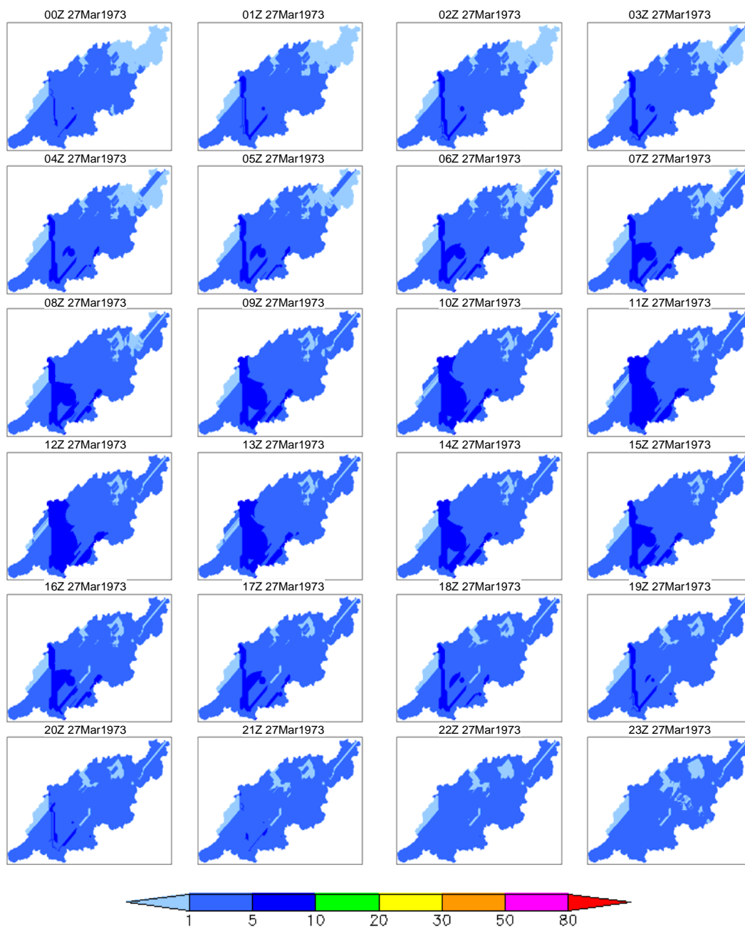
付図 1-b 4日降雨 100年確率降雨の時空間分布 (1973年03月27日(2日目)のケース)
