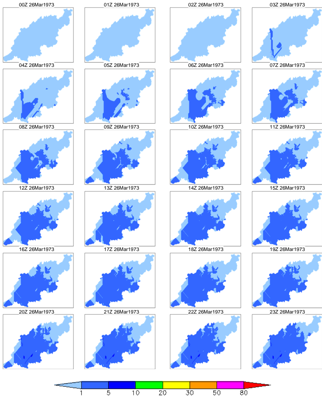
付図 4-a 5日降雨 100年確率降雨の時空間分布（1973年3月26日（1日目）のケース） 図の時刻表示は、左上が00Zで右に1時間ずつ増加し、右下が23Zを示す。
