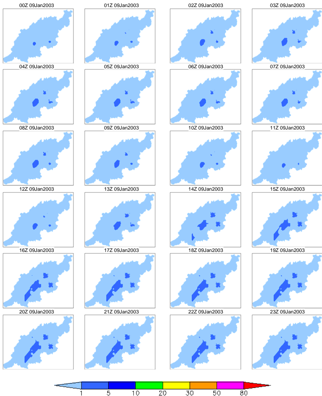
付図 6-b 5日降雨 100年確率降雨の時空間分布（2003年1月9日（2日目）のケース） 図の時刻表示は、左上が00Zで右に1時間ずつ増加し、右下が23Zを示す。
