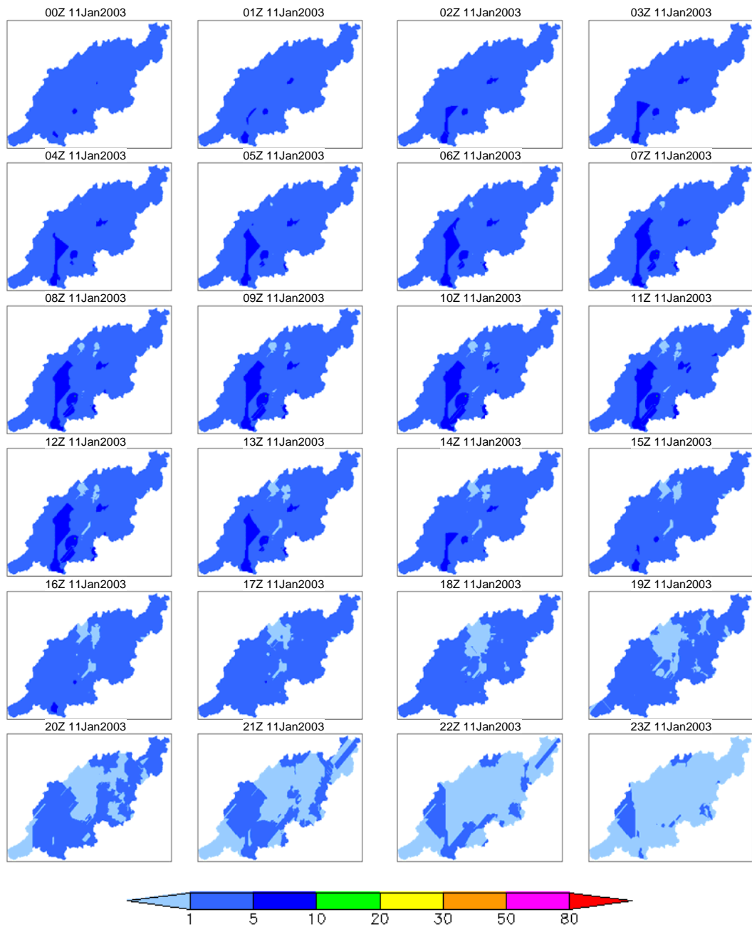
付図 6-d 5日降雨 100年確率降雨の時空間分布(2003年1月11日(4日目)のケース) 図の時刻表示は、左上が00Zで右に1時間ずつ増加し、右下が23Zを示す。
