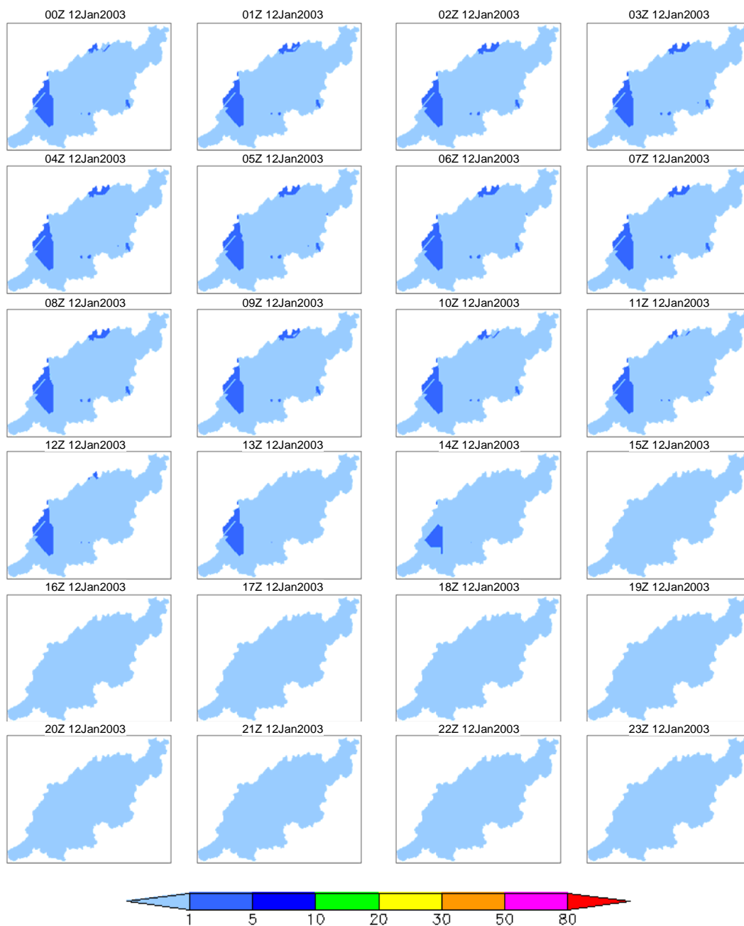
付図 2-d 4日降雨 100年確率降雨の時空間分布 (2003年01月12日(4日目)のケース)
