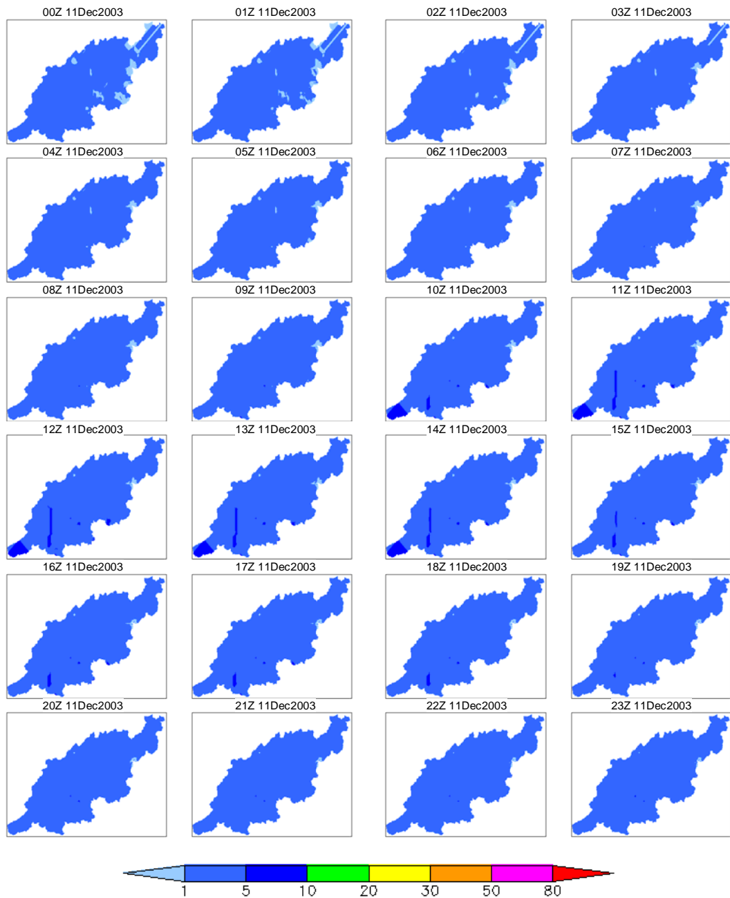
付図 7-b 5日降雨 100年確率降雨の時空間分布 (2003年12月11日(2日目)のケース)
