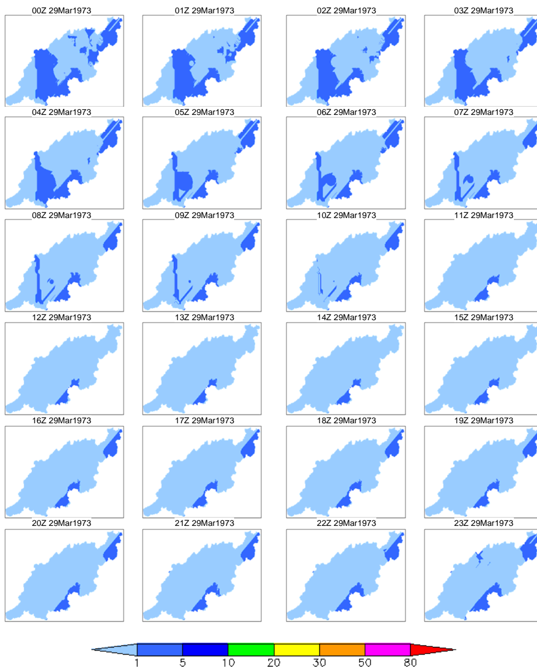
付図 4-d 5日降雨 100年確率降雨の時空間分布（1973年3月29日（4日目）のケース） 図の時刻表示は、左上が00Zで右に1時間ずつ増加し、右下が23Zを示す。
