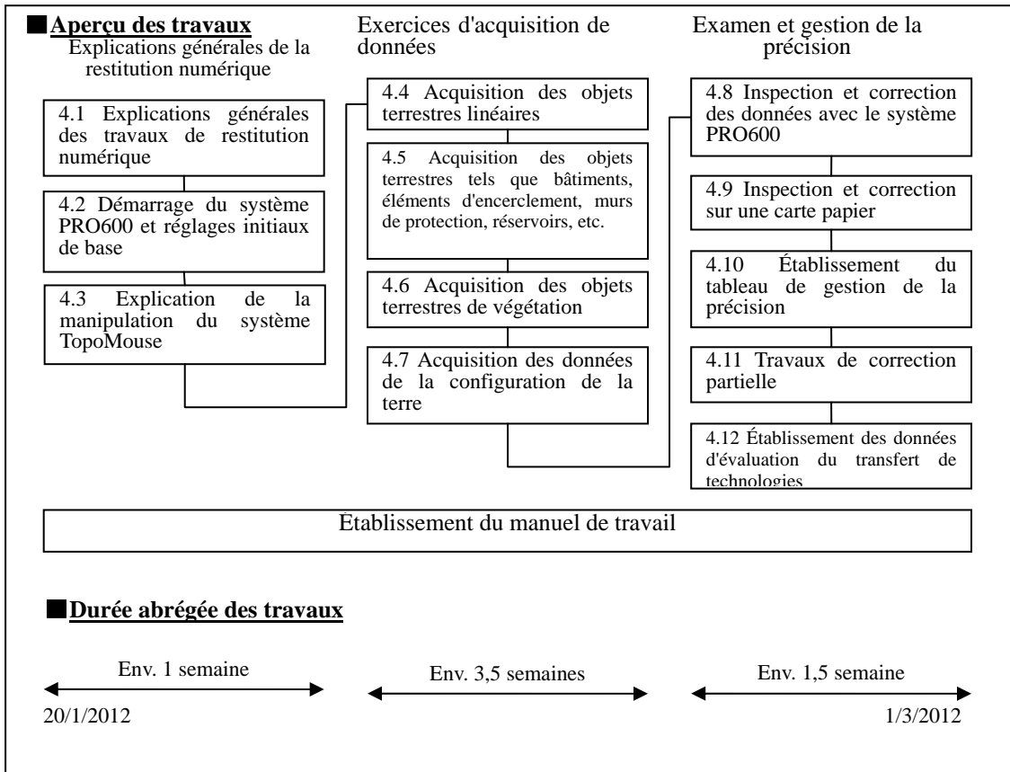
Figure 3-5 Déroutement des travaux de transfert de technologies de la restitution numérique et durée abrégée des travaux
