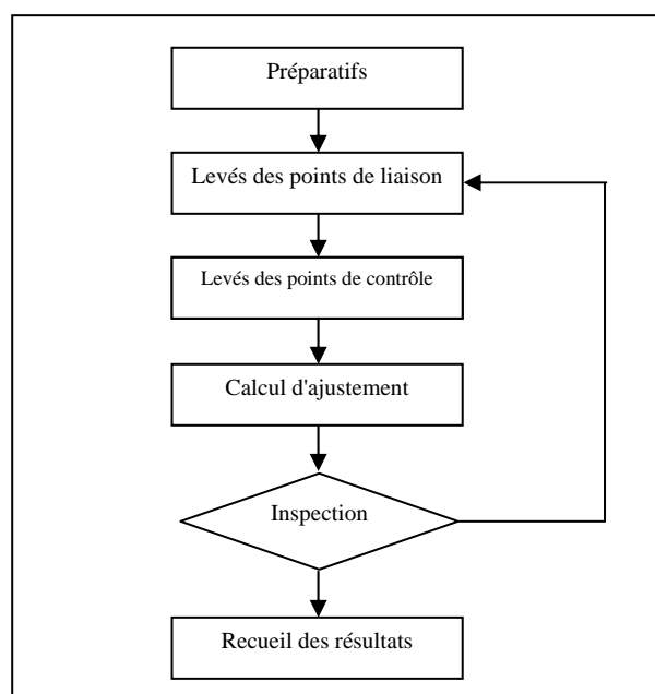
Figure 2-3 Déroulement du transfert de technologies portant sur l'aérotriangulation
