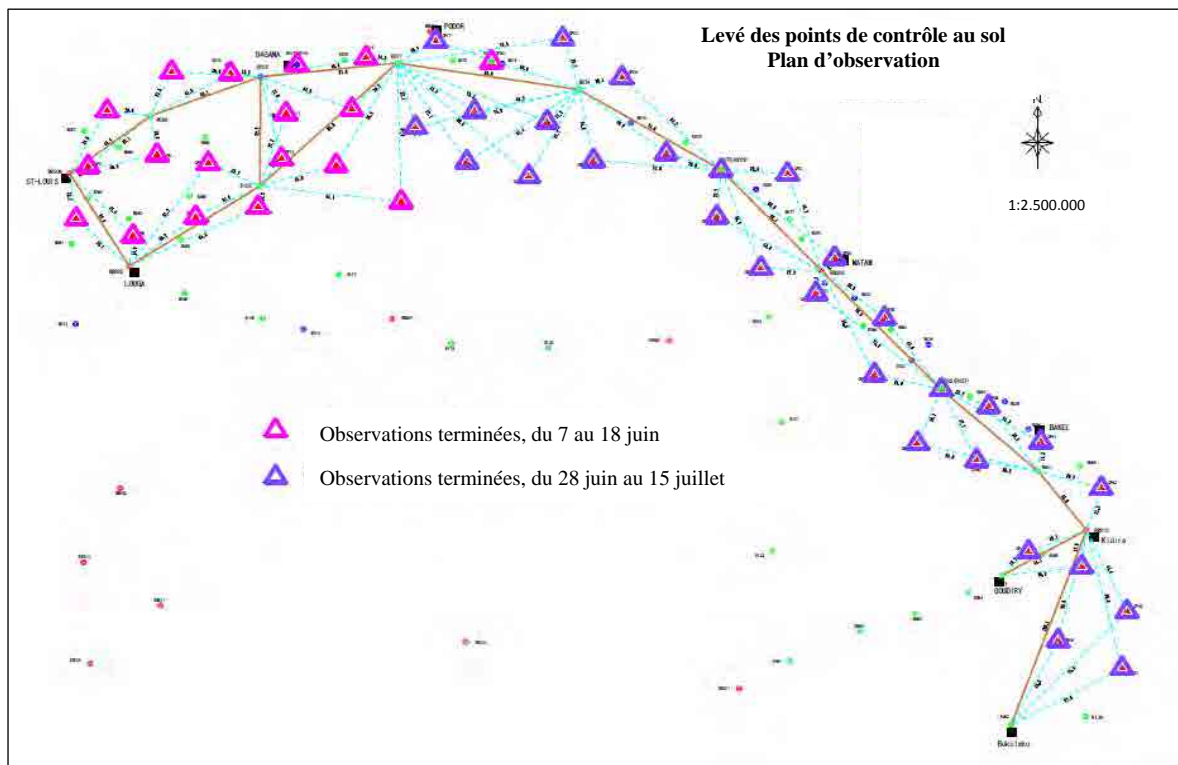
Figure 2-1 Réseau des observations GNSS
