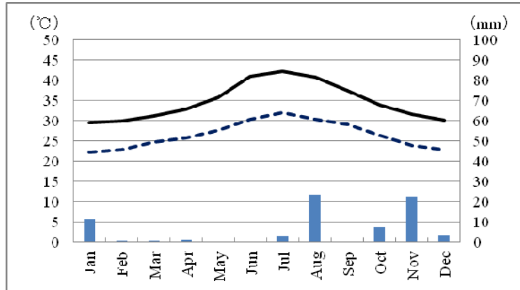
図 2-10 ジブチ市の気温と降水量 (5ヶ年年均 2006-2010)
