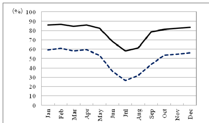
図 2-11 ジブチ市の湿度 (5ヶ年年均 2006-2010)
