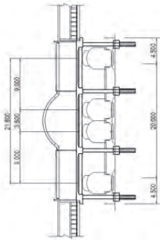
B - B
