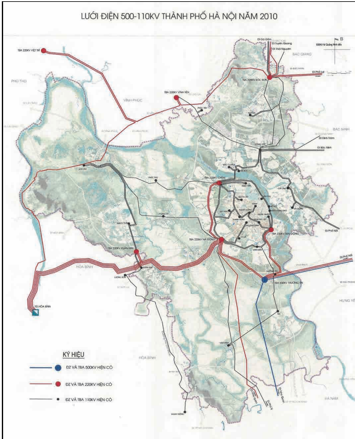
図 3. 6. 1 ハノイ市 500-110 KV 電力系統図 (2010 年時点)
