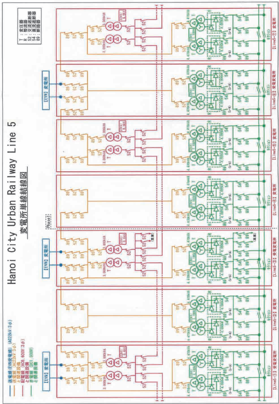
圖 3.6.4 5 号線變電所單線結線圖
