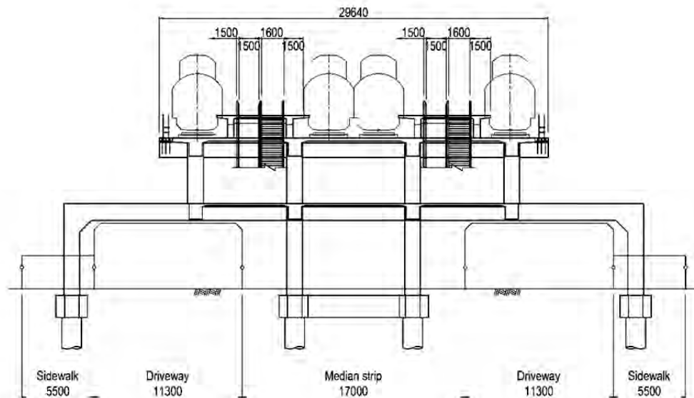
図3.10.18 高架駅（2面4線）
