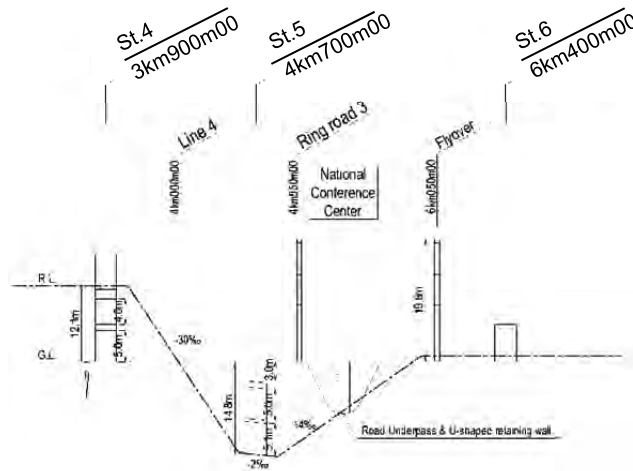
図 3.10.4 St. 5 付近④案詳細図
