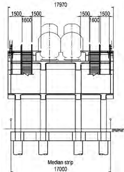
図3.10.17 高架駅（相対式2面2線）
