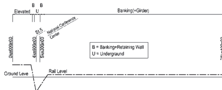
出典：調査団作成 図 3.10.3 高架—地下—地上案
